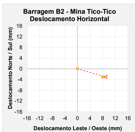
Figura 6.93 – Marco de controle de deformação – MS-09.
