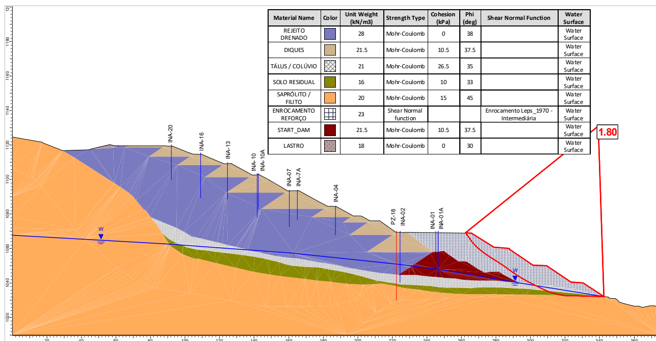
Figura 6.108 – Seção B-B' – Análise Drenada – Superfície de ruptura plano-circular otimizada – Freática 30/04/2025.
