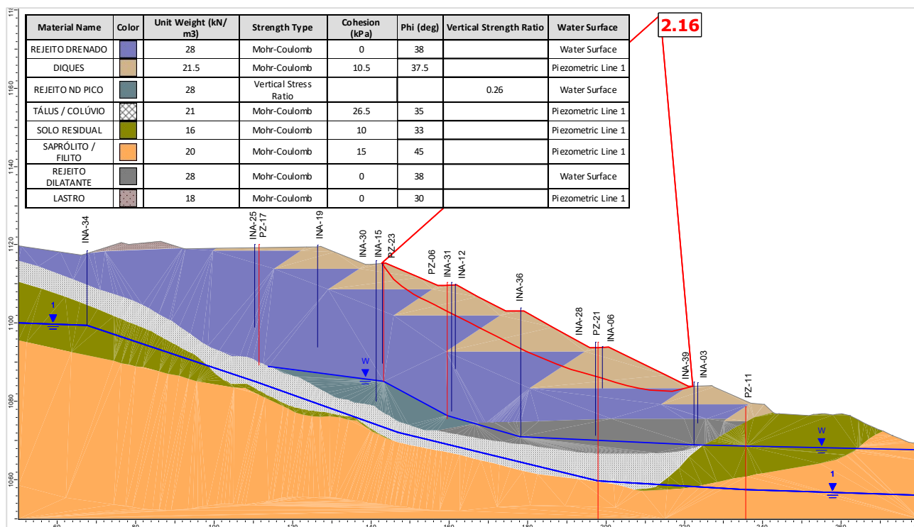
Figura 6.102 – Seção A-A' – Análise Não Drenada – Superfície de ruptura plano-circular otimizada – Freática 30/04/2025 – Razão de resistência não drenada de pico.
