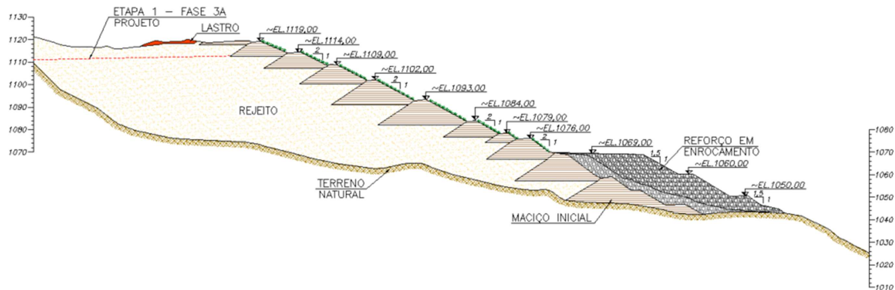
Figura 6.12 – Comparativo Projeto (Etapa 1 - Fase 3A) x Executado – Seção E-E'.
