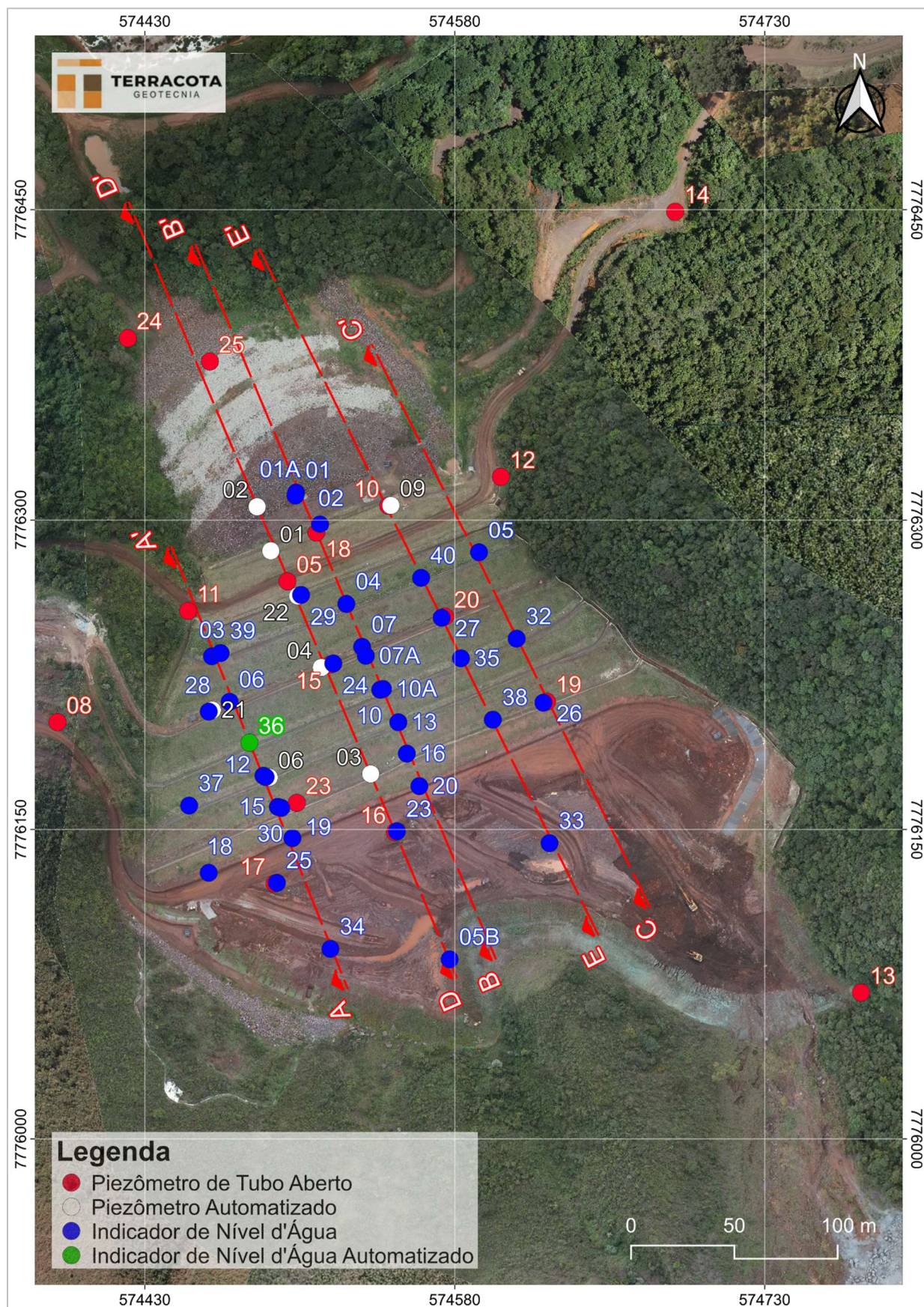
Figura 6.98 – Seções Instrumentadas Barragem B2 – Mina Tico-Tico – Planta.
