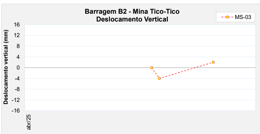
Figura 6.87 – Marco de controle de deformação – MS-03.
