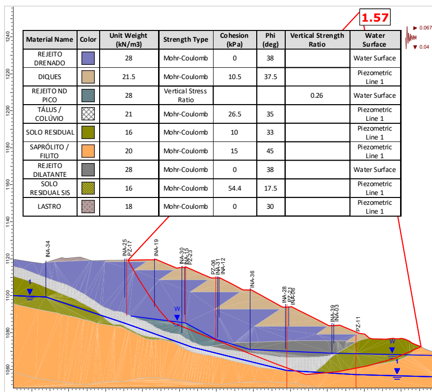
Figura 6.107 – Seção A-A' – Análise Não Drenada – Superfície de ruptura plano-circular otimizada – Freática 30/04/2025 – Razão de resistência não drenada de pico + sismo ↓ (critério vida útil).
