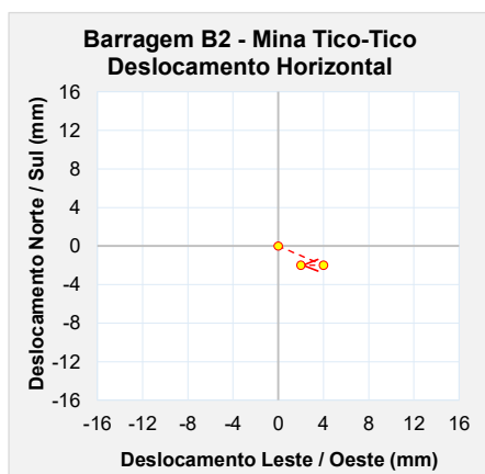
Figura 6.95 – Marco de controle de deformação – MS-11.
