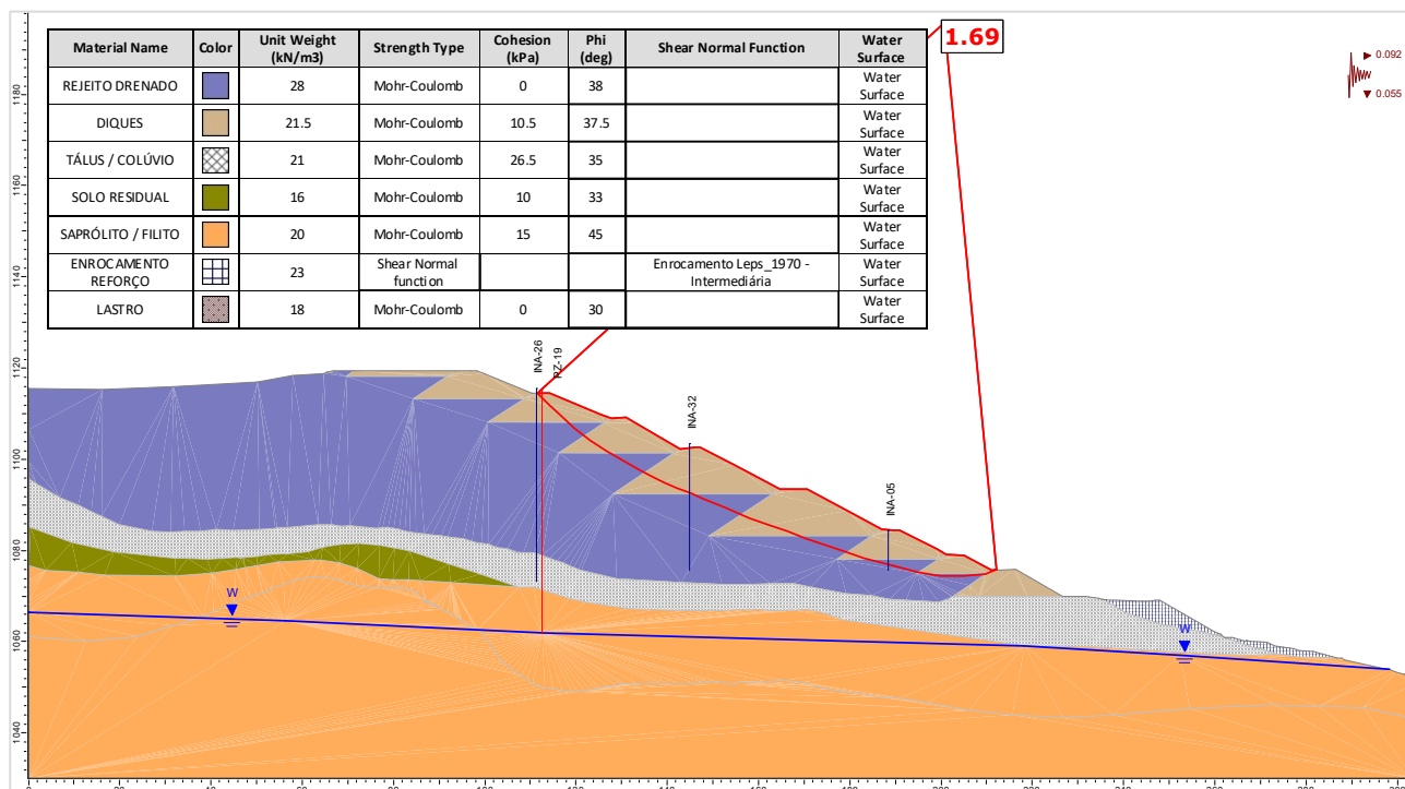
Figura 6.117 – Seção C-C' – Análise Drenada – Superfície de ruptura plano-circular otimizada – Freática 30/04/2025 – Carregamento sísmico ↓ (critério CDA).
