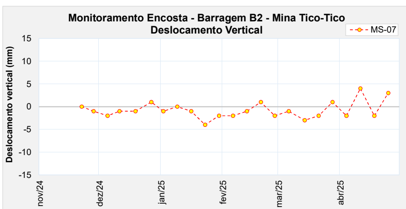
Figura 5.17 – Marco de controle de monitoramento da encosta – MS-07.
