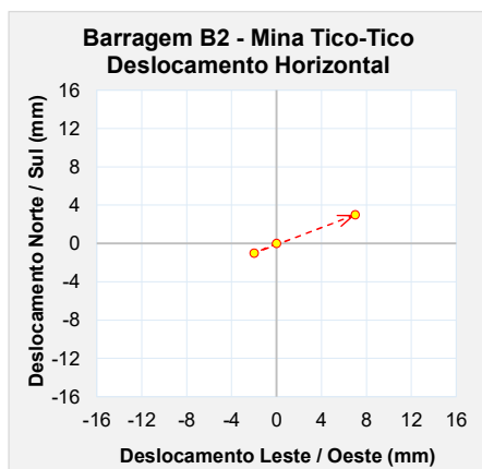
Figura 6.94 – Marco de controle de deformação – MS-10.
