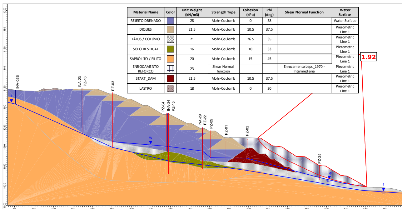
Figura 6.120 – Seção D-D' – Análise Drenada – Superfície de ruptura plano-circular otimizada – Freática 30/04/2025.
