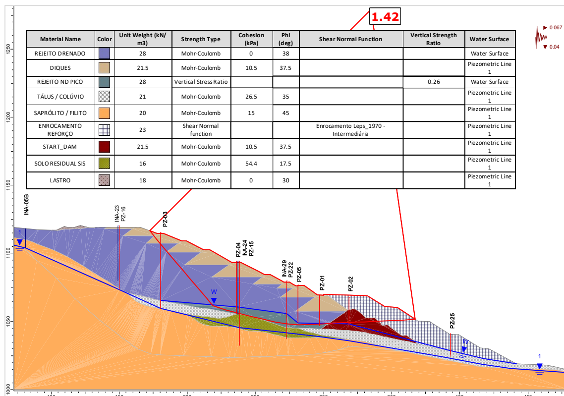
Figura 6.126 – Seção D-D' – Análise Não Drenada – Superfície de ruptura plano-circular otimizada – Freática 30/04/2025 – Razão de resistência não drenada de pico + sismo ↓ (critério vida útil).
