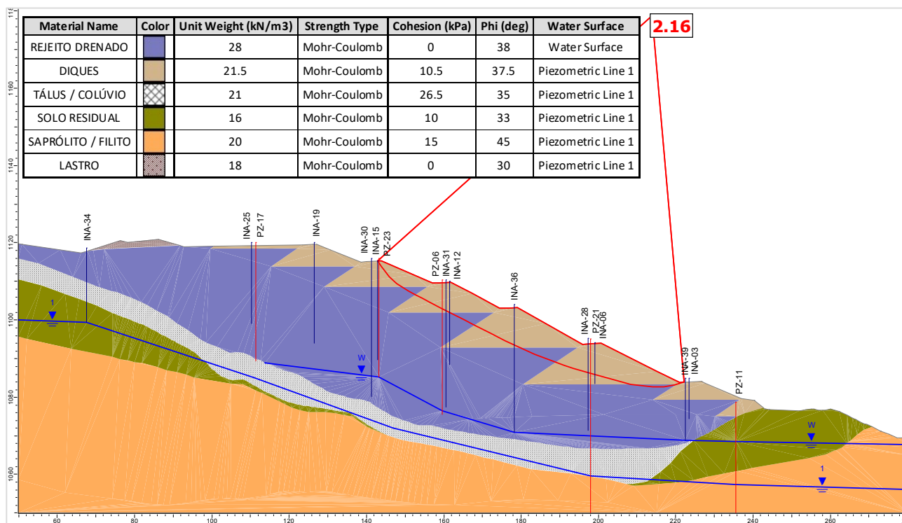
Figura 6.101 – Seção A-A' – Análise Drenada – Superfície de ruptura plano-circular otimizada – Freática 30/04/2025.
