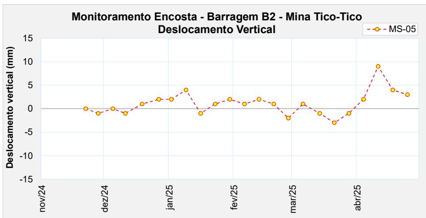
Figura 5.15 – Marco de controle de monitoramento da encosta – MS-05.
