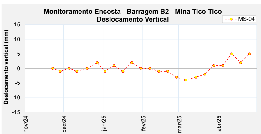
Figura 5.14 – Marco de controle de monitoramento da encosta – MS-04.
