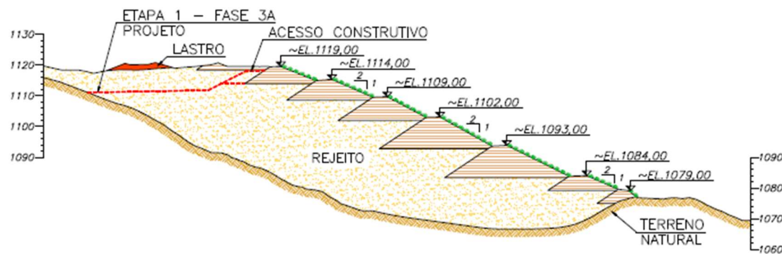
Figura 6.8 – Comparativo Projeto (Etapa 1 - Fase 3A) x Executado – Seção A-A'.
