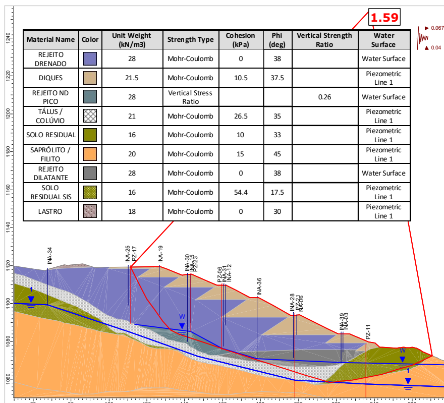
Figura 6.106 – Seção A-A' – Análise Não Drenada – Superfície de ruptura plano-circular otimizada – Freática 30/04/2025 – Razão de resistência não drenada de pico + sismo ↑ (critério vida útil).
