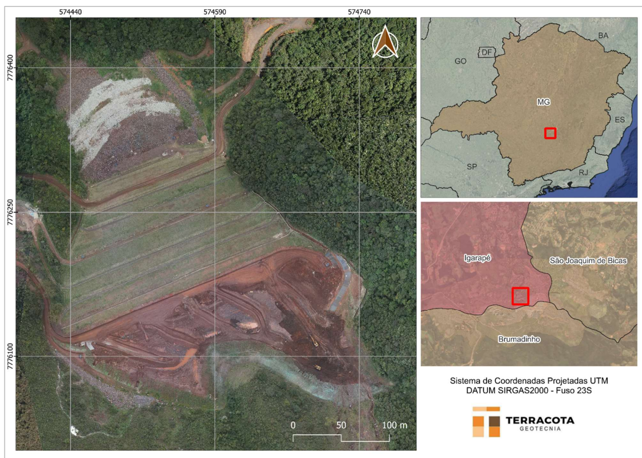
Figura 4.1 – Localização da Barragem B2 – Mina Tico-Tico.
