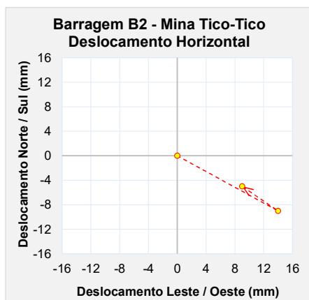
Figura 6.91 – Marco de controle de deformação – MS-07.
