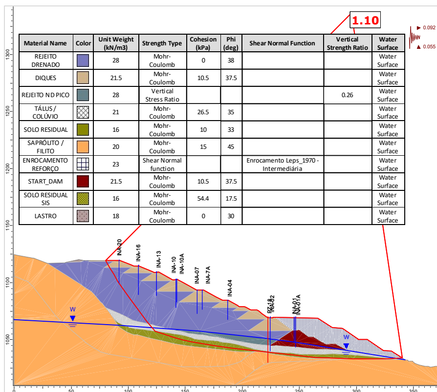
Figura 6.111 – Seção B-B' – Análise Não Drenada – Superfície de ruptura plano-circular otimizada – Freática 30/04/2025 – Razão de resistência não drenada de pico + sismo ↑ (critério CDA).
