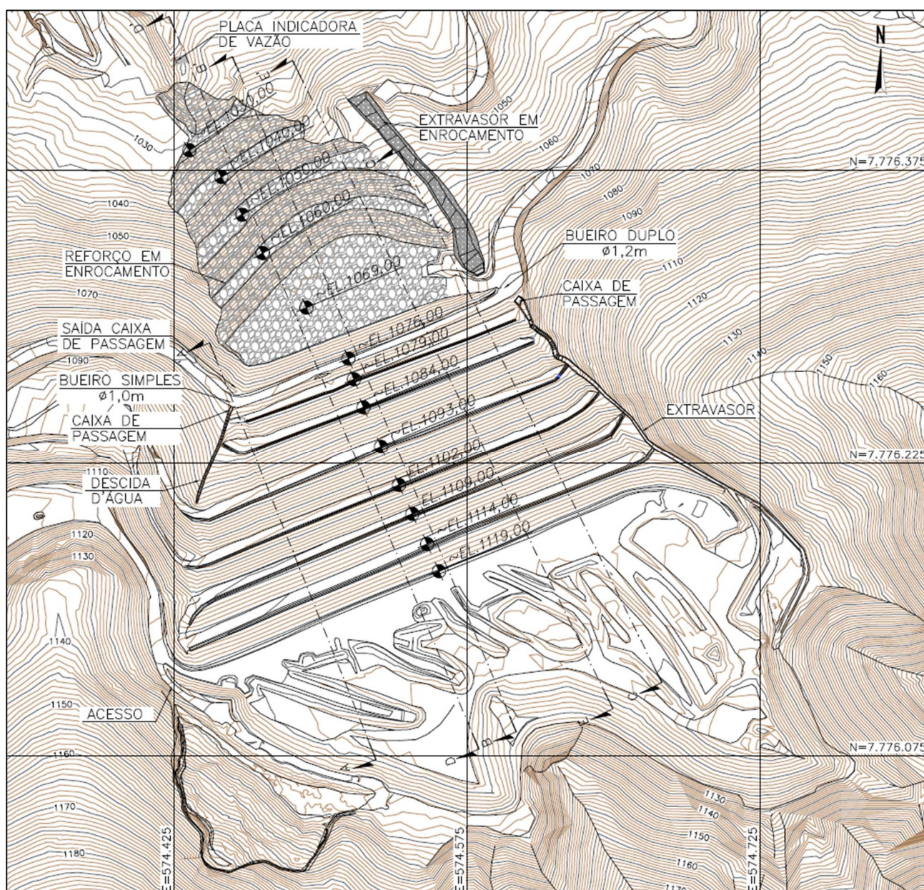
Figura 6.4 – Levantamento topográfico 01/05/2025 – Obras Executadas - Planta.
