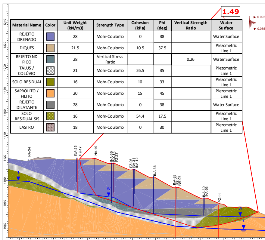
Figura 6.105 – Seção A-A' – Análise Não Drenada – Superfície de ruptura plano-circular otimizada – Freática 30/04/2025 – Razão de resistência não drenada de pico + sismo ↓ (critério CDA).
