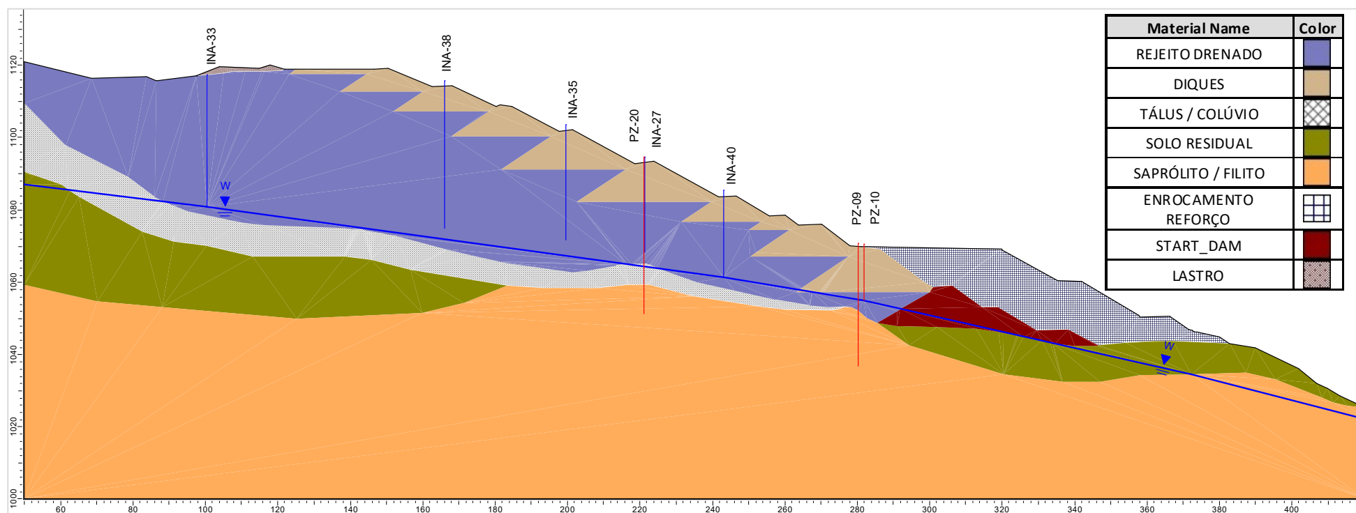
Figura 6.21 – Seção transversal de controle E-E' (Condição em 01/05/2025).
