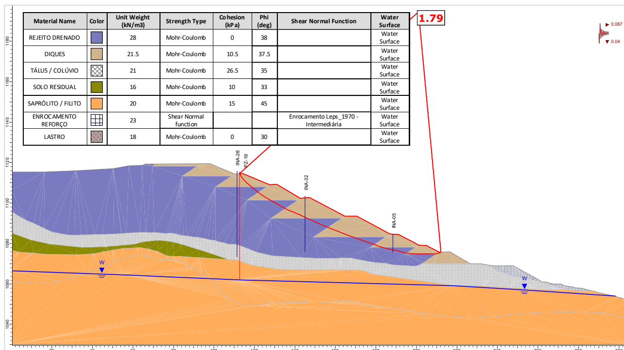
Figura 6.119 – Seção C-C' – Análise Drenada – Superfície de ruptura plano-circular otimizada – Freática 30/04/2025 – Carregamento sísmico ↓ (critério vida útil).
