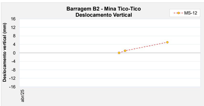
Figura 6.96 – Marco de controle de deformação – MS-12.
