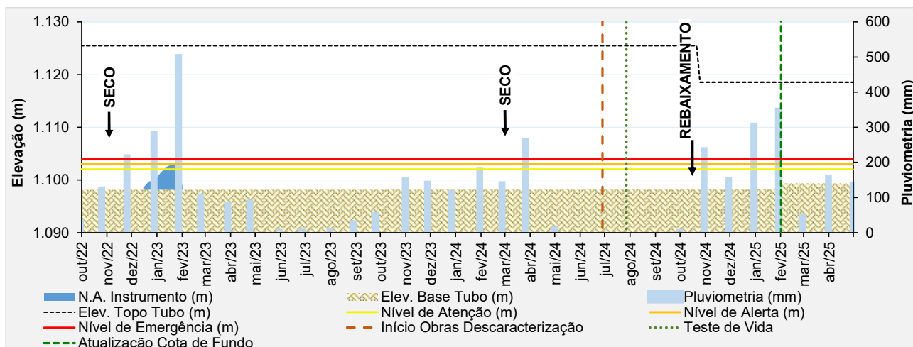
Figura 6.52 – Desempenho do indicador de nível d'água – INA-34.
