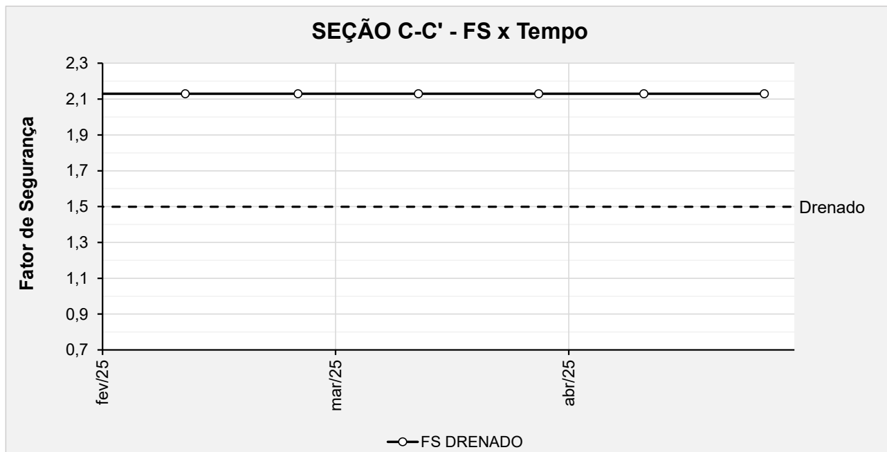
Figura 6.136 – Seção C-C' - Histórico dos F.S. obtidos nas análises de estabilidade no período avaliado.
