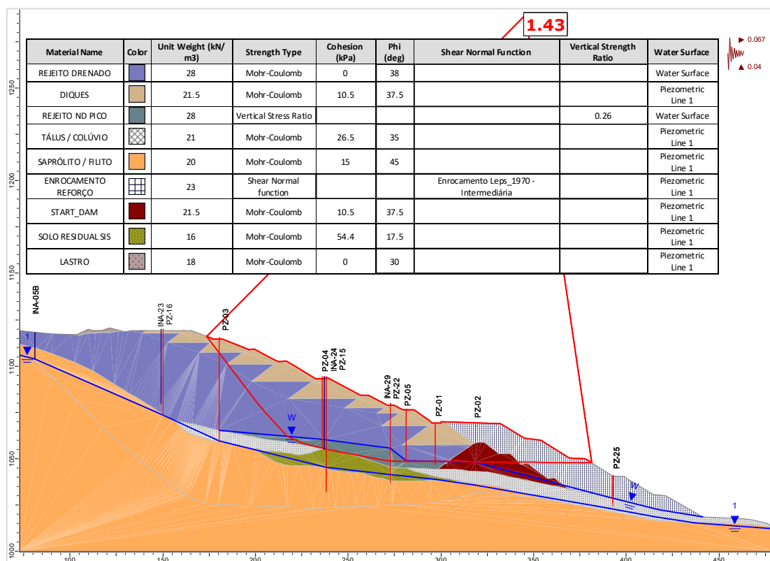
Figura 6.125 – Seção D-D' – Análise Não Drenada – Superfície de ruptura plano-circular otimizada – Freática 30/04/2025 – Razão de resistência não drenada de pico + sismo ↑ (critério vida útil).
