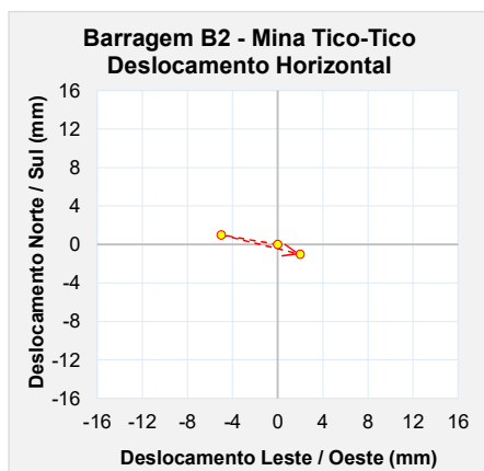
Figura 6.88 – Marco de controle de deformação – MS-04.
