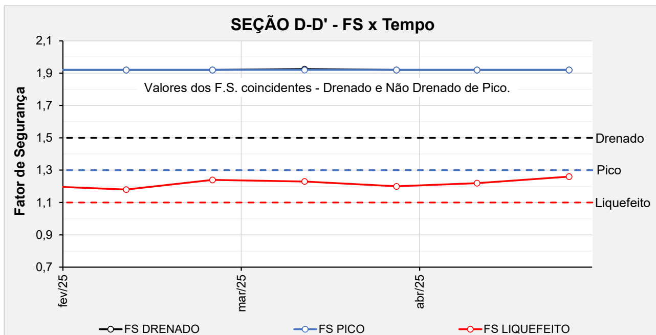
Figura 6.137 – Seção D-D' - Histórico dos F.S. obtidos nas análises de estabilidade no período avaliado.
