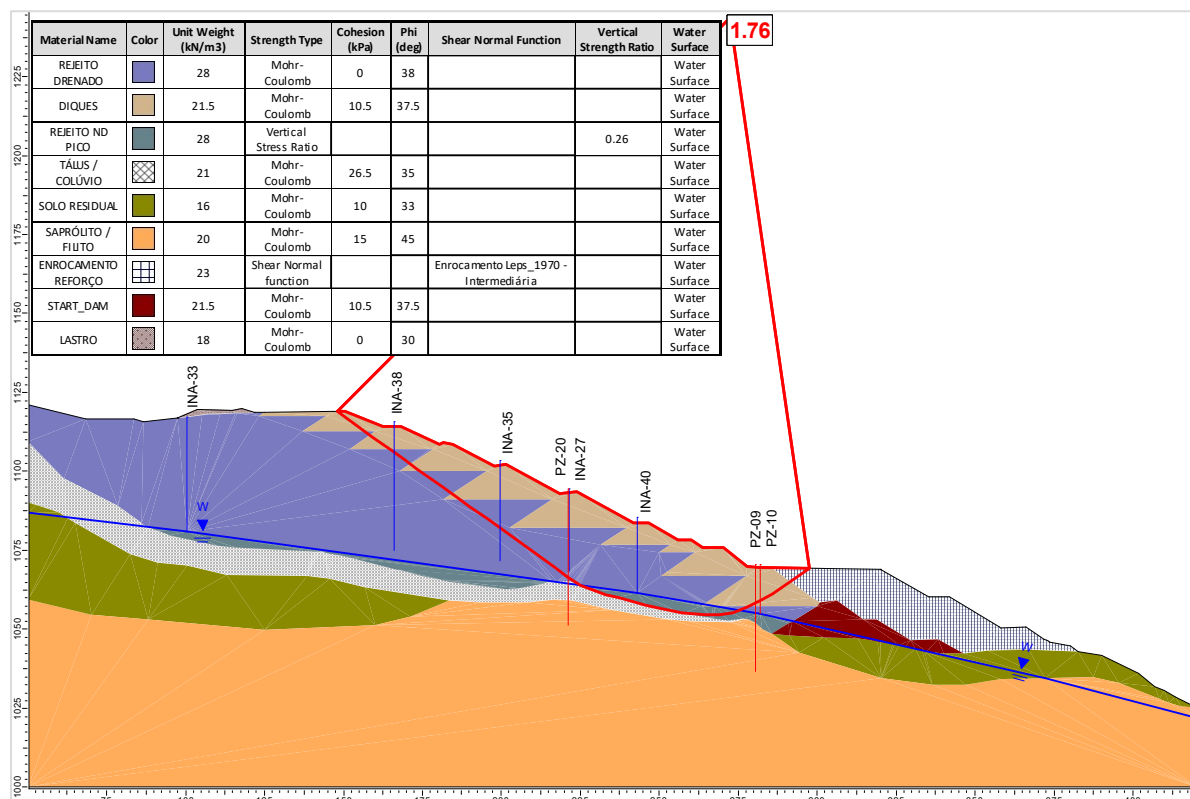
Figura 6.128 – Seção E-E' – Análise Não Drenada – Superfície de ruptura plano-circular otimizada – Freática 30/04/2025 – Razão de resistência não drenada de pico.
