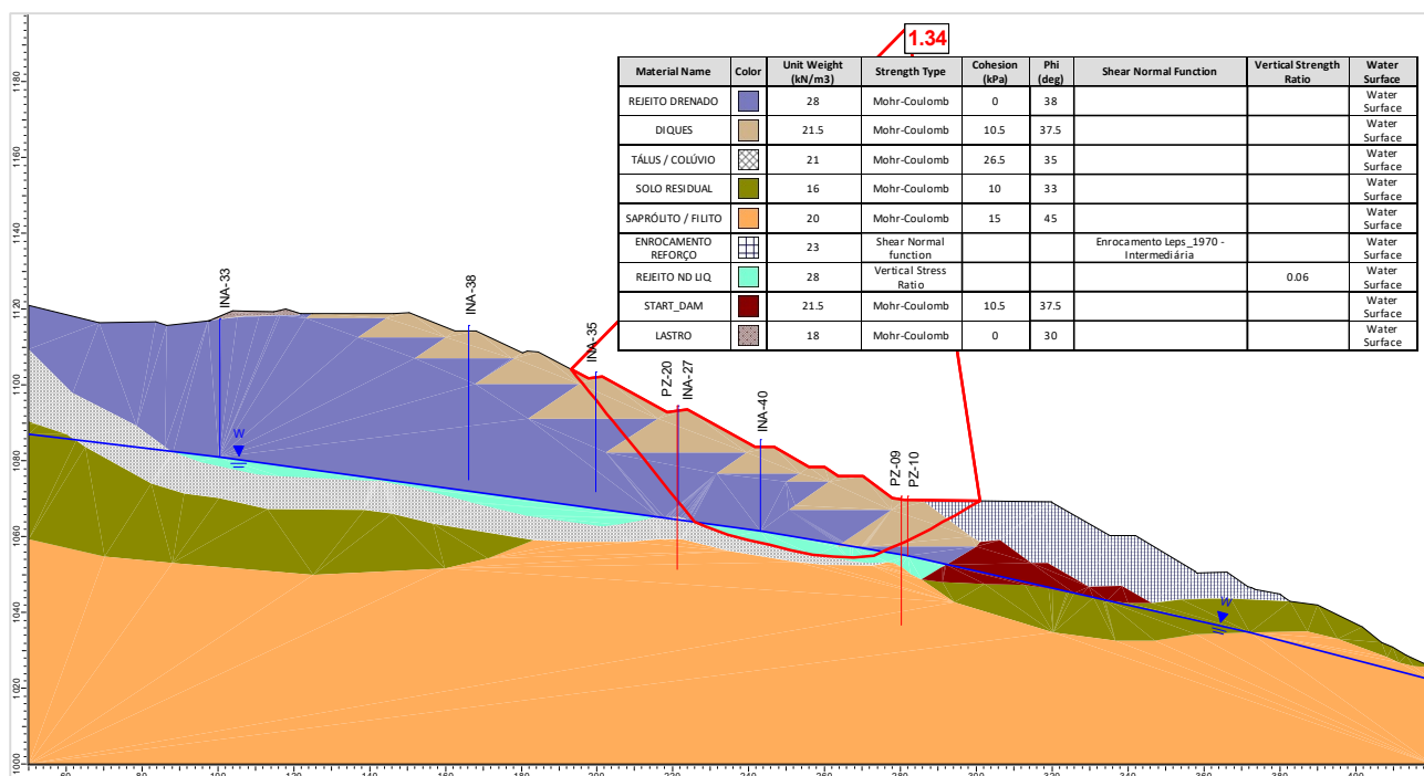
Figura 6.129 – Seção E-E' – Análise Não Drenada – Superfície de ruptura plano-circular otimizada – Freática 30/04/2025 – Razão de resistência não drenada liquefeita.
