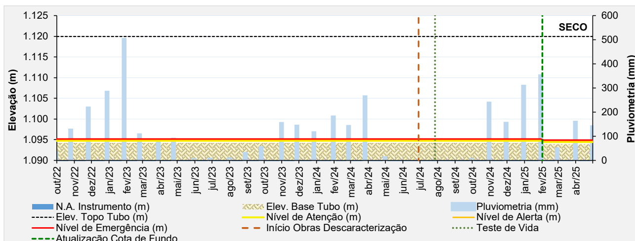
Figura 6.39 – Desempenho do indicador de nível d'água – INA-19.
