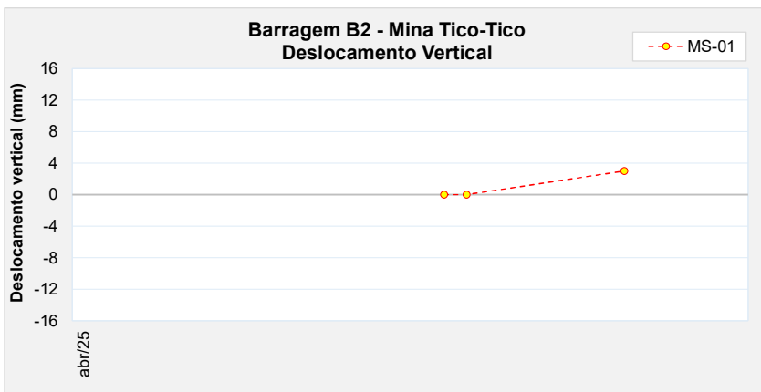
Figura 6.85 – Marco de controle de deformação – MS-01.
