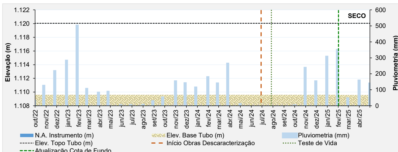
Figura 6.38 – Desempenho do indicador de nível d'água – INA-18.
