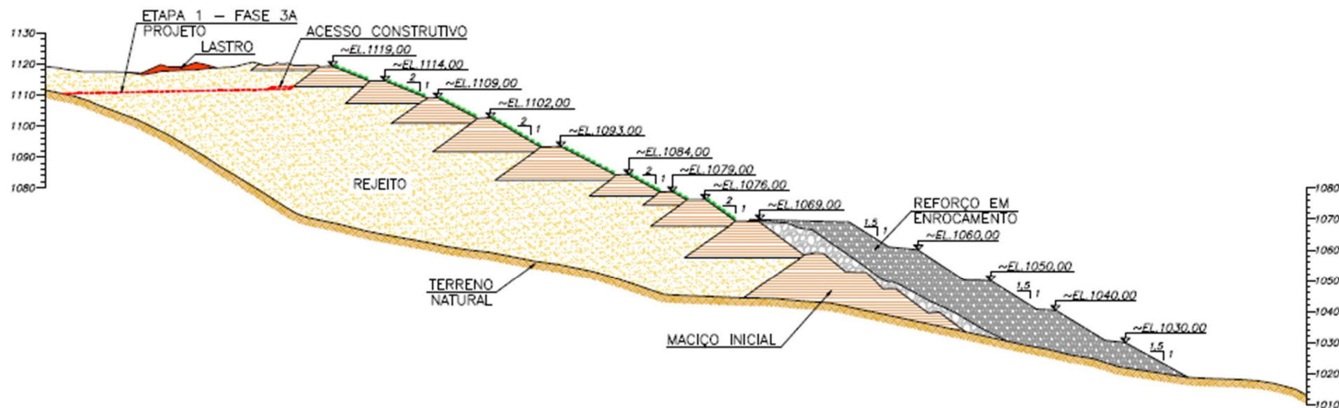
Figura 6.11 – Comparativo Projeto (Etapa 1 - Fase 3A) x Executado – Seção D-D’.
