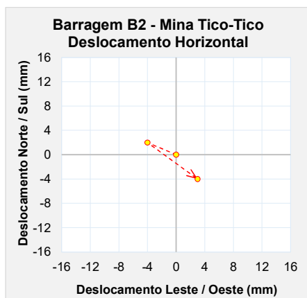
Figura 6.87 – Marco de controle de deformação – MS-03.
