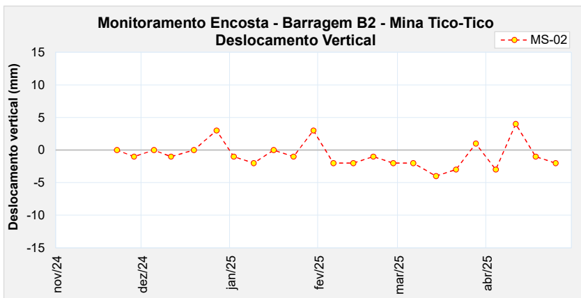
Figura 5.12 – Marco de controle de monitoramento da encosta – MS-02.
