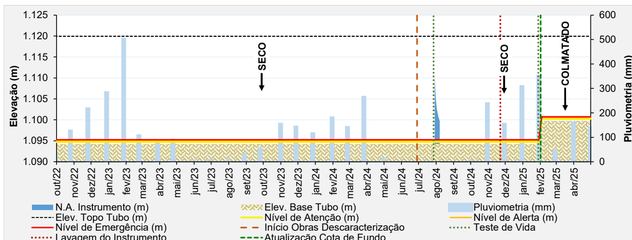
Figura 6.40 – Desempenho do indicador de nível d'água – INA-20.
