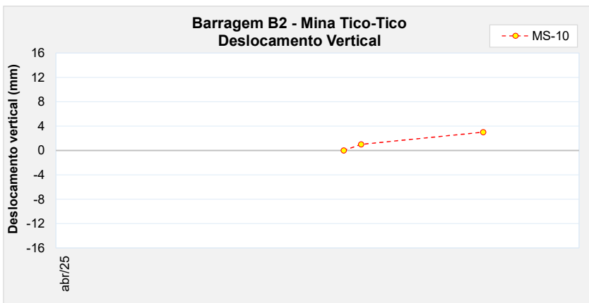
Figura 6.94 – Marco de controle de deformação – MS-10.
