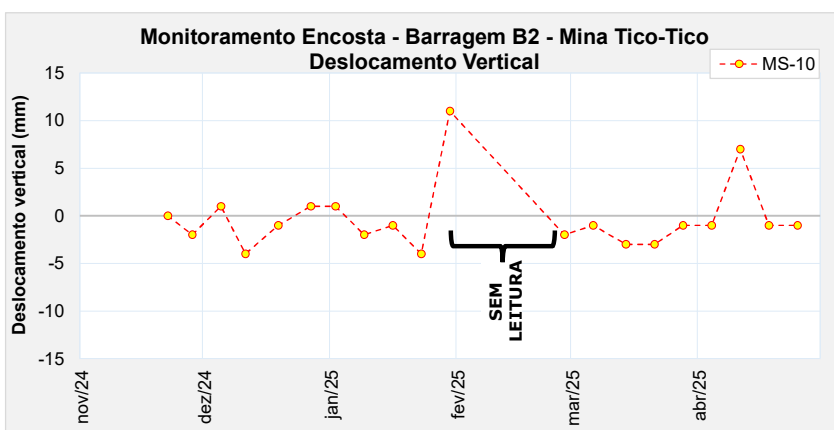
Figura 5.20 – Marco de controle de monitoramento da encosta – MS-10.
