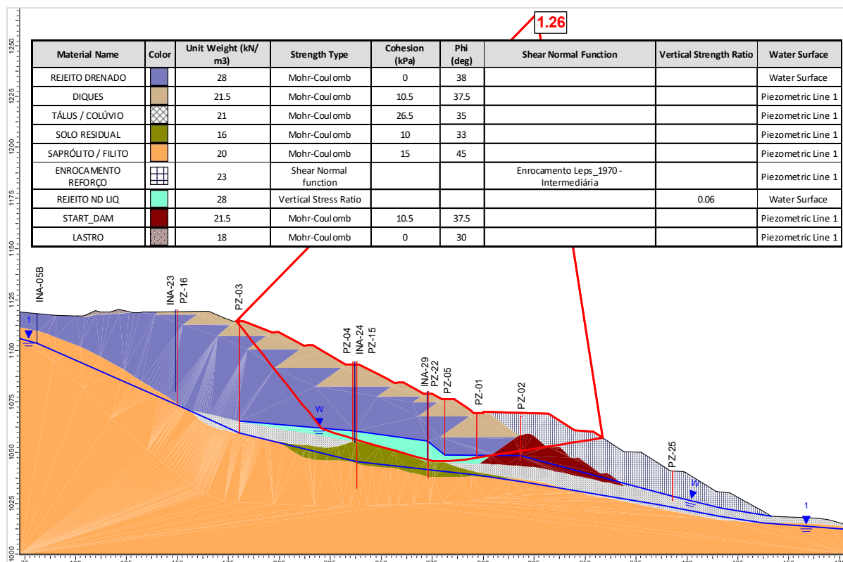
Figura 6.122 – Seção D-D' – Análise Não Drenada – Superfície de ruptura plano-circular otimizada – Freática 30/04/2025 – Razão de resistência não drenada liquefeita.
