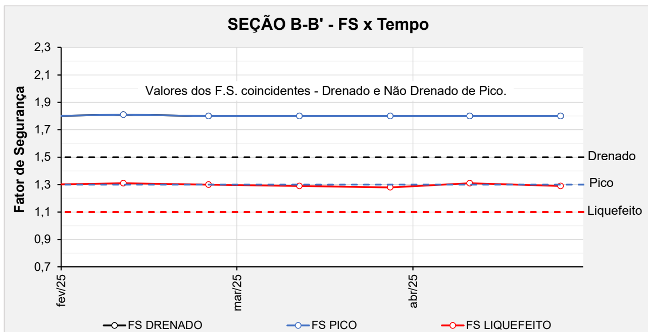
Figura 6.135 – Seção B-B' - Histórico dos F.S. obtidos nas análises de estabilidade no período avaliado.
