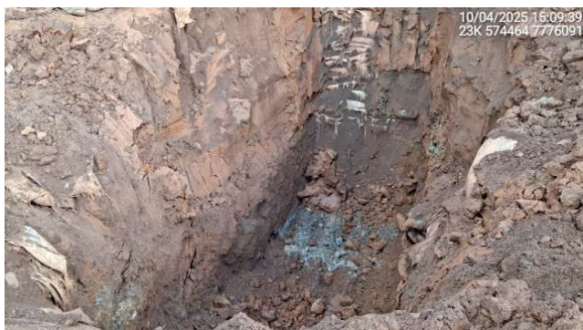
Foto 6.31 – Execução de valas de inspeção em talude escavado no reservatório.
