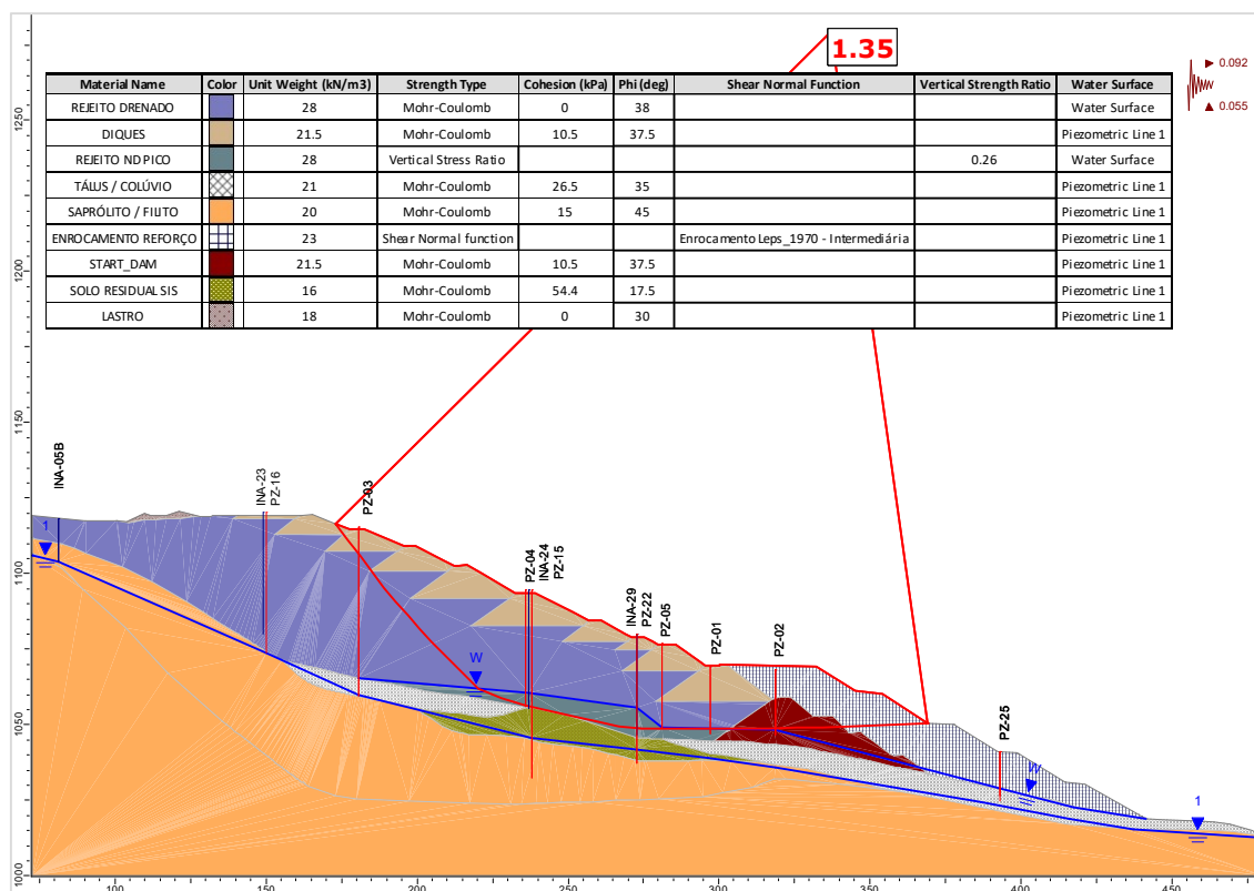
Figura 6.123 – Seção D-D' – Análise Não Drenada – Superfície de ruptura plano-circular otimizada – Freática 30/04/2025 – Razão de resistência não drenada de pico + sismo ↑ (critério CDA).
