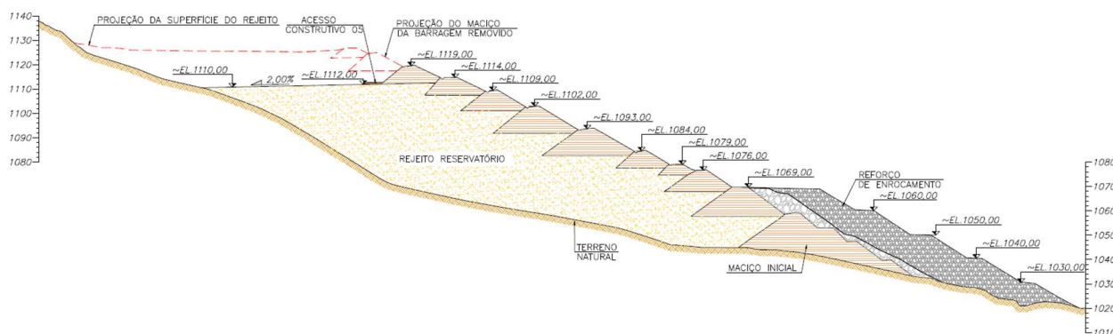
Figura 6.3 – Sequência Construtiva – Seção D-D' – Etapa 1 - Fase 3A (IPE.OP.DE.8000.GT.20.717).
