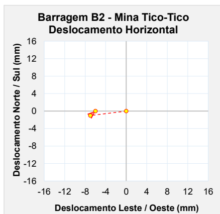
Figura 6.85 – Marco de controle de deformação – MS-01.
