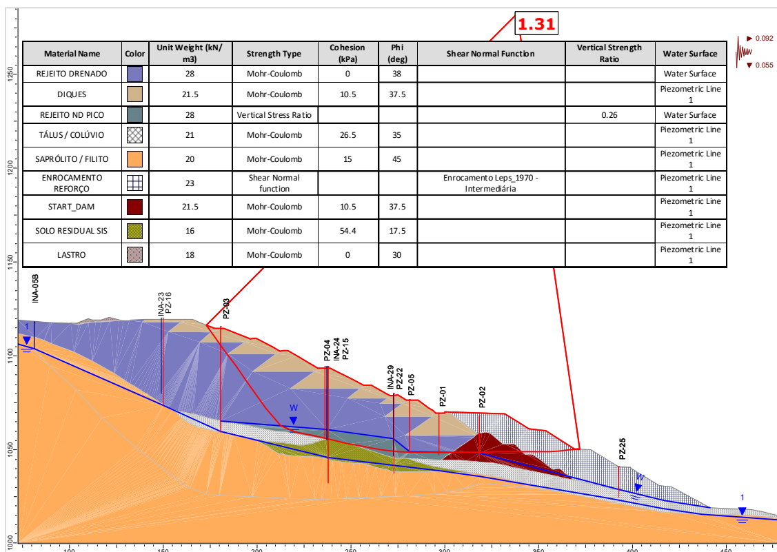
Figura 6.124 – Seção D-D' – Análise Não Drenada – Superfície de ruptura plano-circular otimizada – Freática 30/04/2025 – Razão de resistência não drenada de pico + sismo ↓ (critério CDA).
