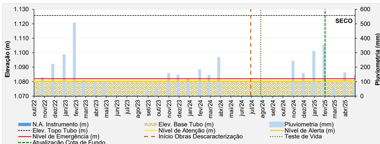
Figura 6.41 – Desempenho do indicador de nível d'água – INA-23.
