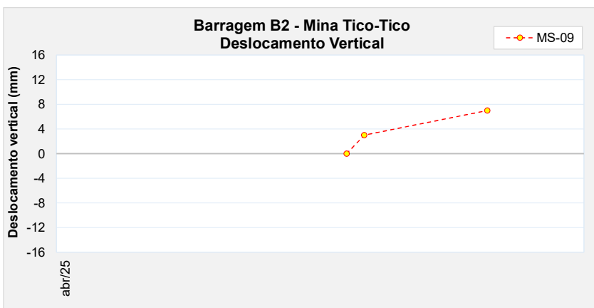
Figura 6.93 – Marco de controle de deformação – MS-09.
