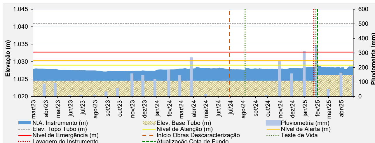
Figura 6.83 – Desempenho do piezômetro de tubo aberto – PZ-25.
