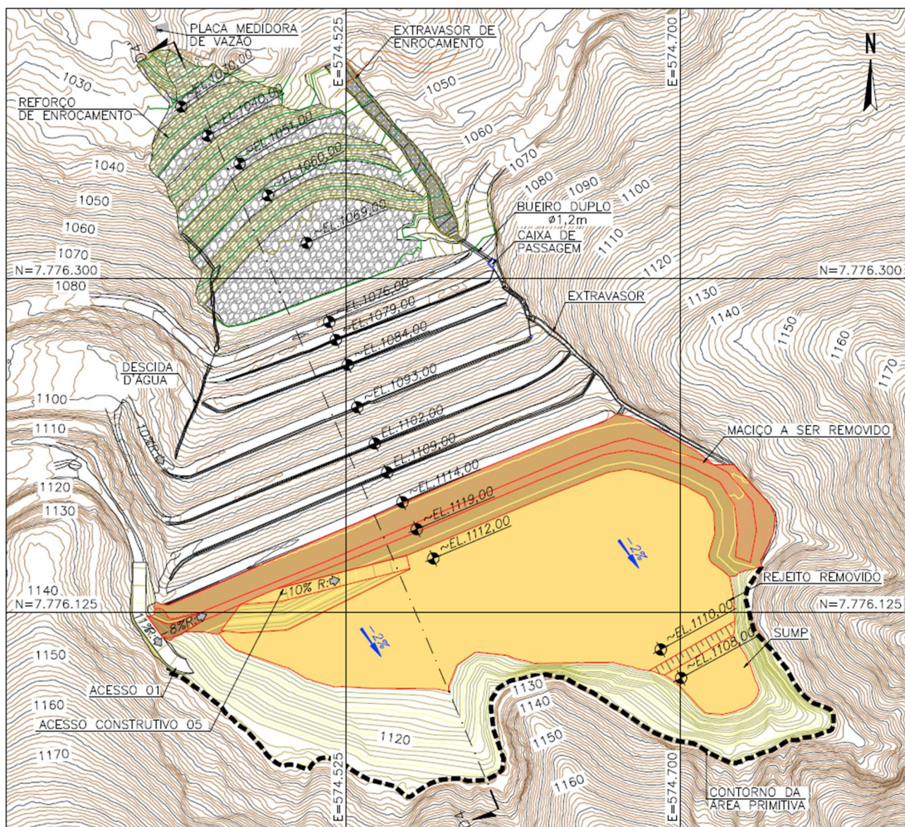
Figura 6.2 – Sequência Construtiva – Planta – Etapa 1-Fase 3A (IPE.OP.DE.8000.GT.20.747).
