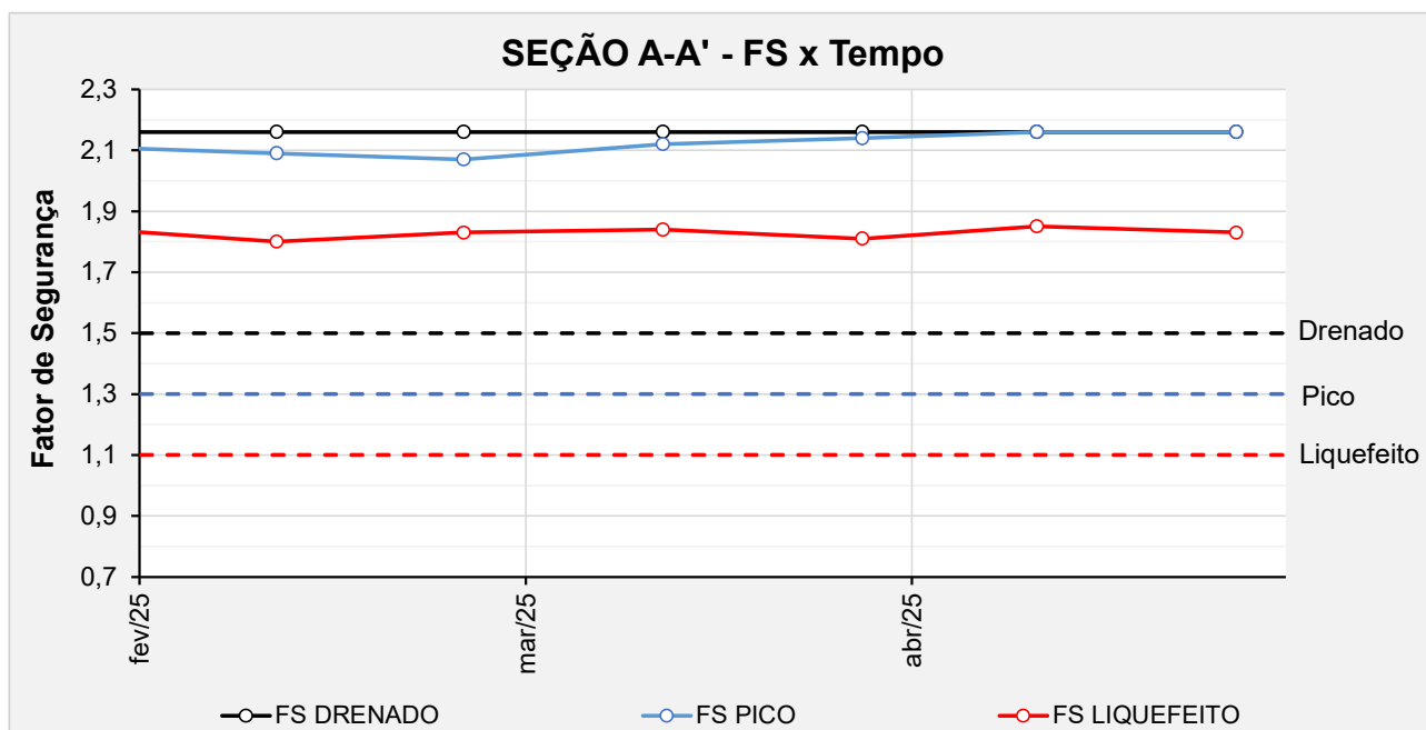
Figura 6.134 – Seção A-A' - Histórico dos F.S. obtidos nas análises de estabilidade no período avaliado.
