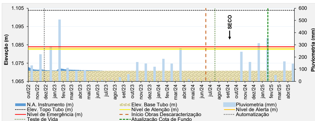
Figura 6.54 – Desempenho do indicador de nível d'água automatizado – INA-36.
