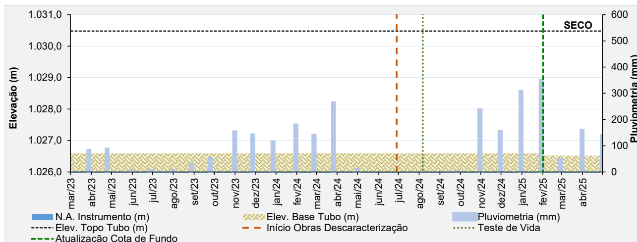
Figura 6.82 – Desempenho do piezômetro de tubo aberto – PZ-24.
