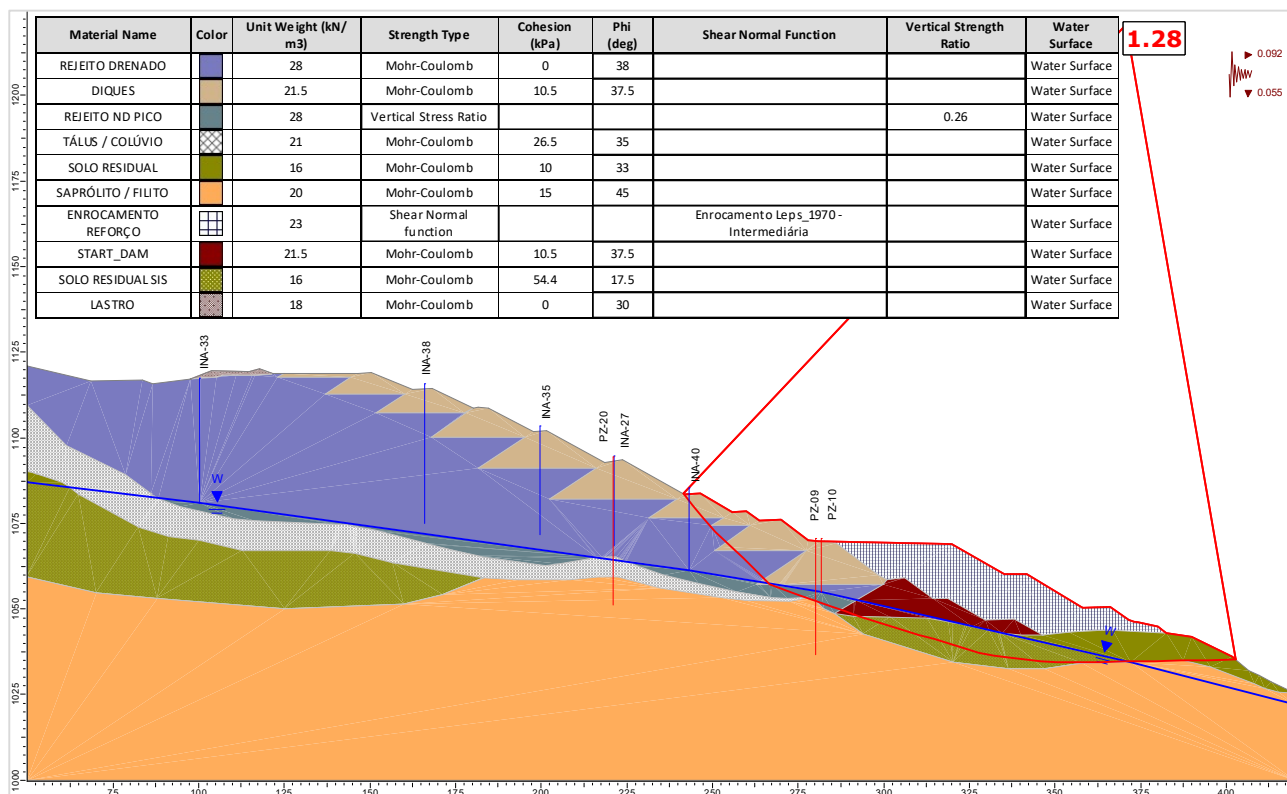
Figura 6.131 – Seção E-E' – Análise Não Drenada – Superfície de ruptura plano-circular otimizada – Freática 30/04/2025 – Razão de resistência não drenada de pico + sismo ↓ (critério CDA).
