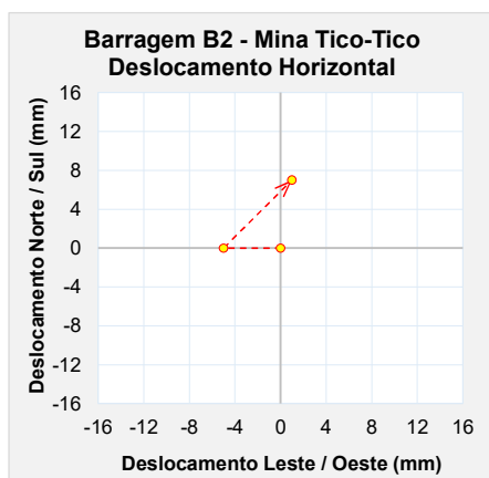
Figura 6.89 – Marco de controle de deformação – MS-05.
