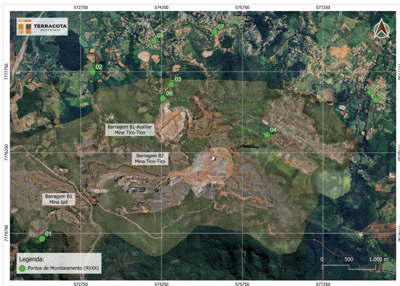
Figura 6.144 – Localização dos pontos de monitoramento de qualidade do ar.
