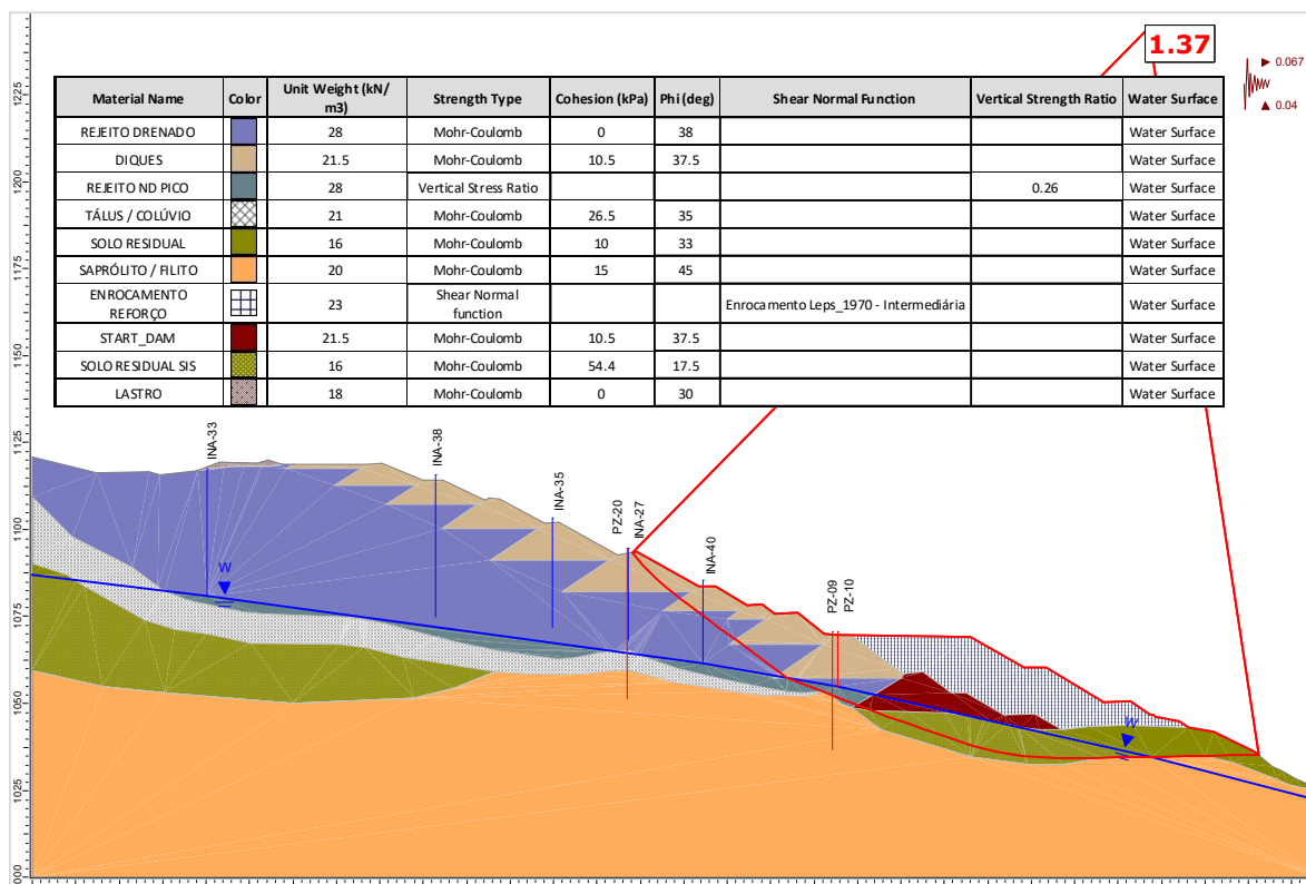
Figura 6.132 – Seção E-E' – Análise Não Drenada – Superfície de ruptura plano-circular otimizada – Freática 30/04/2025 – Razão de resistência não drenada de pico + sismo ↑ (critério vida útil).
