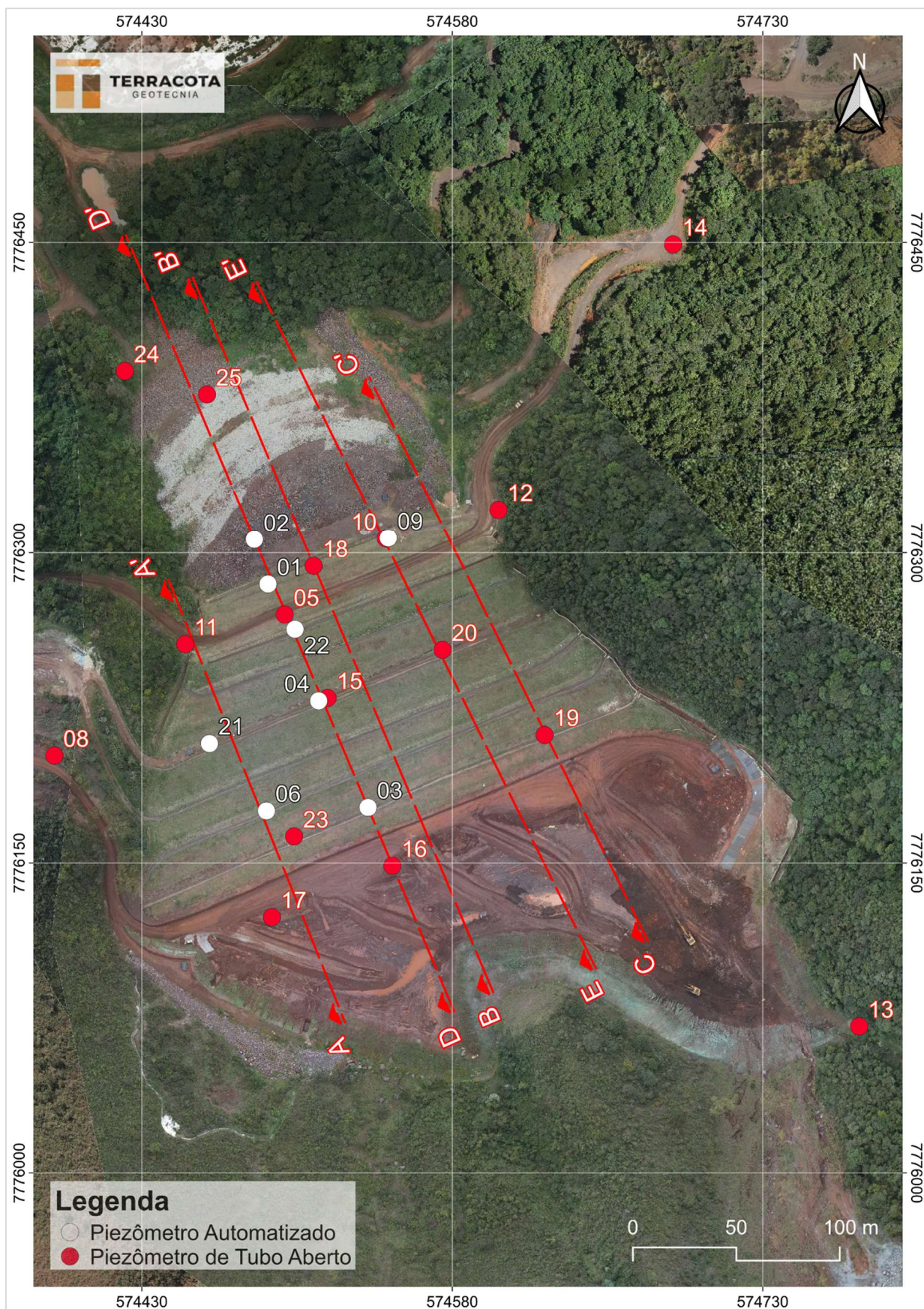
Figura 6.15 – Localização dos piezômetros.
