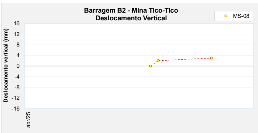
Figura 6.92 – Marco de controle de deformação – MS-08.
