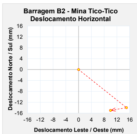
Figura 6.92 – Marco de controle de deformação – MS-08.
