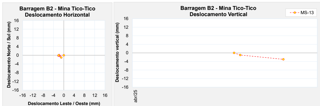
Figura 6.97 – Marco de controle de deformação – MS-13.
