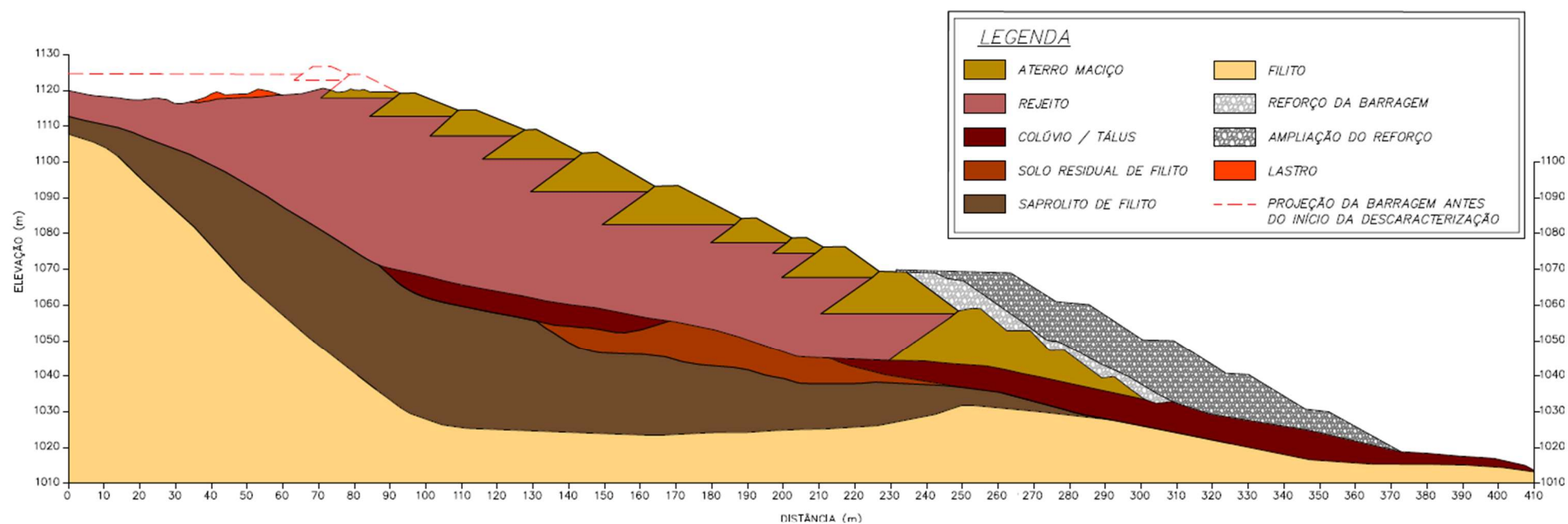
Figura 4.3 – Seção de maior altura (D-D') da Barragem B2 – Mina Tico-Tico (Condição em abril de 2025).
