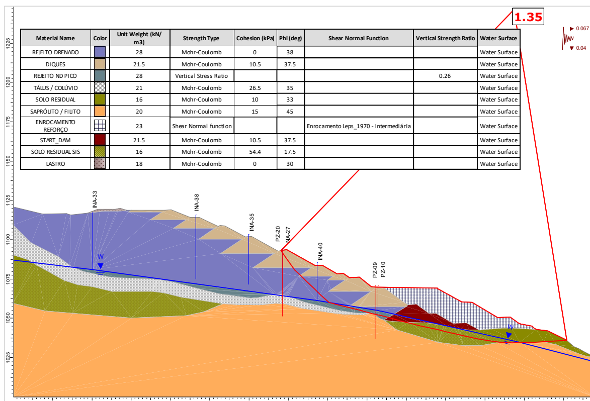
Figura 6.133 – Seção E-E' – Análise Não Drenada – Superfície de ruptura plano-circular otimizada – Freática 30/04/2025 – Razão de resistência não drenada de pico + sismo ↓ (critério vida útil).
