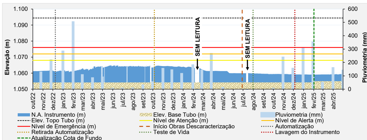
Figura 6.42 – Desempenho do indicador de nível d'água – INA-24.
