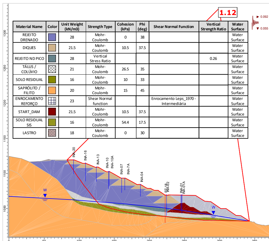
Figura 6.112 – Seção B-B' – Análise Não Drenada – Superfície de ruptura plano-circular otimizada – Freática 30/04/2025 – Razão de resistência não drenada de pico + sismo ↓ (critério CDA).
