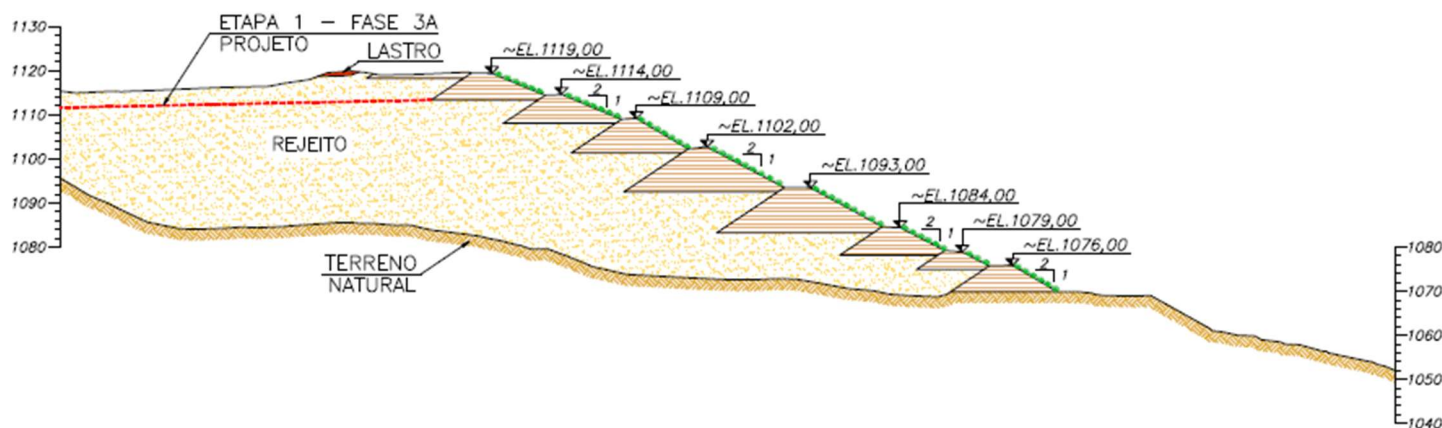
Figura 6.10 – Comparativo Projeto (Etapa 1 - Fase 3A) x Executado – Seção C-C’.
