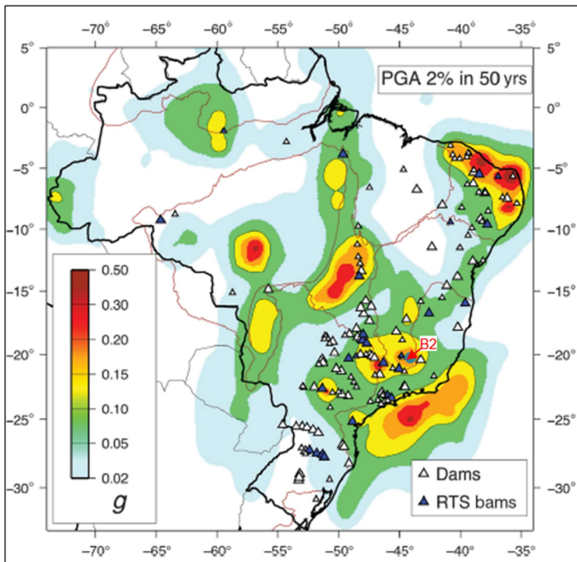
Figura 6.100 – Mapa de Ameaça Sísmica Brasileiro com probabilidade de excedência de 2% durante 50 anos (Assumpção Et al., 2018).
