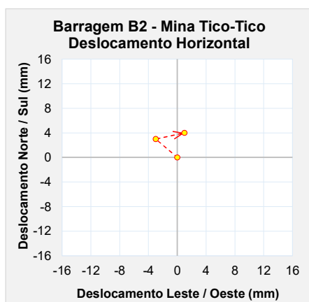
Figura 6.90 – Marco de controle de deformação – MS-06.
