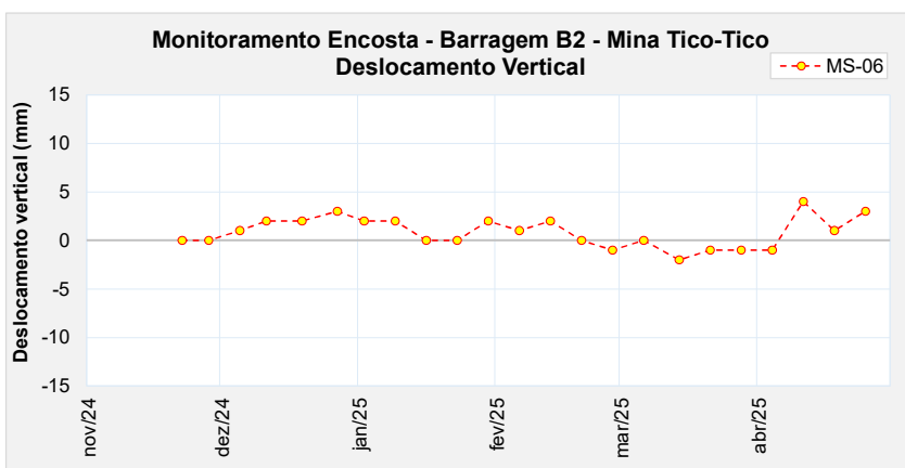
Figura 5.16 – Marco de controle de monitoramento da encosta – MS-06.
