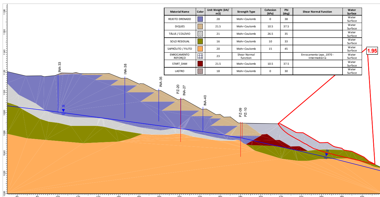
Figura 6.127 – Seção E-E' – Análise Drenada – Superfície de ruptura plano-circular otimizada – Freática 30/04/2025.
