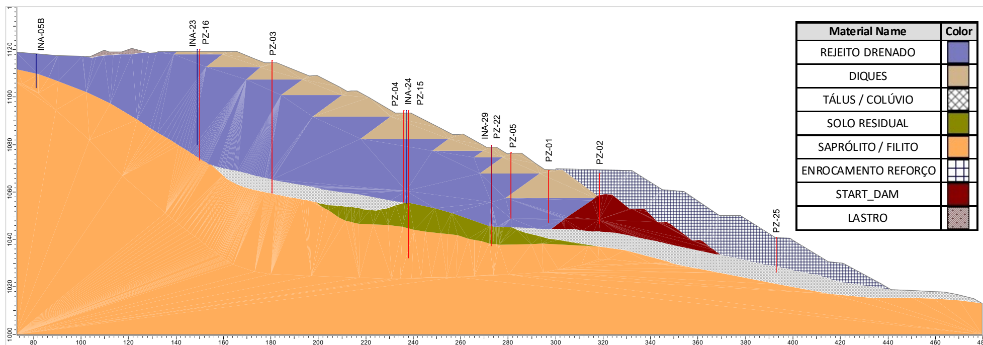
Figura 6.20 – Seção transversal de controle D-D' (Condição em 01/05/2025).
