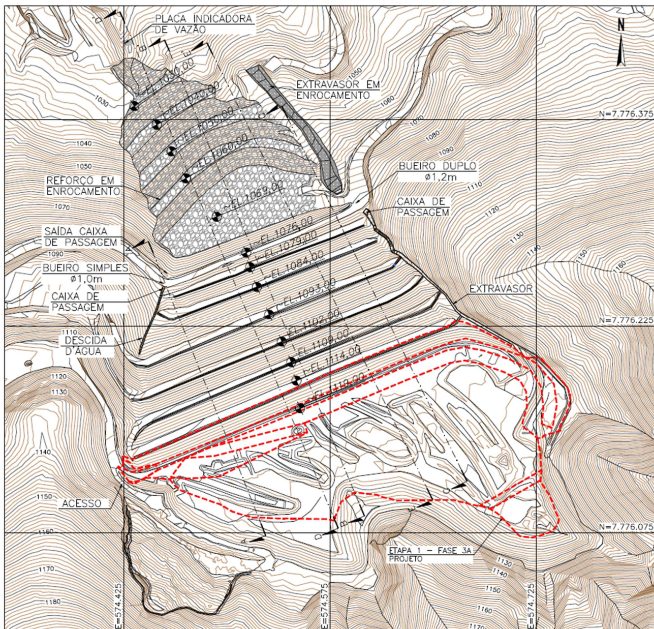
Figura 6.7 – Comparativo Projeto (Etapa 1 - Fase 3A) x Executado – Planta.
