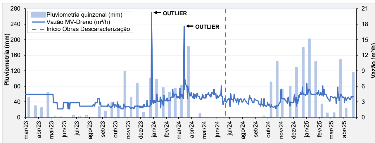
Figura 6.84 – Vazão – MV-Dreno – Barragem B2 – Mina Tico-Tico.
