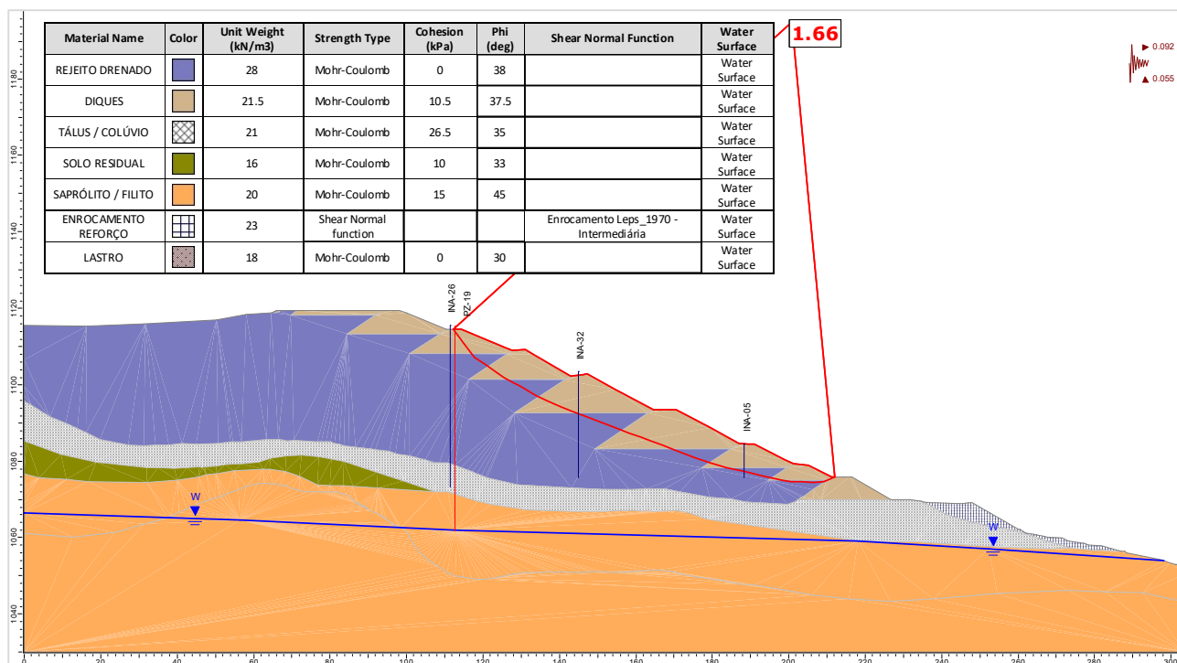
Figura 6.116 – Seção C-C' – Análise Drenada – Superfície de ruptura plano-circular otimizada – Freática 30/04/2025 – Carregamento sísmico ↑ (critério CDA).
