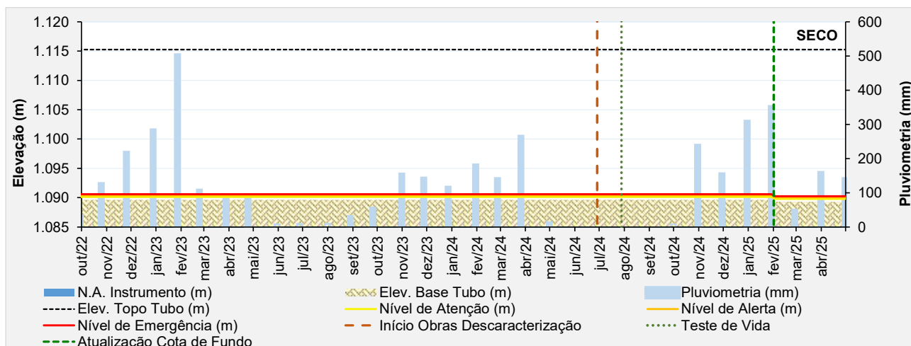
Figura 6.37 – Desempenho do indicador de nível d'água – INA-16.
