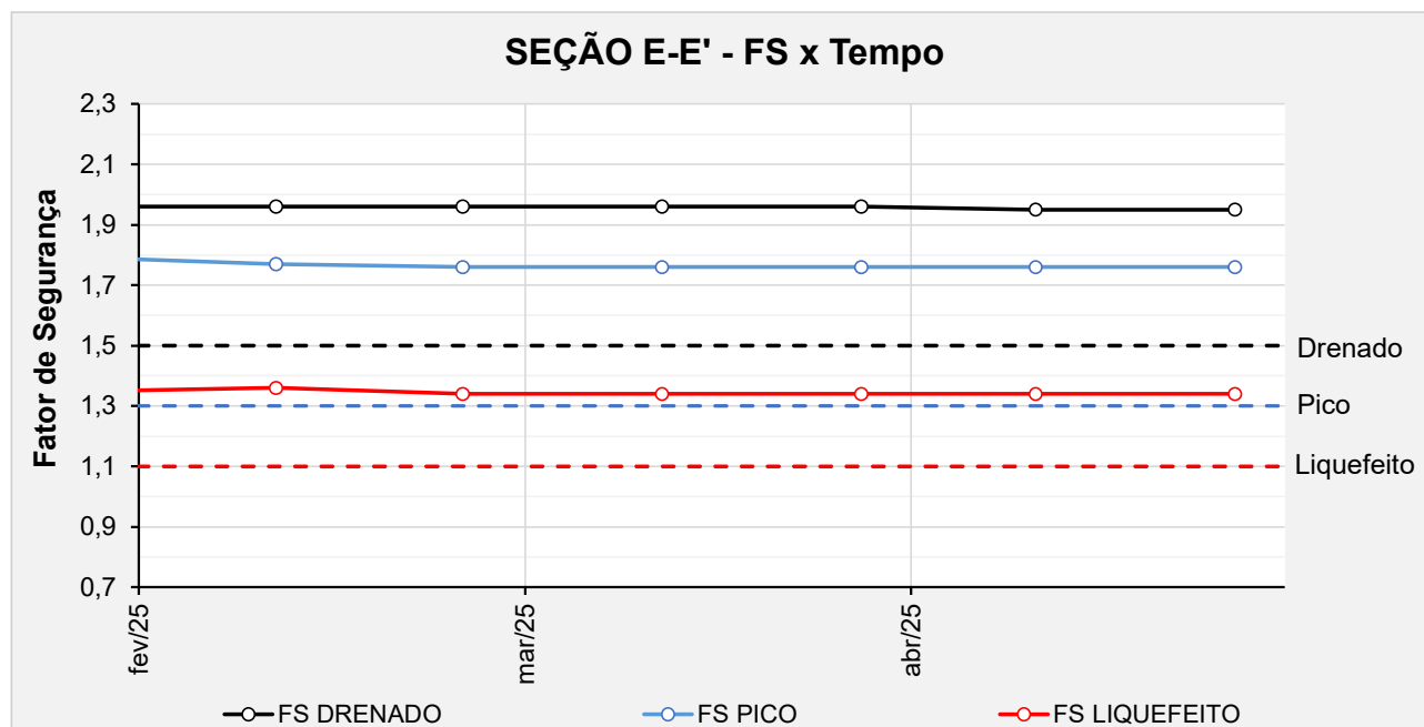
Figura 6.138 – Seção E-E' - Histórico dos F.S. obtidos nas análises de estabilidade no período avaliado.
