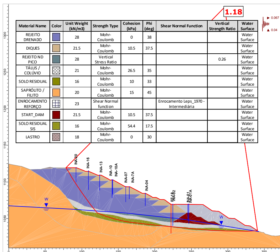
Figura 6.113 – Seção B-B' – Análise Não Drenada – Superfície de ruptura plano-circular otimizada – Freática 30/04/2025 – Razão de resistência não drenada de pico + sismo ↑ (critério vida útil).
