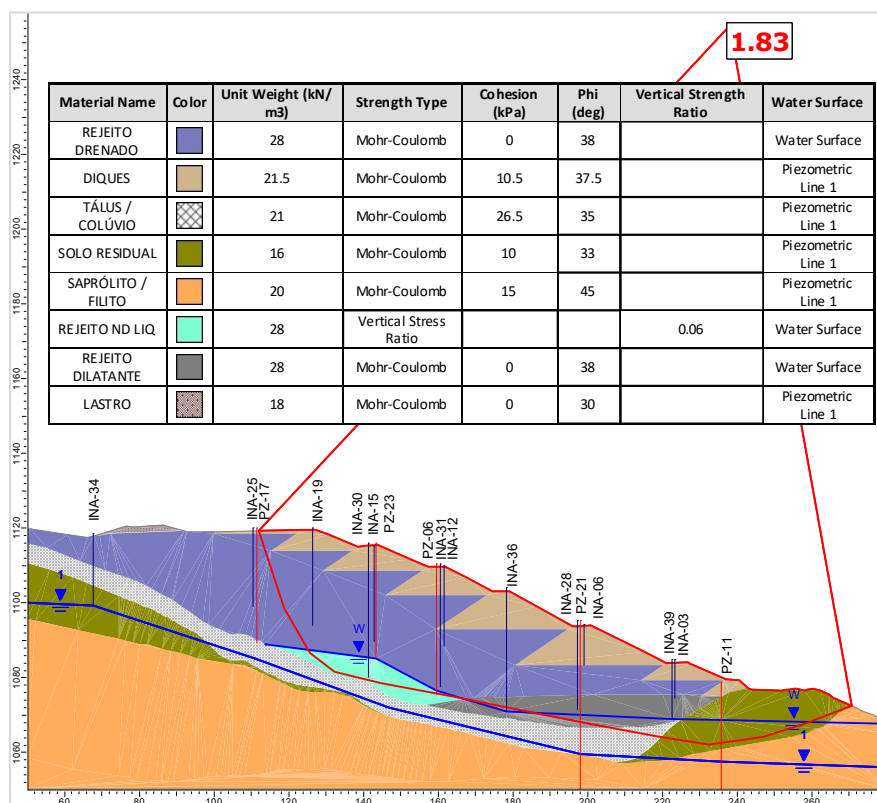
Figura 6.103 – Seção A-A' – Análise Não Drenada – Superfície de ruptura plano-circular otimizada – Freática 30/04/2025 – Razão de resistência não drenada liquefeita.
