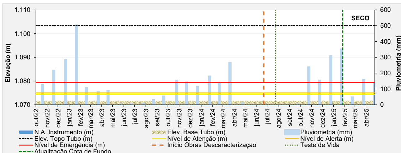
Figura 6.53 – Desempenho do indicador de nível d'água – INA-35.
