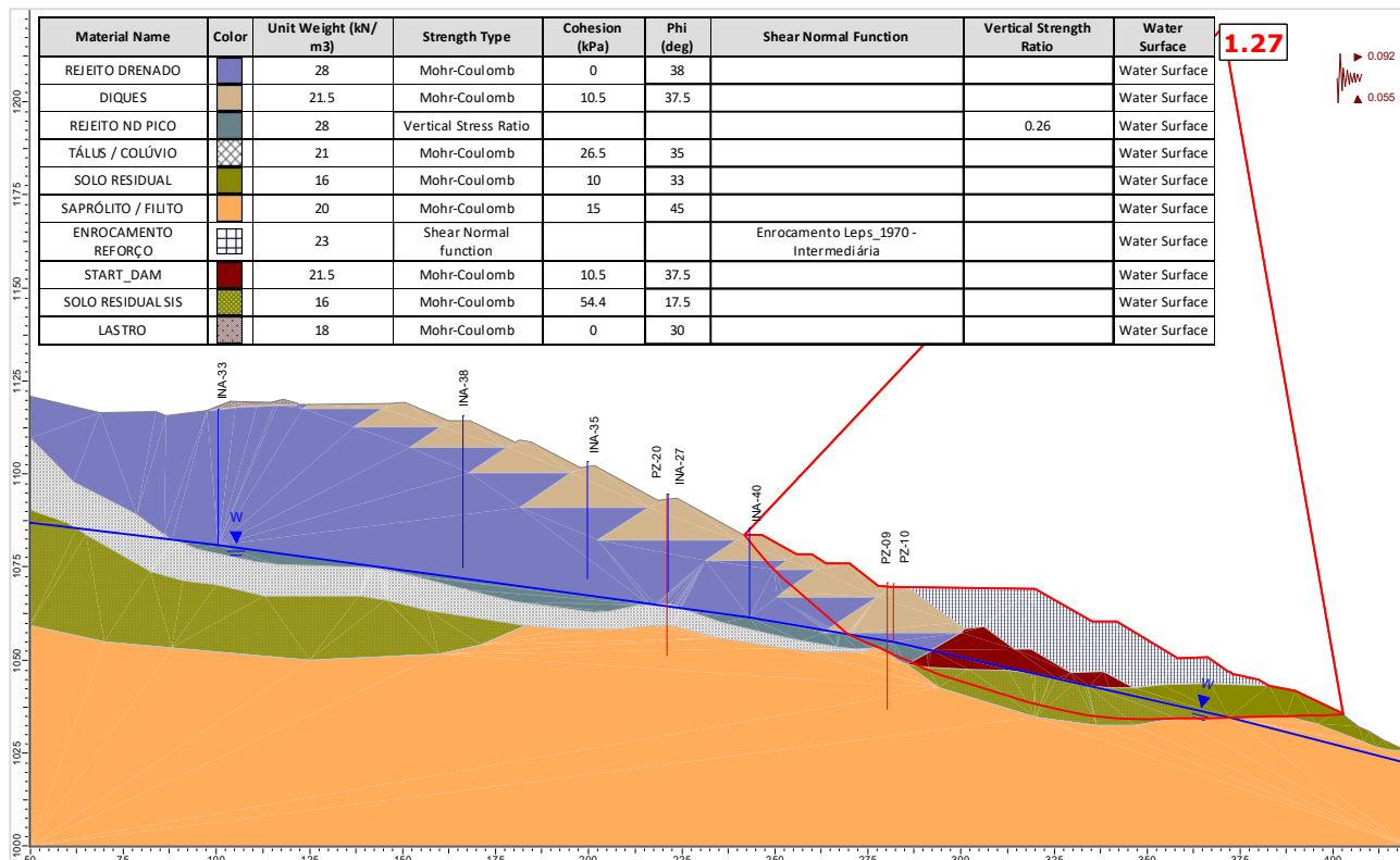
Figura 6.130 – Seção E-E' – Análise Não Drenada – Superfície de ruptura plano-circular otimizada – Freática 30/04/2025 – Razão de resistência não drenada de pico + sismo ↑ (critério CDA).
