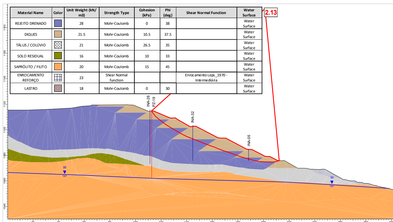
Figura 6.115 – Seção C-C' – Análise Drenada – Superfície de ruptura plano-circular otimizada – Freática 30/04/2025.
