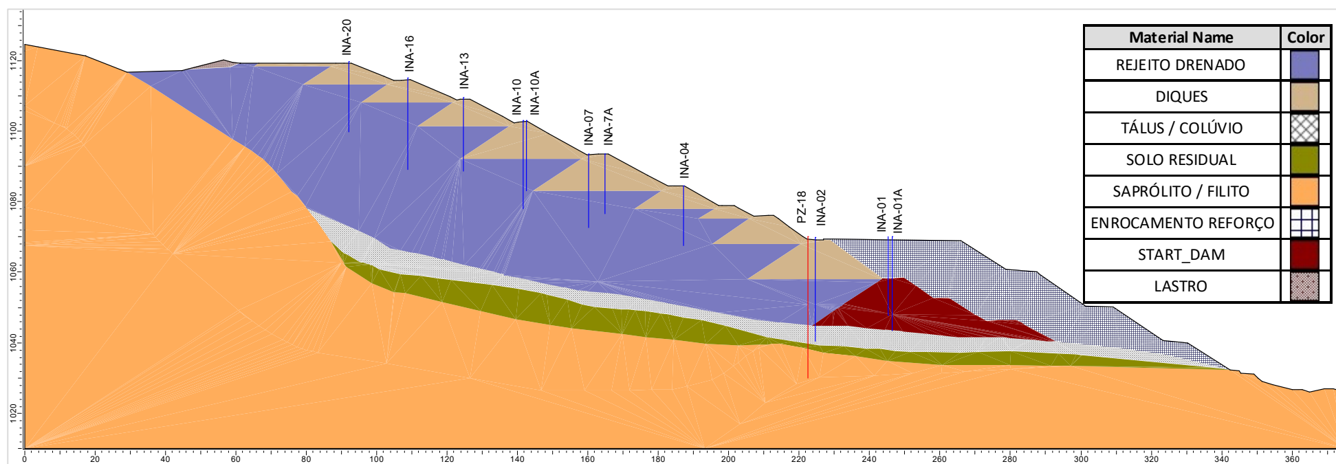
Figura 6.18 – Seção transversal de controle B-B' (Condição em 01/05/2025).
