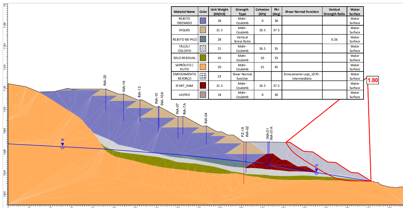
Figura 6.109 – Seção B-B' – Análise Não Drenada – Superfície de ruptura plano-circular otimizada – Freática 30/04/2025 – Razão de resistência não drenada de pico.
