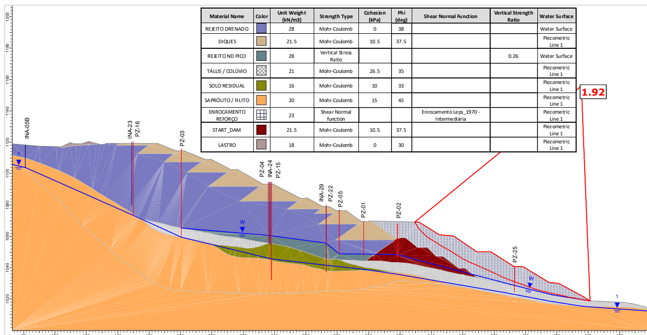
Figura 6.121 – Seção D-D' – Análise Não Drenada – Superfície de ruptura plano-circular otimizada – Freática 30/04/2025 – Razão de resistência não drenada de pico.
