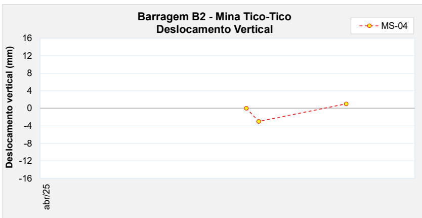
Figura 6.88 – Marco de controle de deformação – MS-04.
