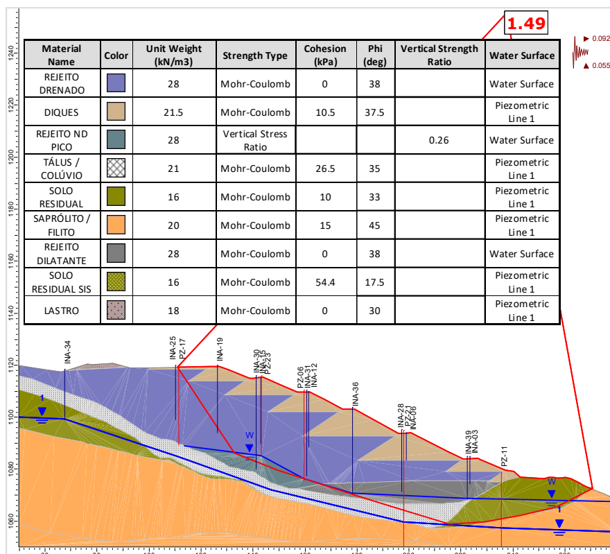
Figura 6.104 – Seção A-A' – Análise Não Drenada – Superfície de ruptura plano-circular otimizada – Freática 30/04/2025 – Razão de resistência não drenada de pico + sismo ↑ (critério CDA).
