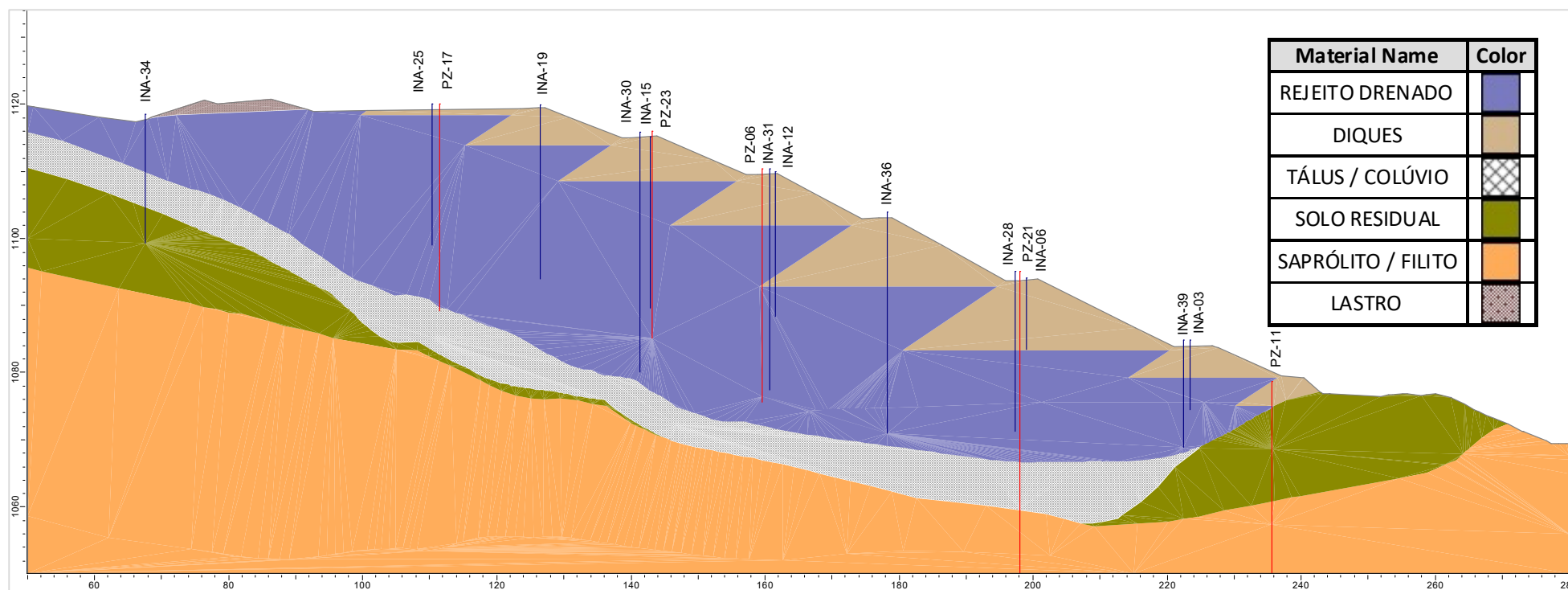
Figura 6.17 – Seção transversal de controle A-A' (Condição em 01/05/2025).
