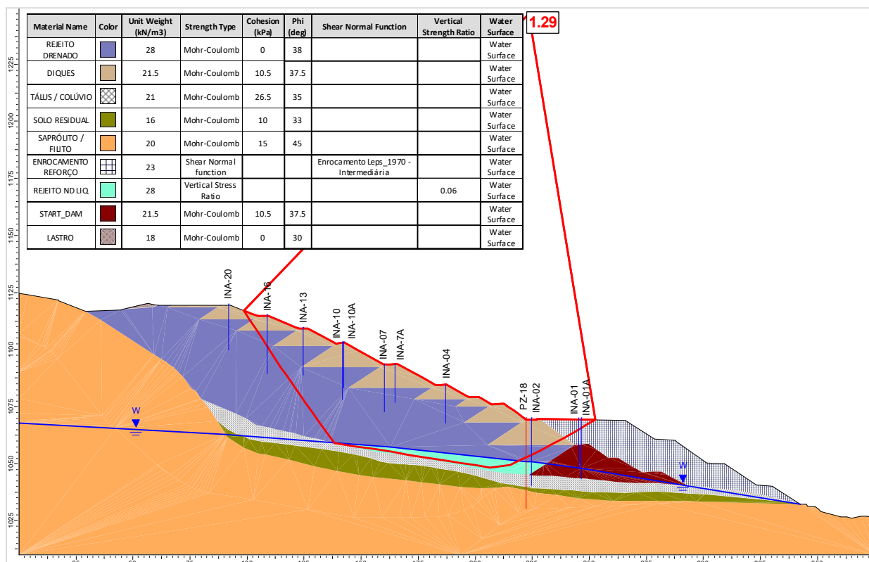
Figura 6.110 – Seção B-B' – Análise Não Drenada – Superfície de ruptura plano-circular otimizada – Freática 30/04/2025 – Razão de resistência não drenada liquefeita.
