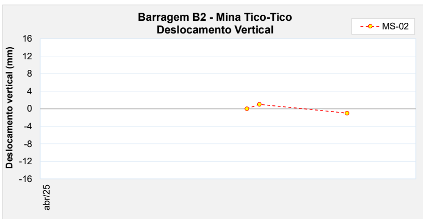
Figura 6.86 – Marco de controle de deformação – MS-02.
