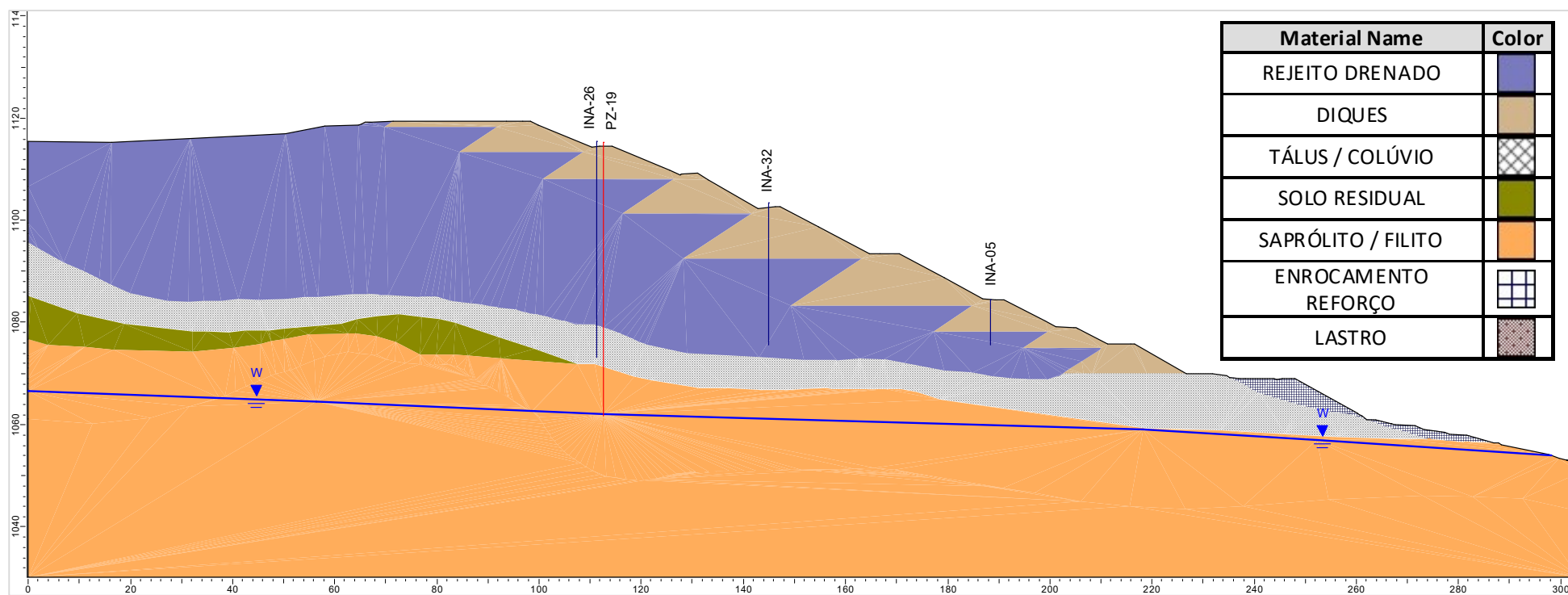
Figura 6.19 – Seção transversal de controle C-C' (Condição em 01/05/2025).
