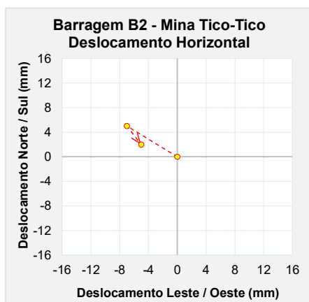
Figura 6.86 – Marco de controle de deformação – MS-02.
