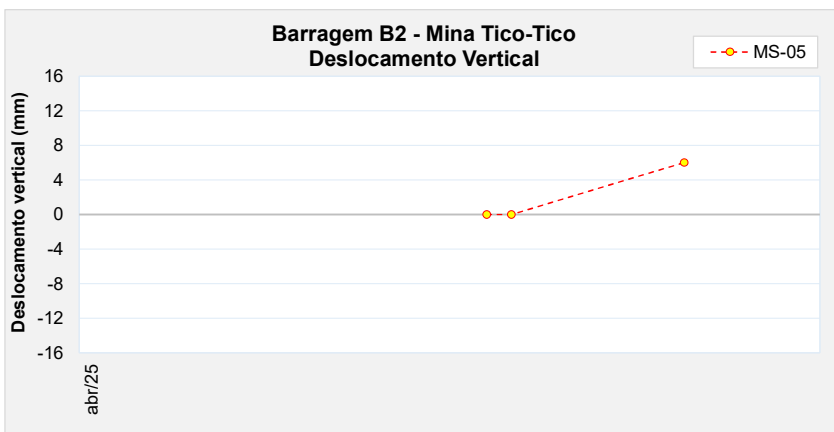
Figura 6.89 – Marco de controle de deformação – MS-05.
