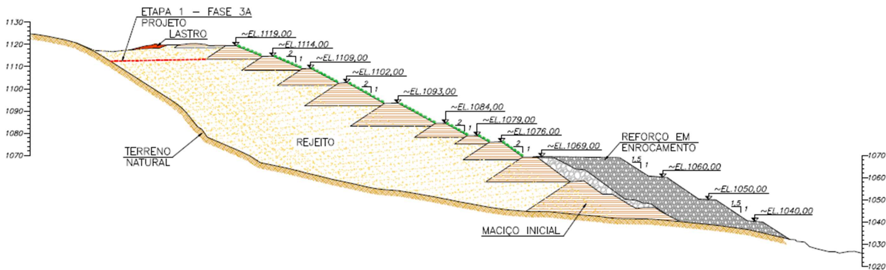
Figura 6.9 – Comparativo Projeto (Etapa 1 - Fase 3A) x Executado – Seção B-B'.
