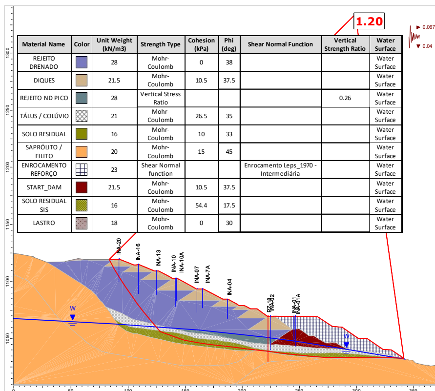
Figura 6.114 – Seção B-B' – Análise Não Drenada – Superfície de ruptura plano-circular otimizada – Freática 30/04/2025 – Razão de resistência não drenada de pico + sismo ↓ (critério vida útil).
