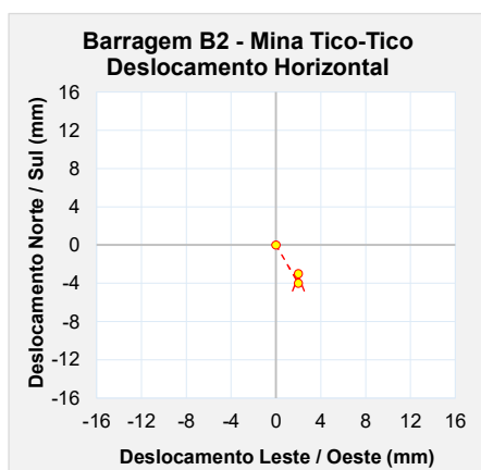
Figura 6.96 – Marco de controle de deformação – MS-12.
