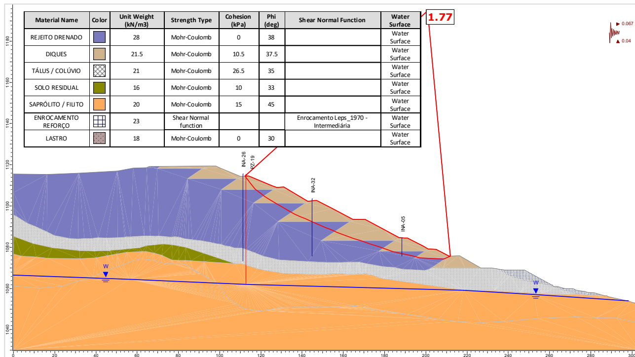
Figura 6.118 – Seção C-C' – Análise Drenada – Superfície de ruptura plano-circular otimizada – Freática 30/04/2025 – Carregamento sísmico ↑ (critério vida útil).
