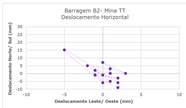
Figura 6.31 – Marco de controle de deformação – MS-04.
