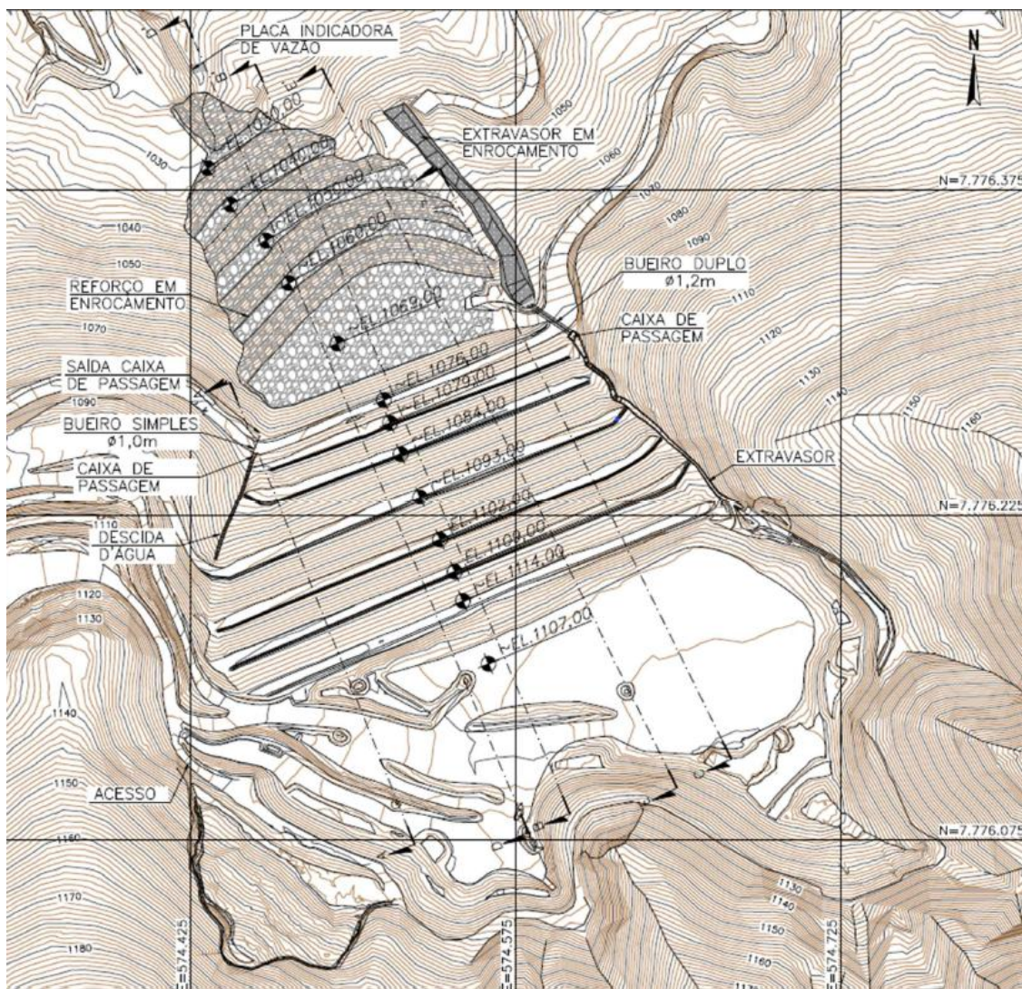
Figura 6.5 – Levantamento topográfico 31/07/2025 – Obras Executadas - Planta.
