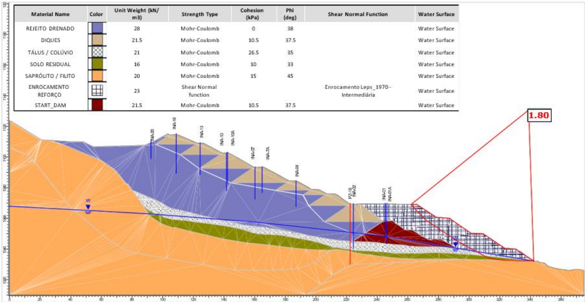
Figura 6.49 – Seção B-B’ – Análise Drenada – Superfície de ruptura plano-circular otimizada – Freática 31/07/2025.
