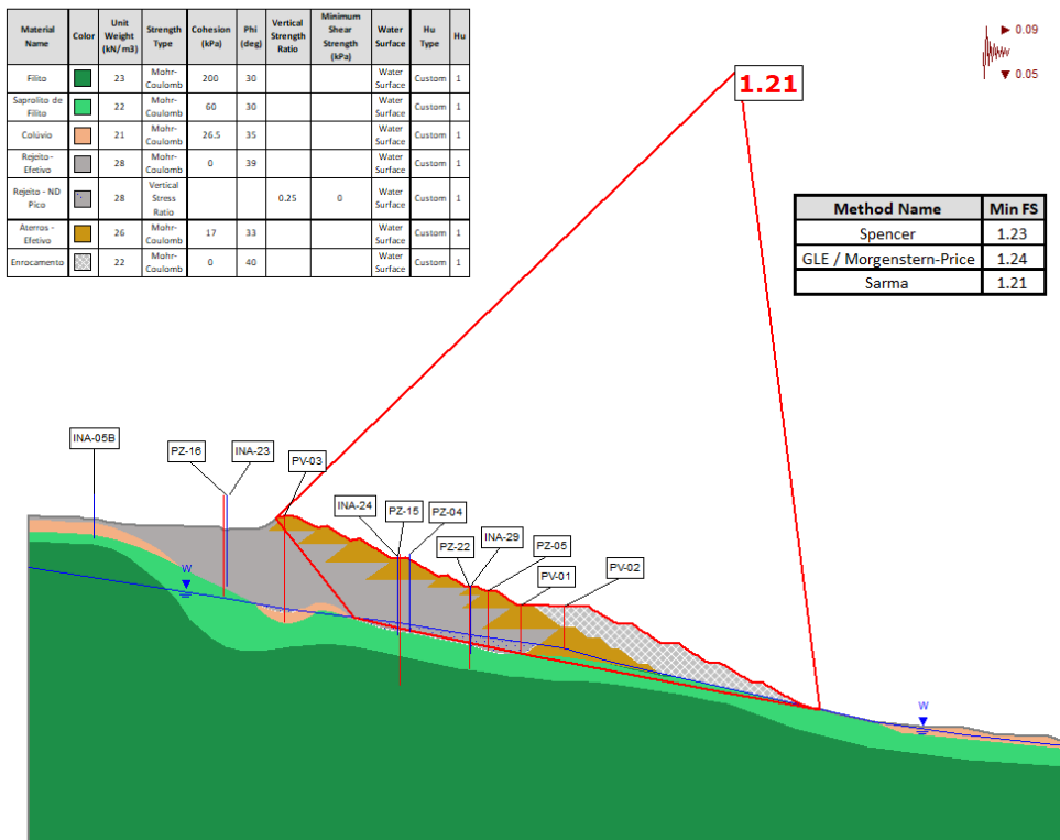
Figura 6.61 – Seção D-D’ – Análise Não Drenada – Carregamento Pseudo-Estático sismo ↓
