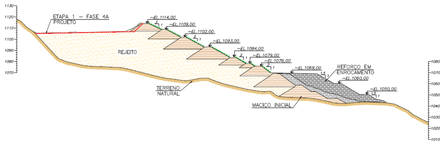
Figura 6.12 – Comparativo Projeto (Etapa 1 - Fase 3A) x Executado – Seção E-E’.
