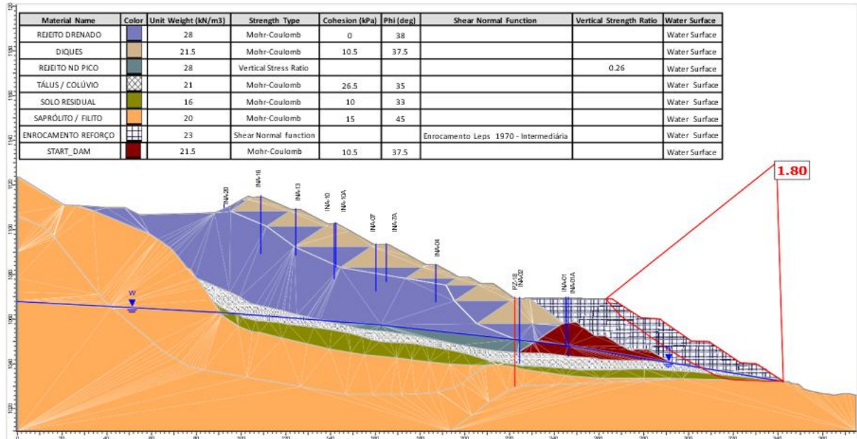
Figura 6.50 – Seção B-B’ – Análise Não Drenada – Superfície de ruptura plano-circular otimizada – Freática 31/07/2025 – Razão de resistência não drenada de pico.
