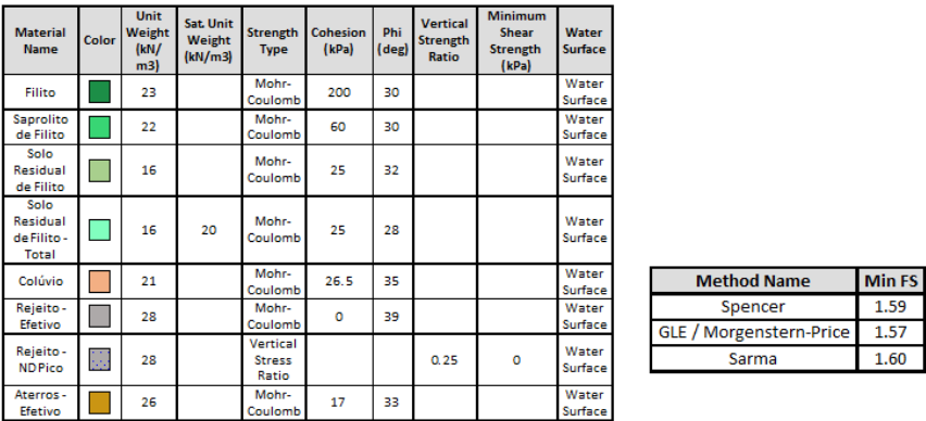
Figura 6.46 – Seção A-A’ – Análise Não Drenada – Superfície de ruptura plano-circular otimizada – Freática 31/07/2025 – Razão de resistência não drenada liquefeita.
