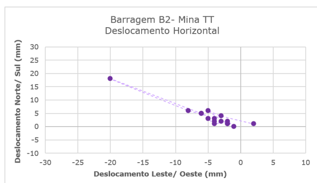
Figura 6.39 – Marco de controle de deformação – MS-12.
