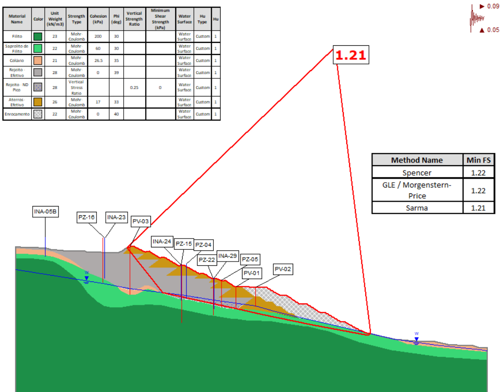
Figura 6.60 – Seção D-D’ – Análise Não Drenada – Carregamento Pseudo-Estático sismo ↑
