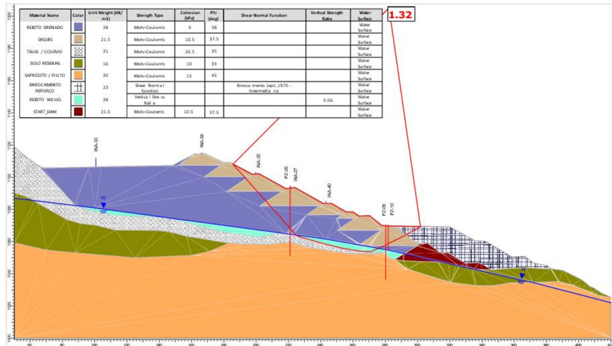
Figura 6.64 – Seção E-E' – Análise Não Drenada – Superfície de ruptura plano-circular otimizada – Freática 31/07/2025 – Razão de resistência não drenada liquefeita.
