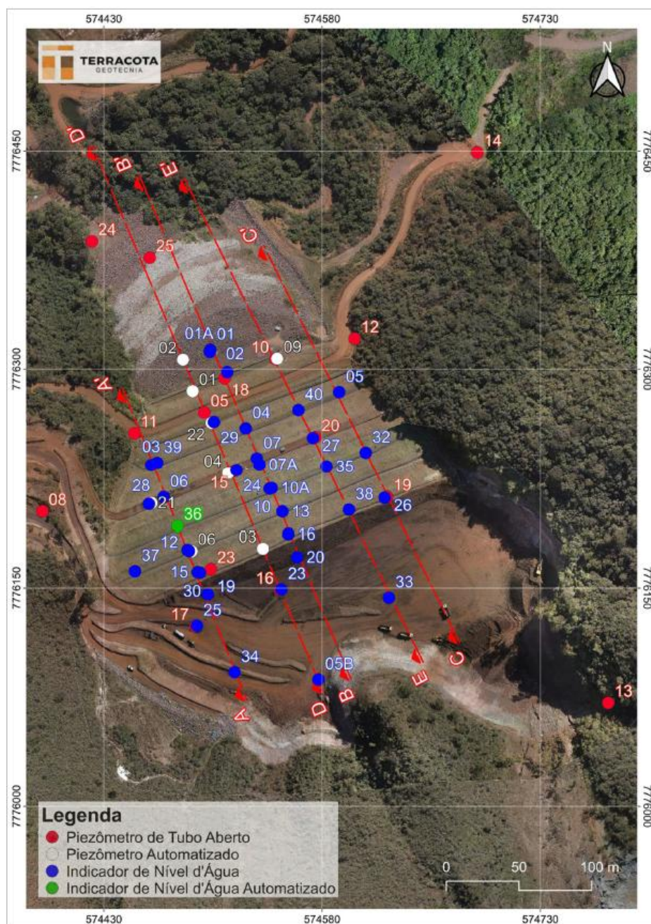
Figura 6.41 – Seções Instrumentadas Barragem B2 – Mina Tico-Tico – Planta.
