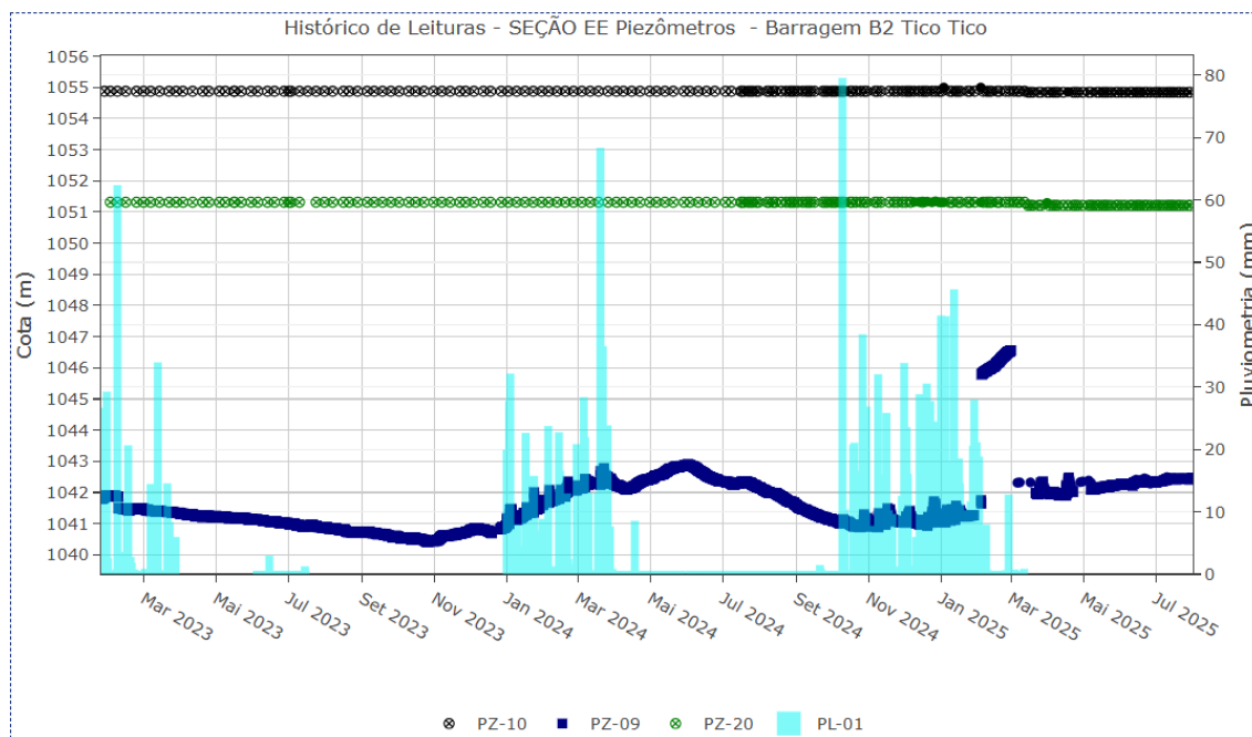
Figura 6.25 - Piezômetros Seção EE
