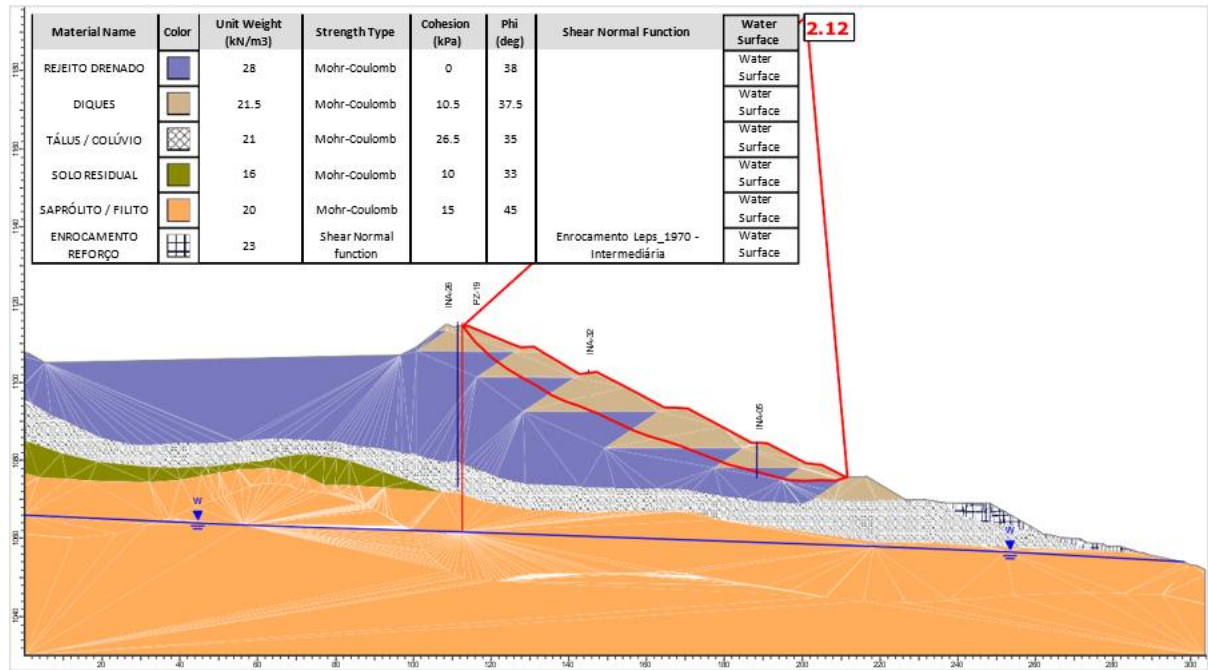
Figura 6.54 – Seção C-C’ – Análise Drenada – Superfície de ruptura plano-circular otimizada – Freática 31/07/2025.
