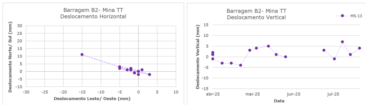
Figura 6.40 – Marco de controle de deformação – MS-13.
