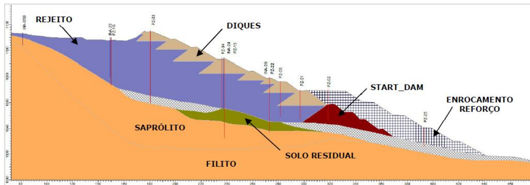
Figura 4.3 – Seção de maior altura (D-D') da Barragem B2 – Mina Tico-Tico (Condição em junho de 2025).
