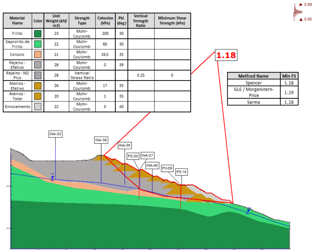
Figura 6.65 – Seção E-E' – Análise Não Drenada – Carregamento Pseudo-Estático sismo ↑
