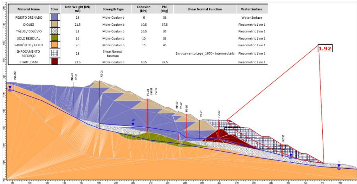
Figura 6.57 – Seção D-D' – Análise Drenada – Superfície de ruptura plano-circular otimizada – Freática 31/07/2025.
