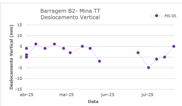
Figura 6.32 – Marco de controle de deformação – MS-05.
