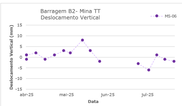
Figura 6.33 – Marco de controle de deformação – MS-06.
