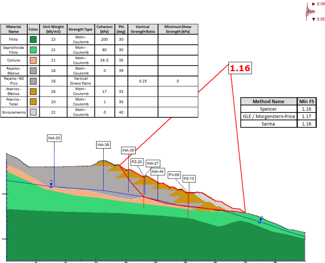
Figura 6.66 – Seção E-E’ – Análise Não Drenada – Carregamento Pseudo-Estático sismo ↓
