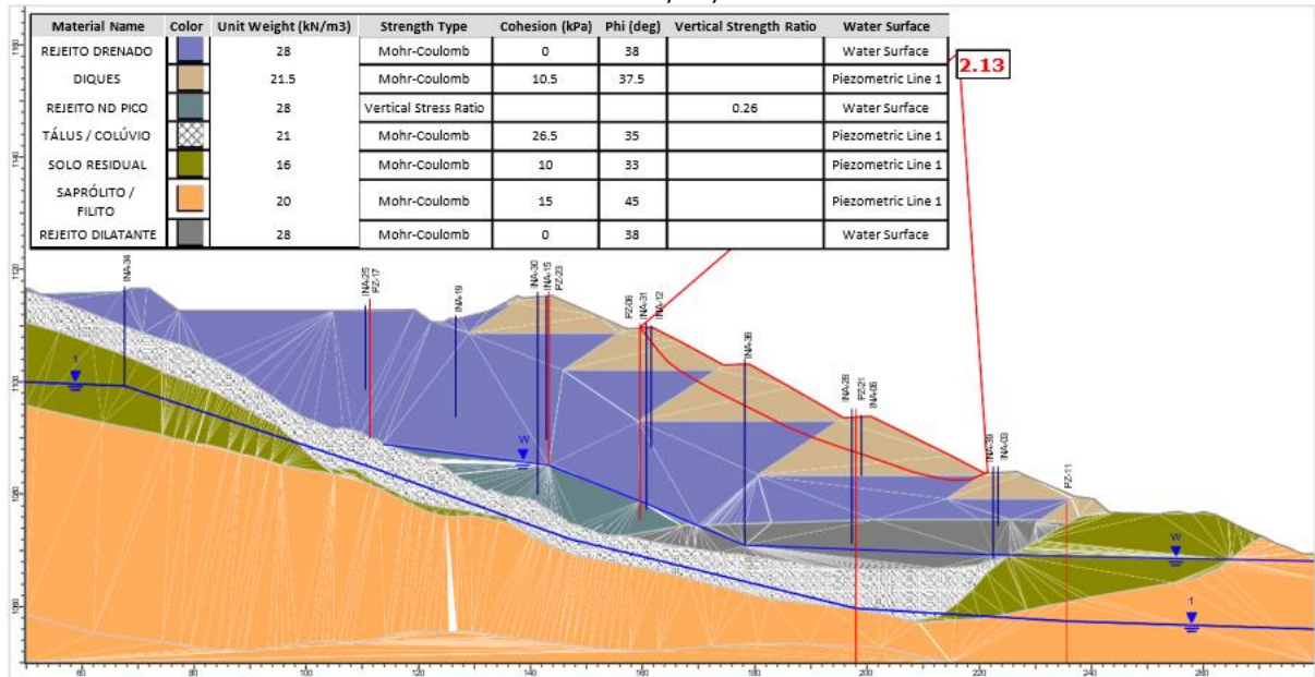
Figura 6.45 – Seção A-A’ – Análise Não Drenada – Superfície de ruptura plano-circular otimizada – Freática 31/07/2025 – Razão de resistência não drenada de pico.
