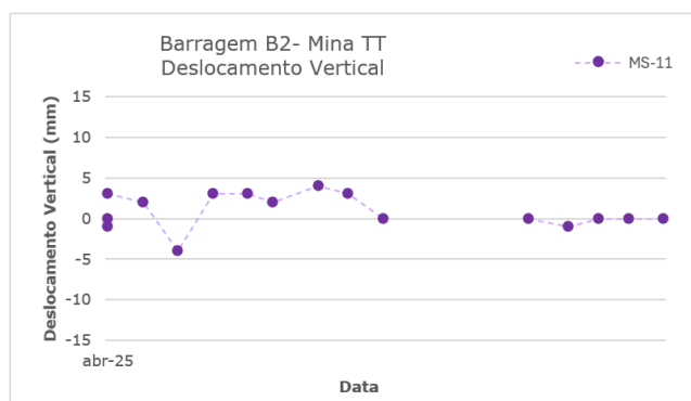
Figura 6.38 – Marco de controle de deformação – MS-11.
