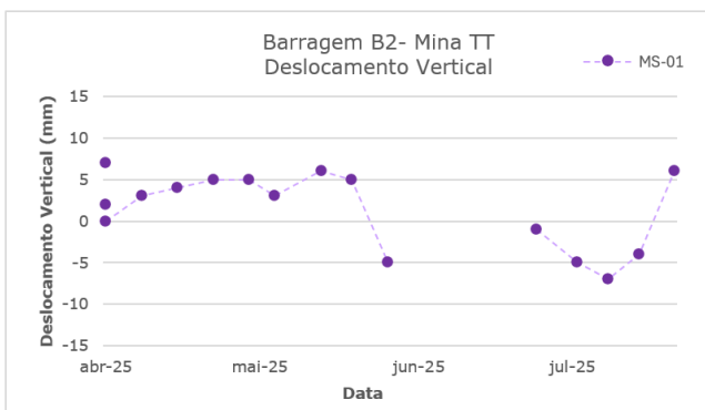
Figura 6.28 – Marco de controle de deformação – MS-01.
