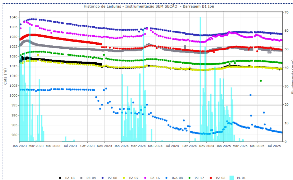
Figura 6.26 - Instrumentos Sem Seção
