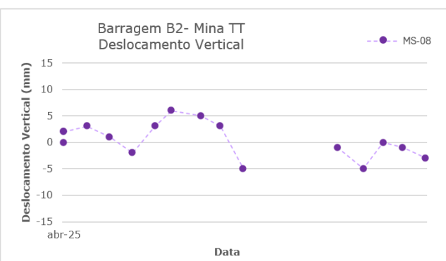
Figura 6.35 – Marco de controle de deformação – MS-08.
