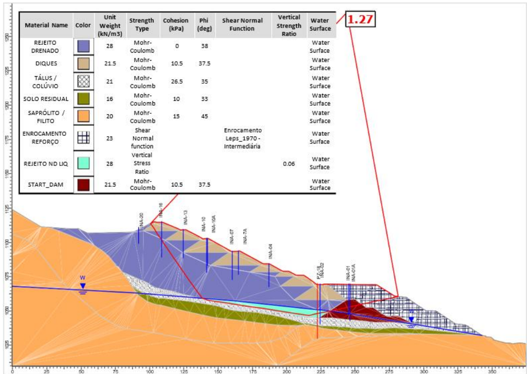
Figura 6.51 – Seção B-B’ – Análise Não Drenada – Superfície de ruptura plano-circular otimizada – Freática 31/07/2025 – Razão de resistência não drenada liquefeita.
