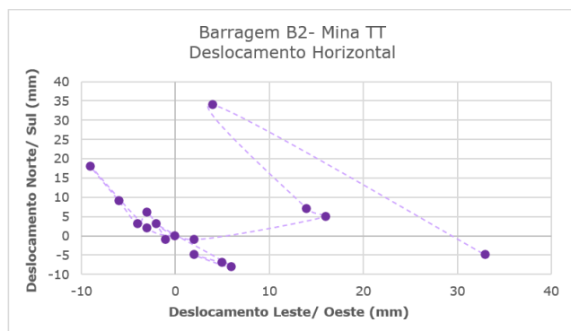
Figura 6.29 – Marco de controle de deformação – MS-02.
