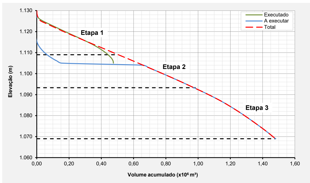
Figura 6.13 – Curva elevação-volume – Comparativo andamento das obras.
