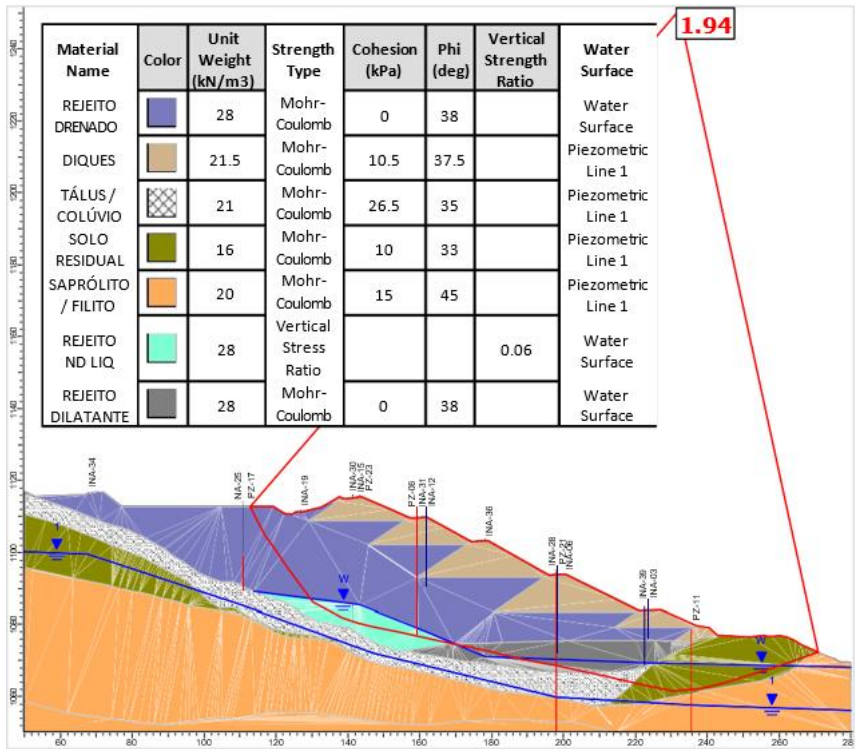
Figura 6.46 – Seção A-A’ – Análise Não Drenada – Superfície de ruptura plano-circular otimizada – Freática 31/07/2025 – Razão de resistência não drenada liquefeita.
