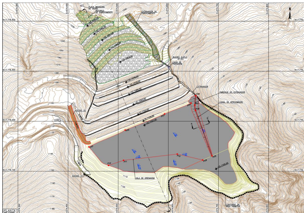
Figura 6.72 - Adequação do novo canal extravasor de emergência
