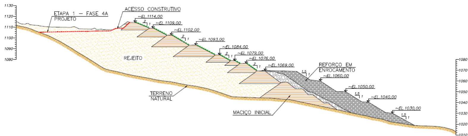
Figura 6.11 – Comparativo Projeto (Etapa 1 - Fase 3A) x Executado – Seção D-D'.
