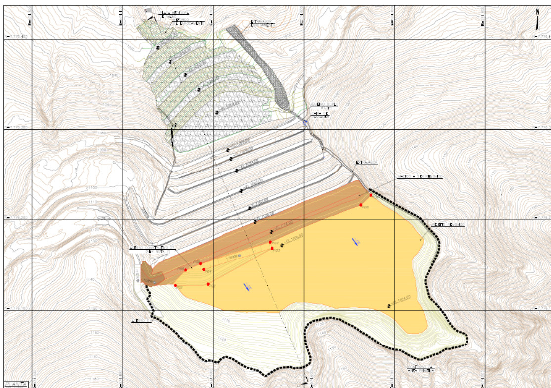
Figura 6.2 - Sequência Construtiva – Planta – Etapa 1- Fase 4A (IPE.OP.DE.8000.GT.20.719)
