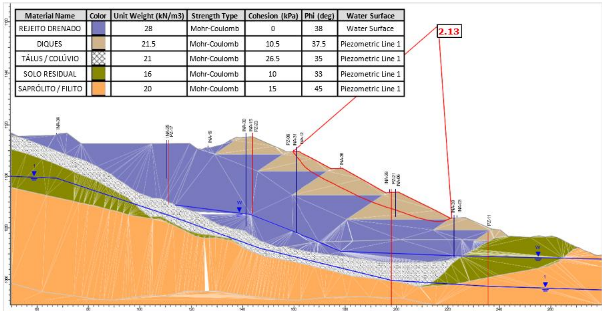
Figura 6.44 – Seção A-A’ – Análise Drenada – Superfície de ruptura plano-circular otimizada – Freática 31/07/2025.
