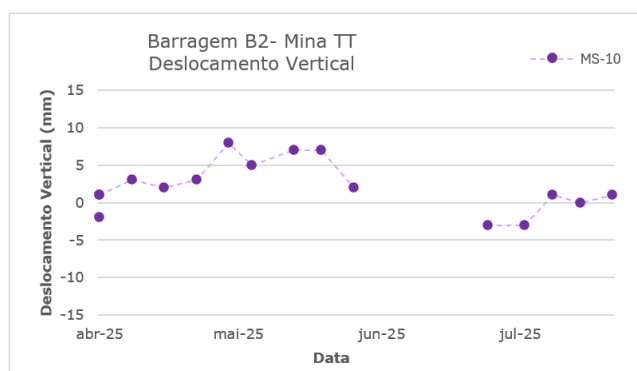
Figura 6.37 – Marco de controle de deformação – MS-10.
