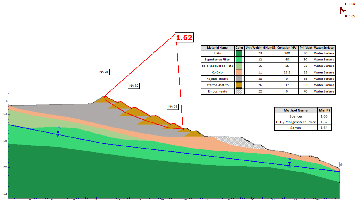
Figura 6.56 – Seção C-C' – Análise Drenada – Carregamento Pseudo-Estático sísmico ↓
