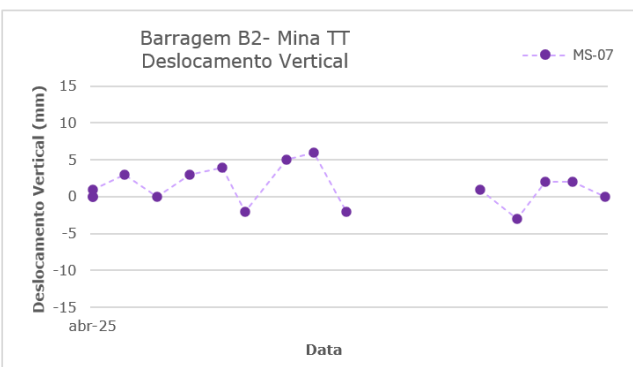
Figura 6.34 – Marco de controle de deformação – MS-07.
