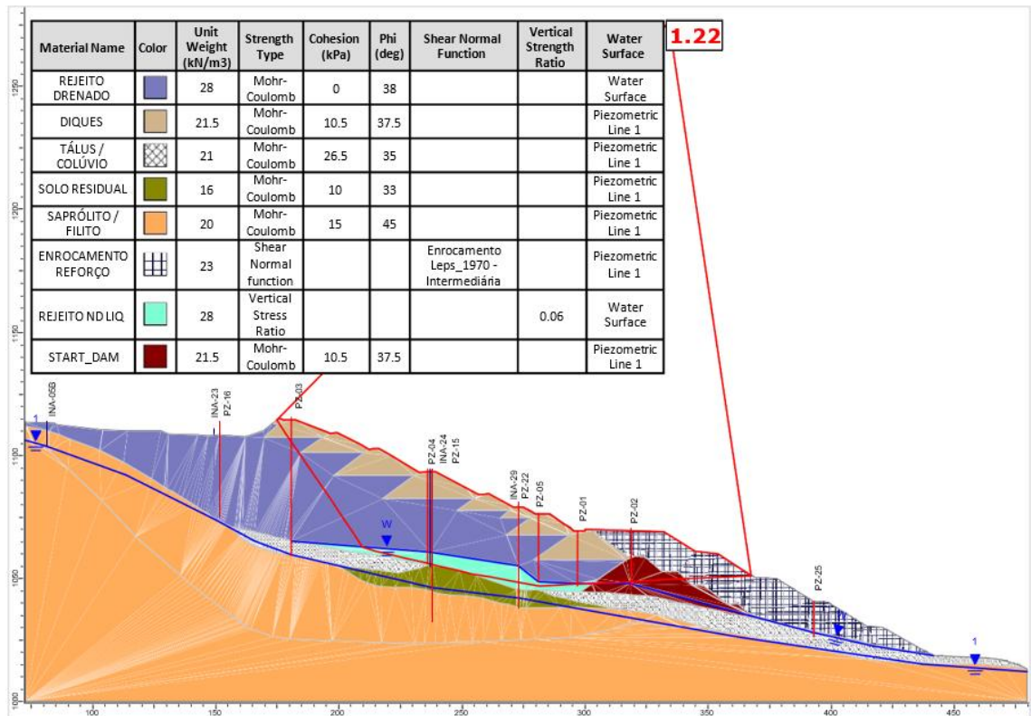
Figura 6.59 – Seção D-D’ – Análise Não Drenada – Superfície de ruptura plano-circular otimizada – Freática 31/07/2025 – Razão de resistência não drenada liquefeita.
