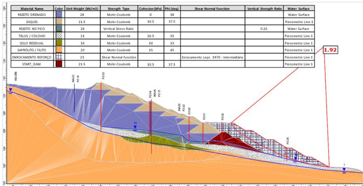
Figura 6.58 – Seção D-D’ – Análise Não Drenada – Superfície de ruptura plano-circular otimizada – Freática 31/07/2025 – Razão de resistência não drenada de pico.
