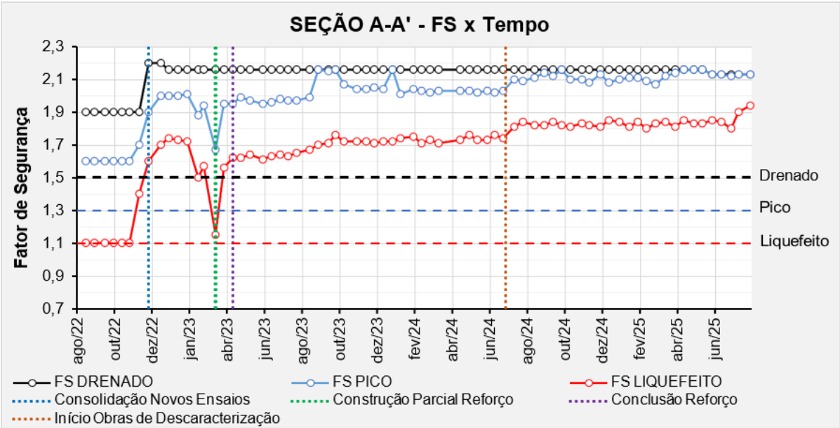
Figura 6.67 – Seção A-A’ - Histórico dos F.S. obtidos nas análises de estabilidade.
