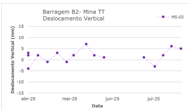
Figura 6.30 – Marco de controle de deformação – MS-03.
