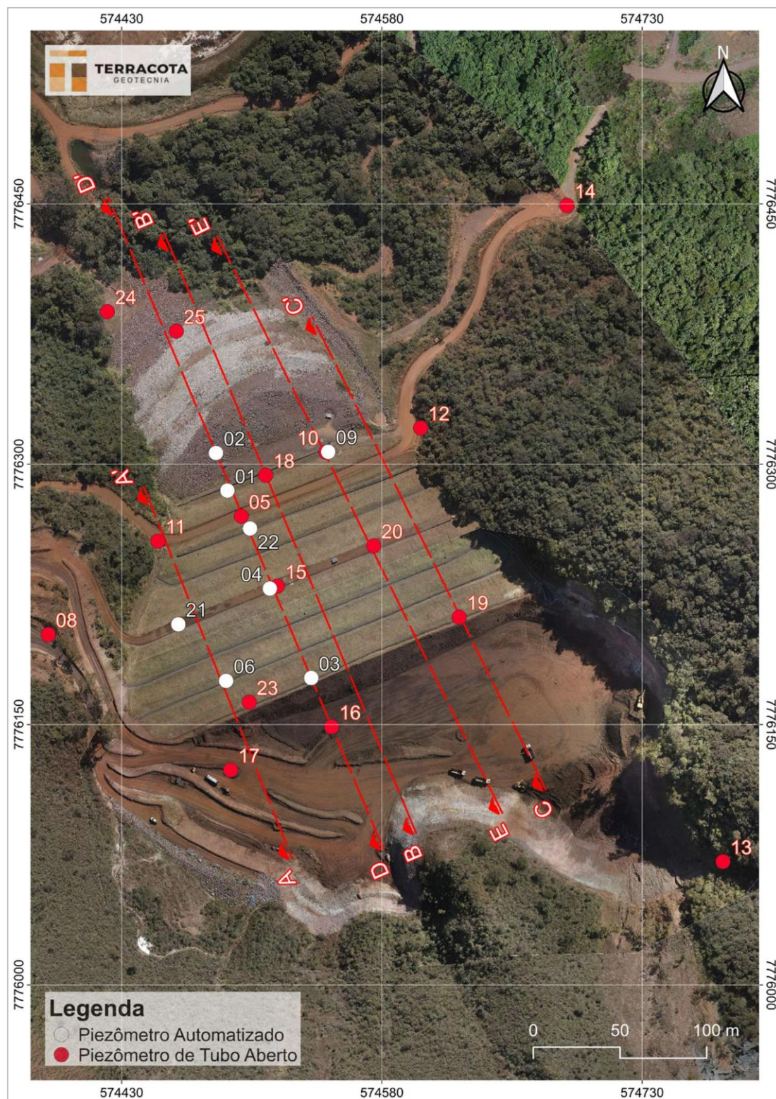
Figura 6.15 – Localização dos piezômetros.
