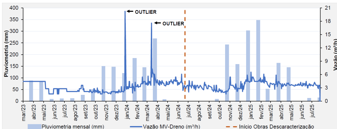
Figura 6.27 – Vazão – MV-Dreno – Barragem B2 – Mina Tico-Tico.
