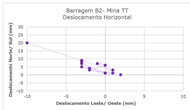
Figura 6.36 – Marco de controle de deformação – MS-09.
