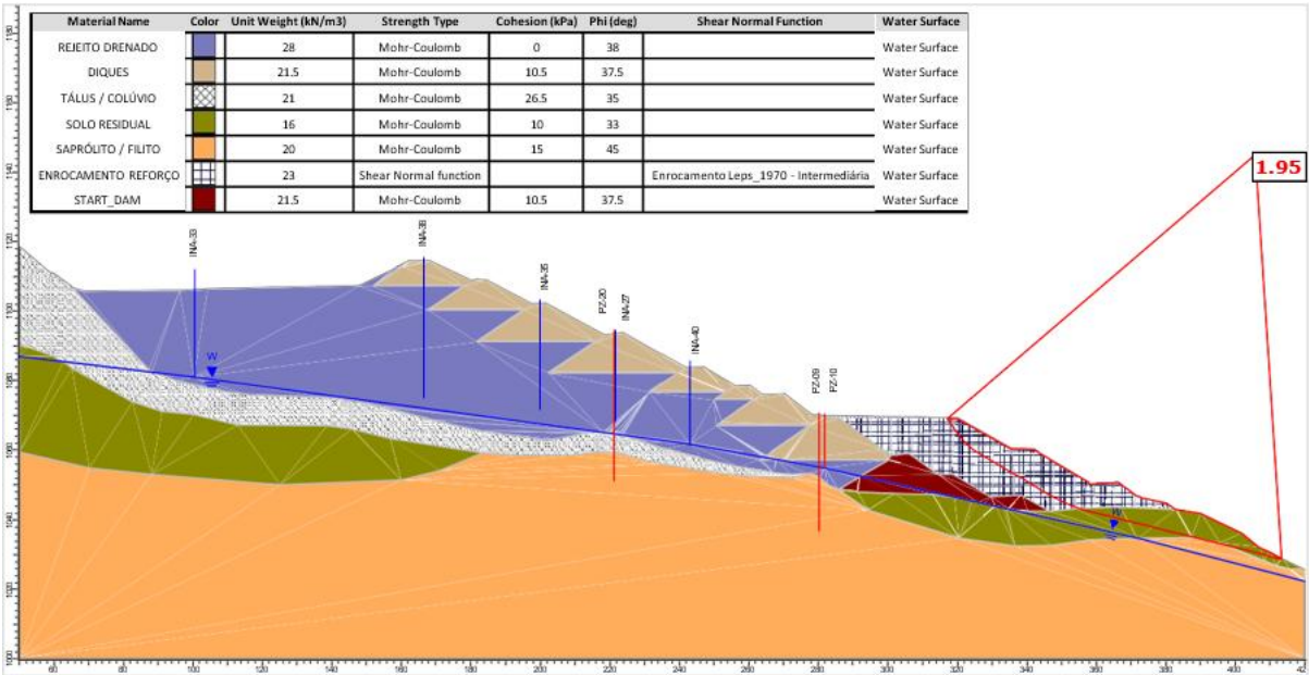
Figura 6.62 – Seção E-E’ – Análise Drenada – Superfície de ruptura plano-circular otimizada – Freática 31/07/2025.
