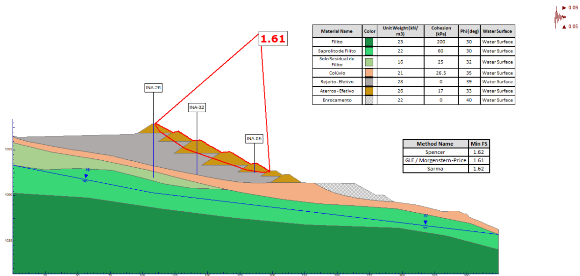
Figura 6.55 – Seção C-C’ – Análise Drenada – Carregamento Pseudo-Estático sísmico ↑
