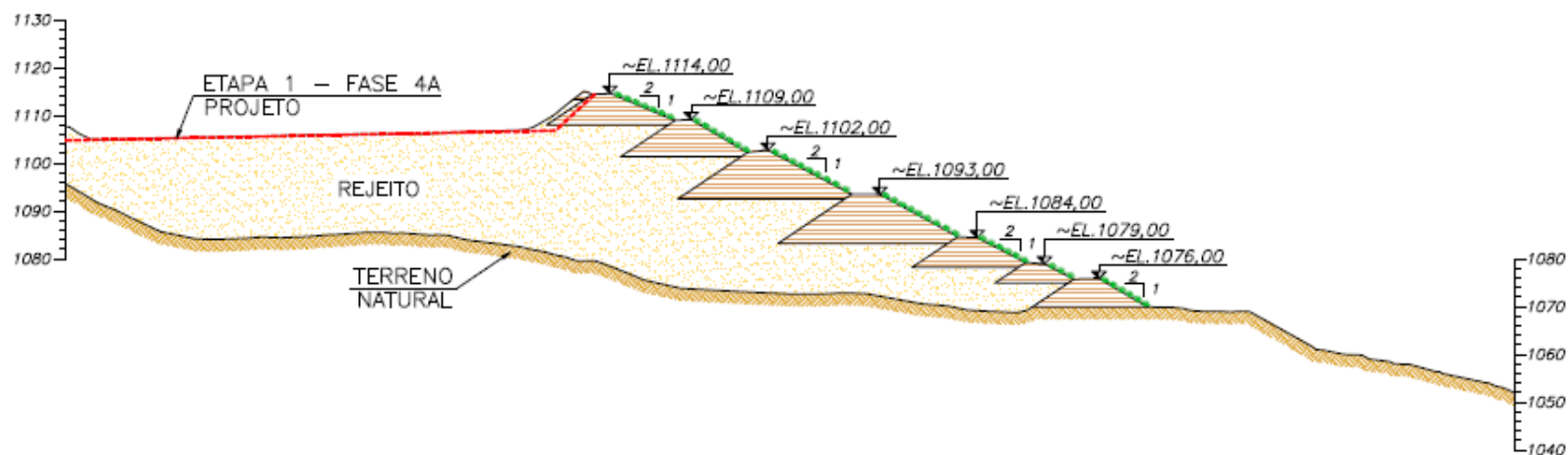
Figura 6.10 – Comparativo Projeto (Etapa 1 - Fase 3A) x Executado – Seção C-C'.
