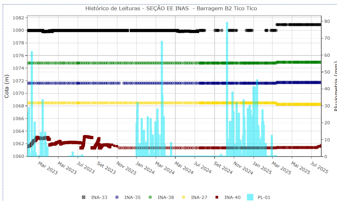
Figura 6.24 - INAS Seção EE
