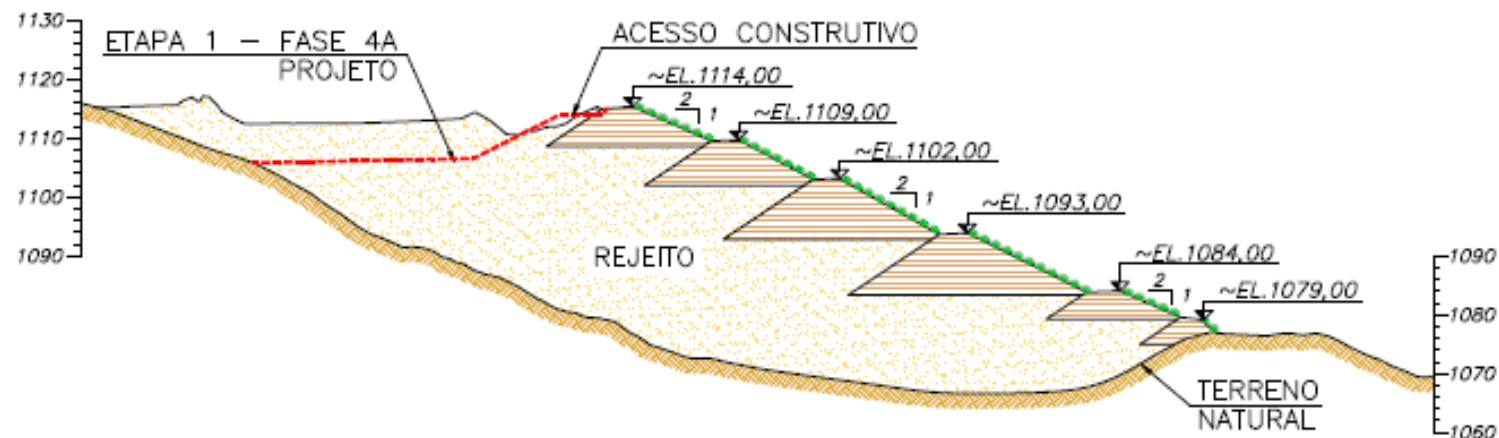
Figura 6.8 – Comparativo Projeto (Etapa 1 - Fase 4A) x Executado – Seção A-A'.
