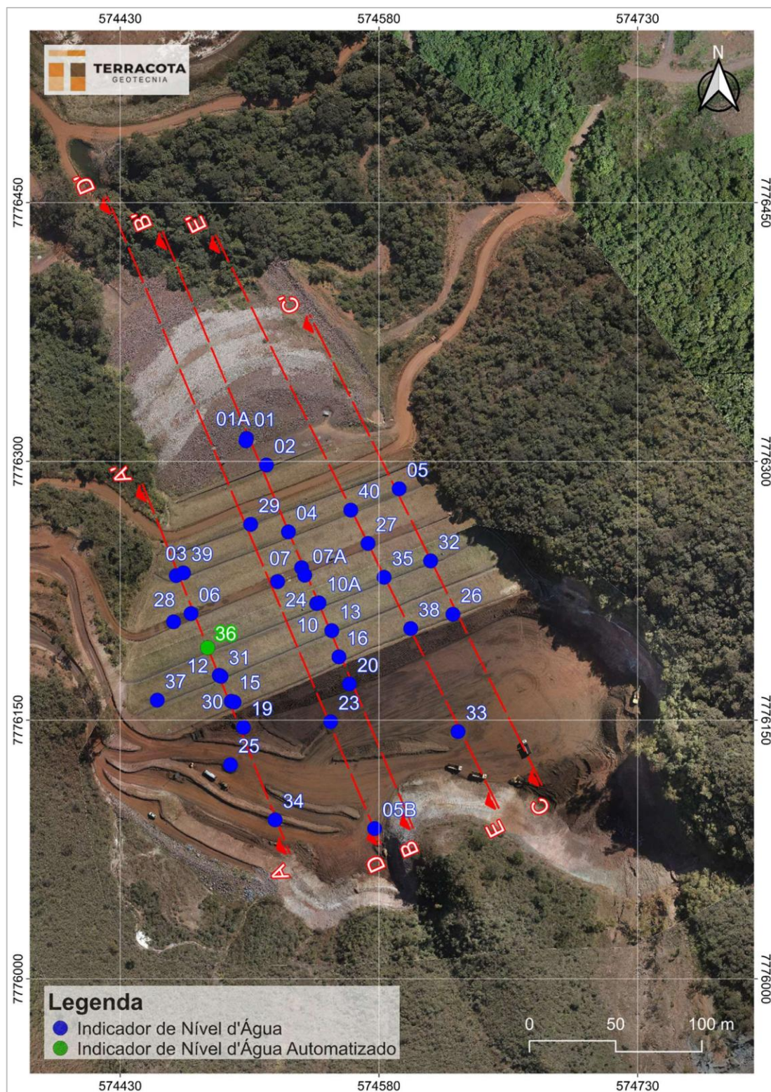
Figura 6.14 – Localização dos indicadores de nível d'água.
