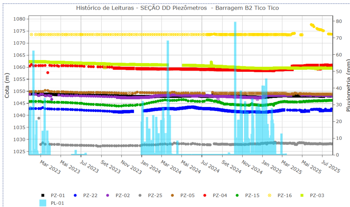
Figura 6.23 - Piezômetros Seção DD
