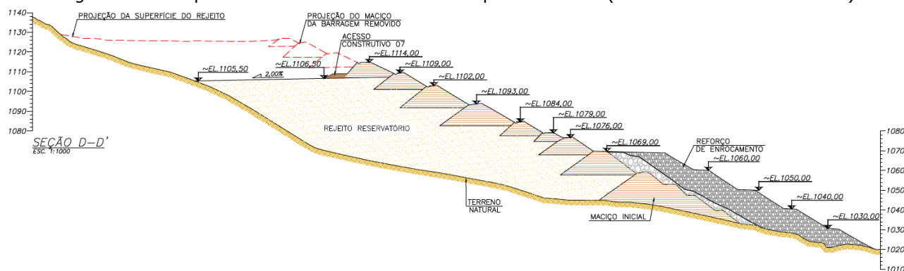
Figura 6.3 - Sequência Construtiva – Seção D-D' – Etapa 1 - Fase 4A (IPE.OP.DE.8000.GT.20.719)
