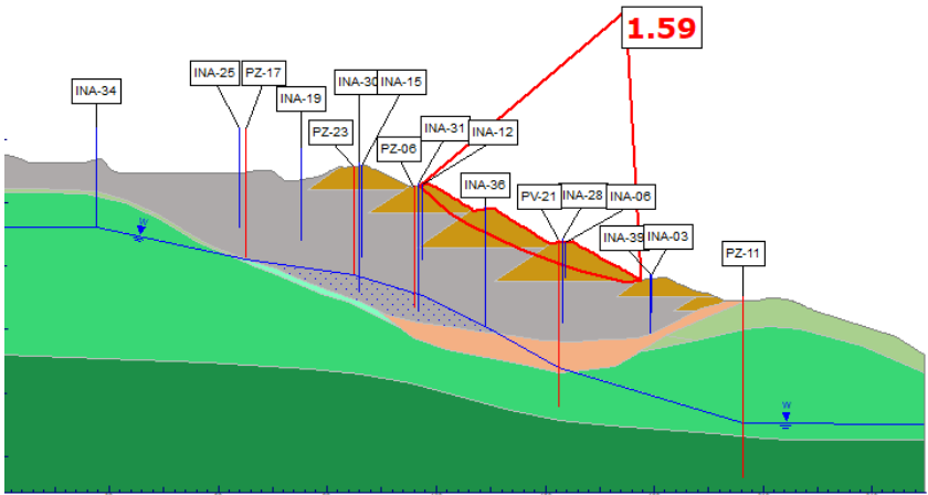
Figura 6.48 – Seção A-A’ – Análise Não Drenada – Carregamento Pseudo-Estático sismo ↓
