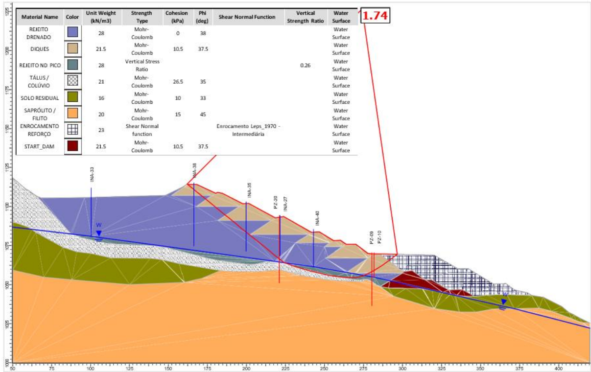
Figura 6.63 – Seção E-E’ – Análise Não Drenada – Superfície de ruptura plano-circular otimizada – Freática 31/07/2025 – Razão de resistência não drenada de pico.
