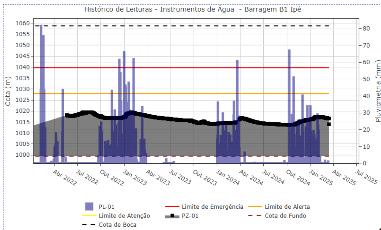
Figura 5.32 – Desempenho do piezômetro automatizado selado – PZ-01.
