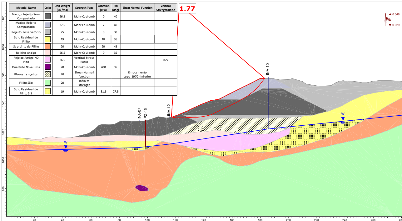
Figura 5.105 – Seção C-C’ – Análise Não Drenada – Superfície de ruptura plano-circular otimizada – Freática 30/07/2025 – Razão de resistência não drenada de pico + sismo ↓ (critério vida útil).
