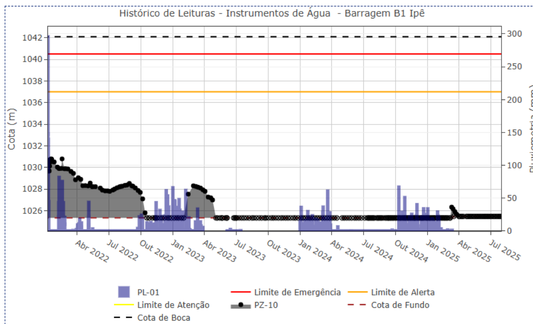
Figura 5.41 – Desempenho do piezômetro de tubo aberto – PZ-10.
