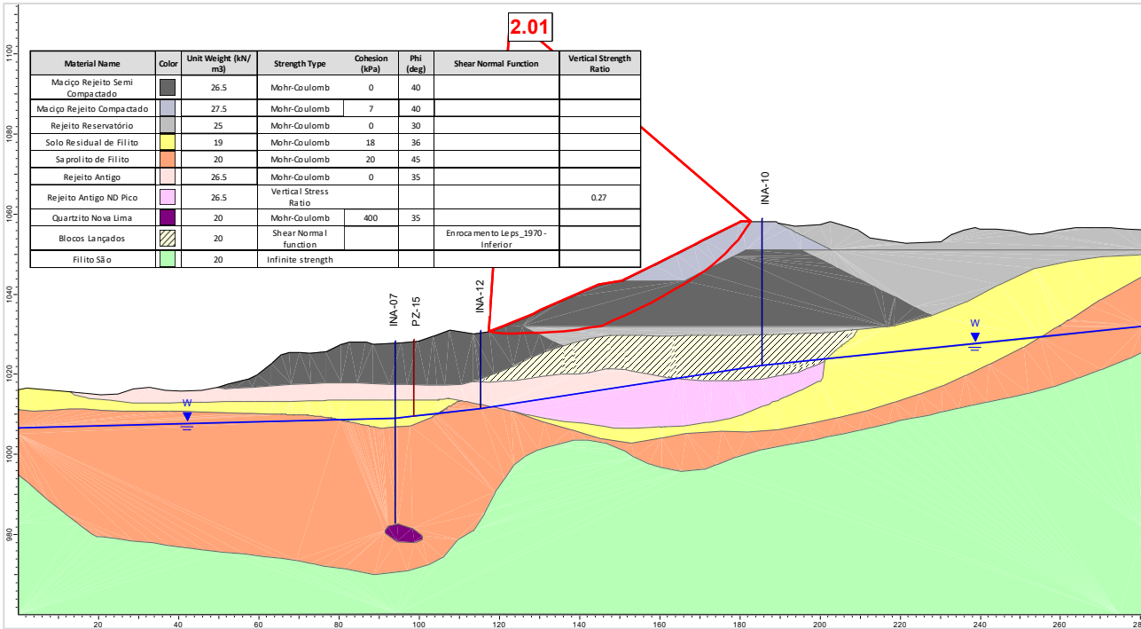
Figura 5.100 – Seção C-C’ – Análise Não Drenada – Superfície de ruptura plano-circular otimizada – Freática 30/07/2025 – Razão de resistência não drenada de pico.
