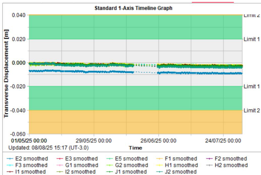
Figura 5.57 – Registros parciais das leituras dos prismas – Transverse Displacement. (ref: 01/05/25 a 31/07/25)
