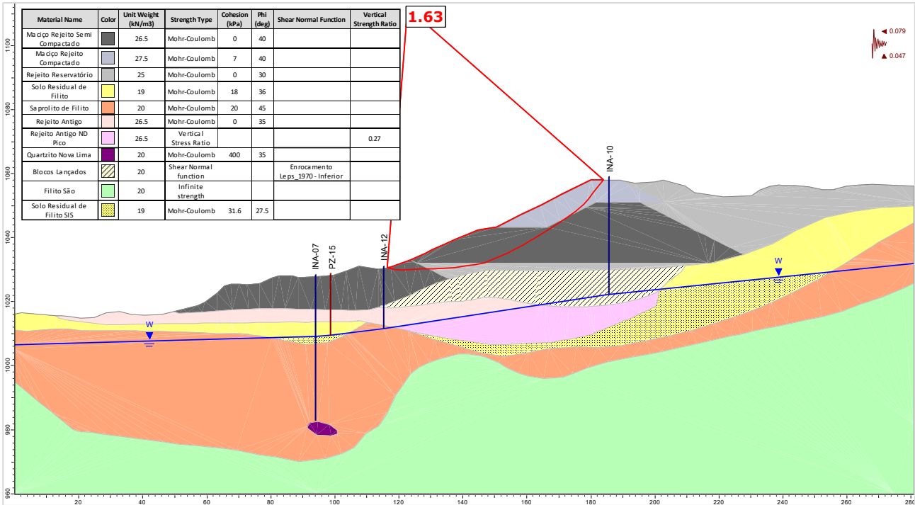
Figura 5.102 – Seção C-C’ – Análise Não Drenada – Superfície de ruptura plano-circular otimizada – Freática 30/07/2025 – Razão de resistência não drenada de pico + sismo ↑ (critério CDA).
