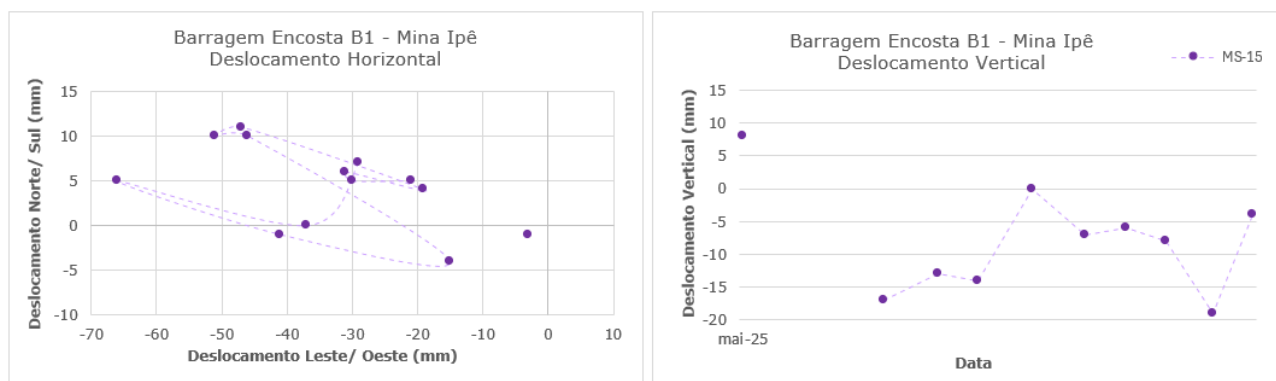
Figura 5.78 – Prisma de monitoramento da encosta MS-15.
