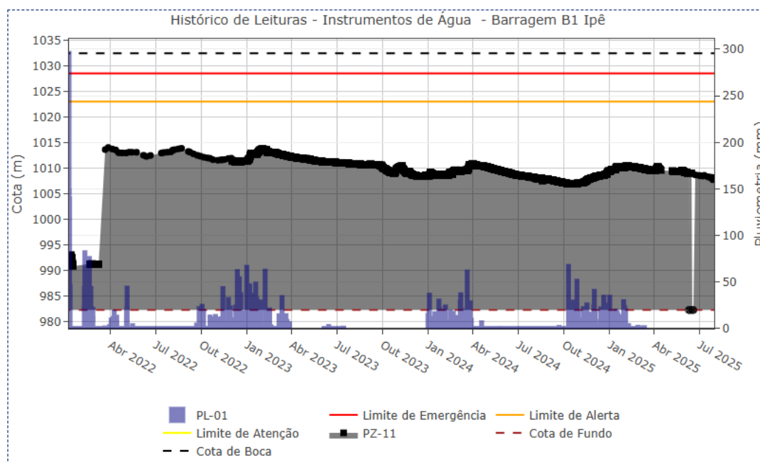
Figura 5.42 – Desempenho do piezômetro automatizado – PZ-11.
