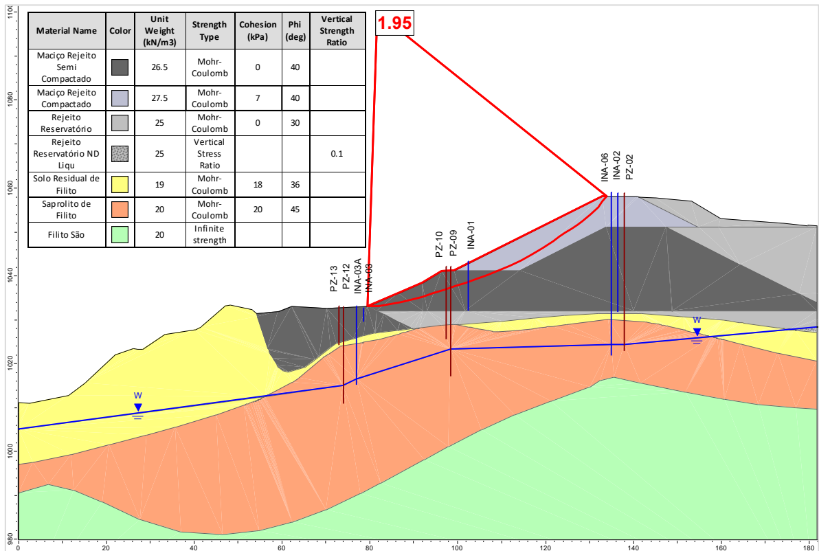
Figura 5.87 – Seção A-A' – Análise Não Drenada – Superfície de ruptura plano-circular otimizada – Freática 30/07/2025 – Razão de resistência não drenada liquefeito.
