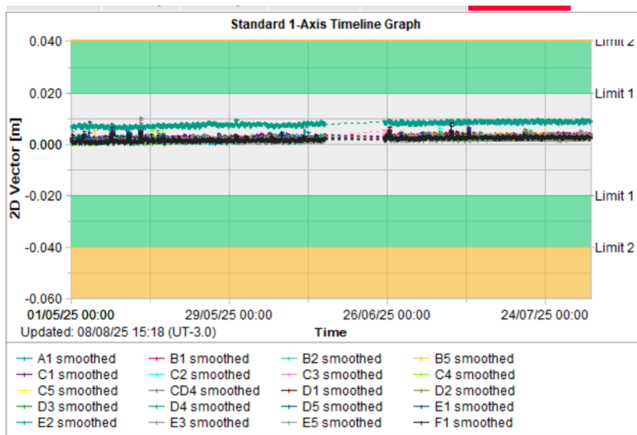
Figura 5.58 – Registros parciais das leituras dos prismas – 2D Vector. (ref: 01/05/25 a 31/07/25)
