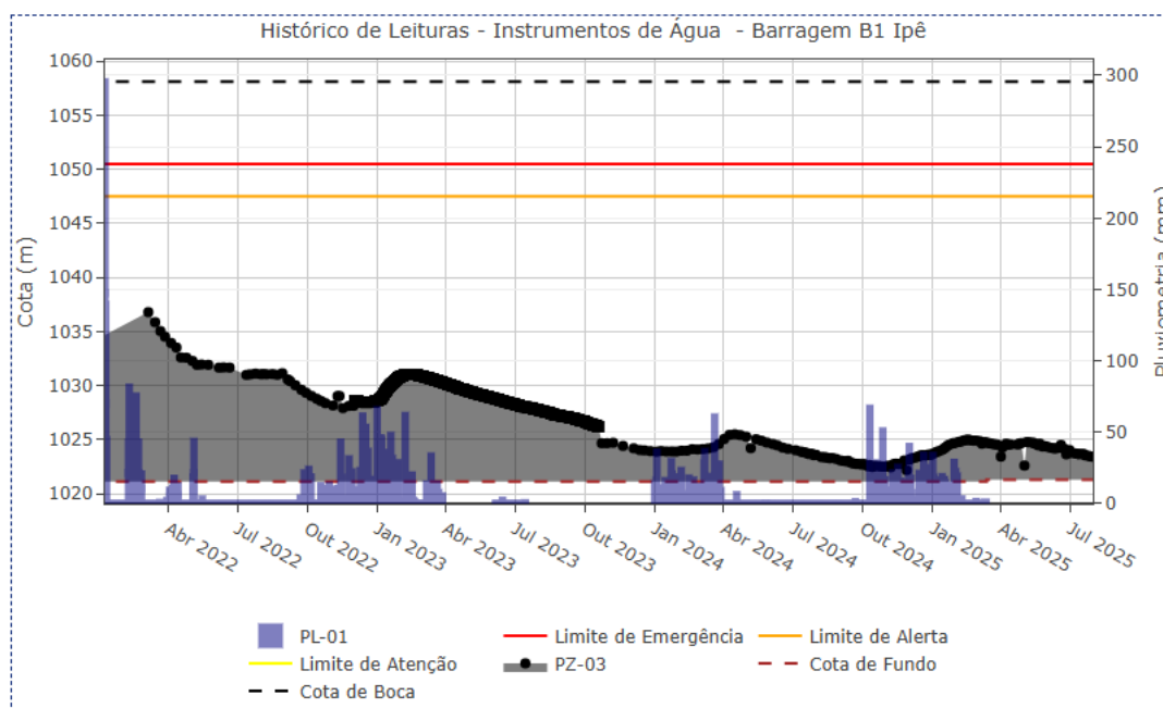
Figura 5.34 – Desempenho do piezômetro de tubo aberto – PZ-03.
