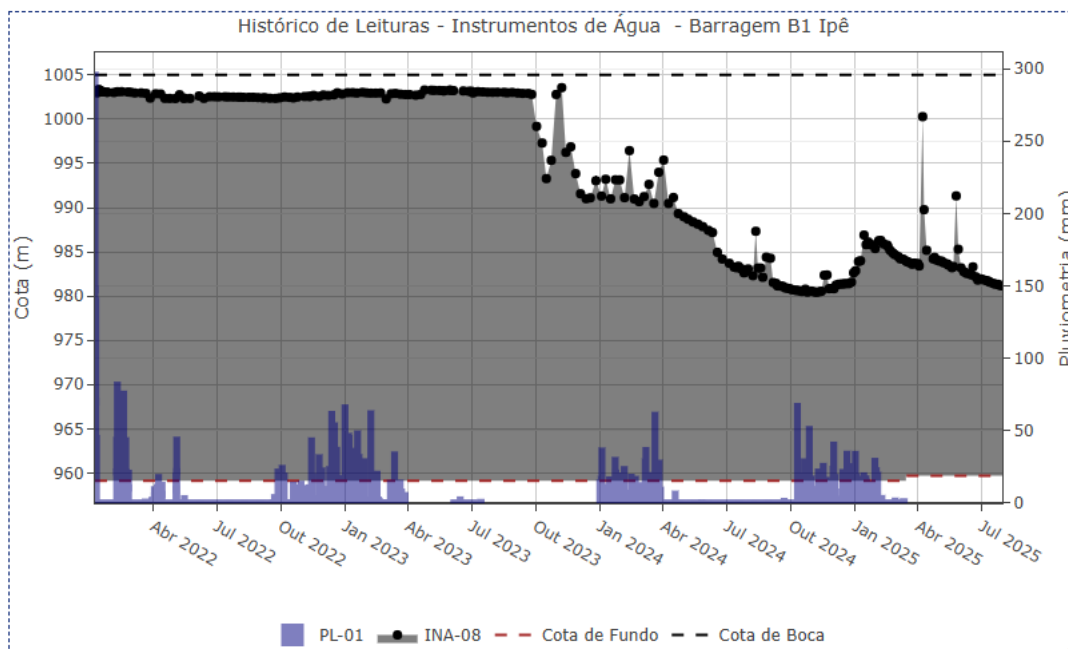
Figura 5.25 – Desempenho do indicador de nível d'água – INA-08.
