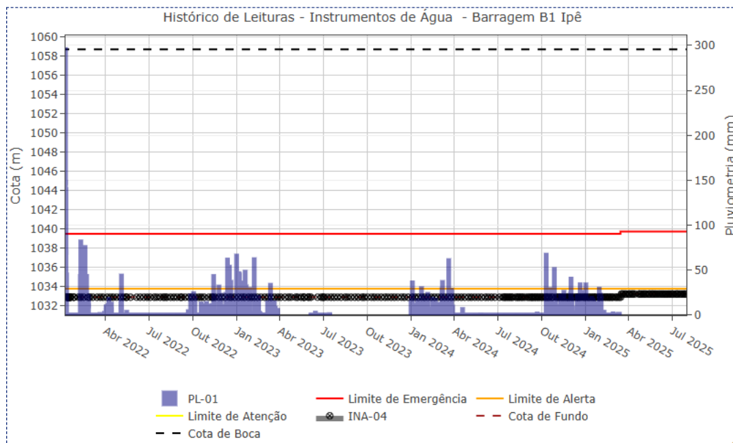
Figura 5.21 – Desempenho do indicador de nível d'água – INA-04.
