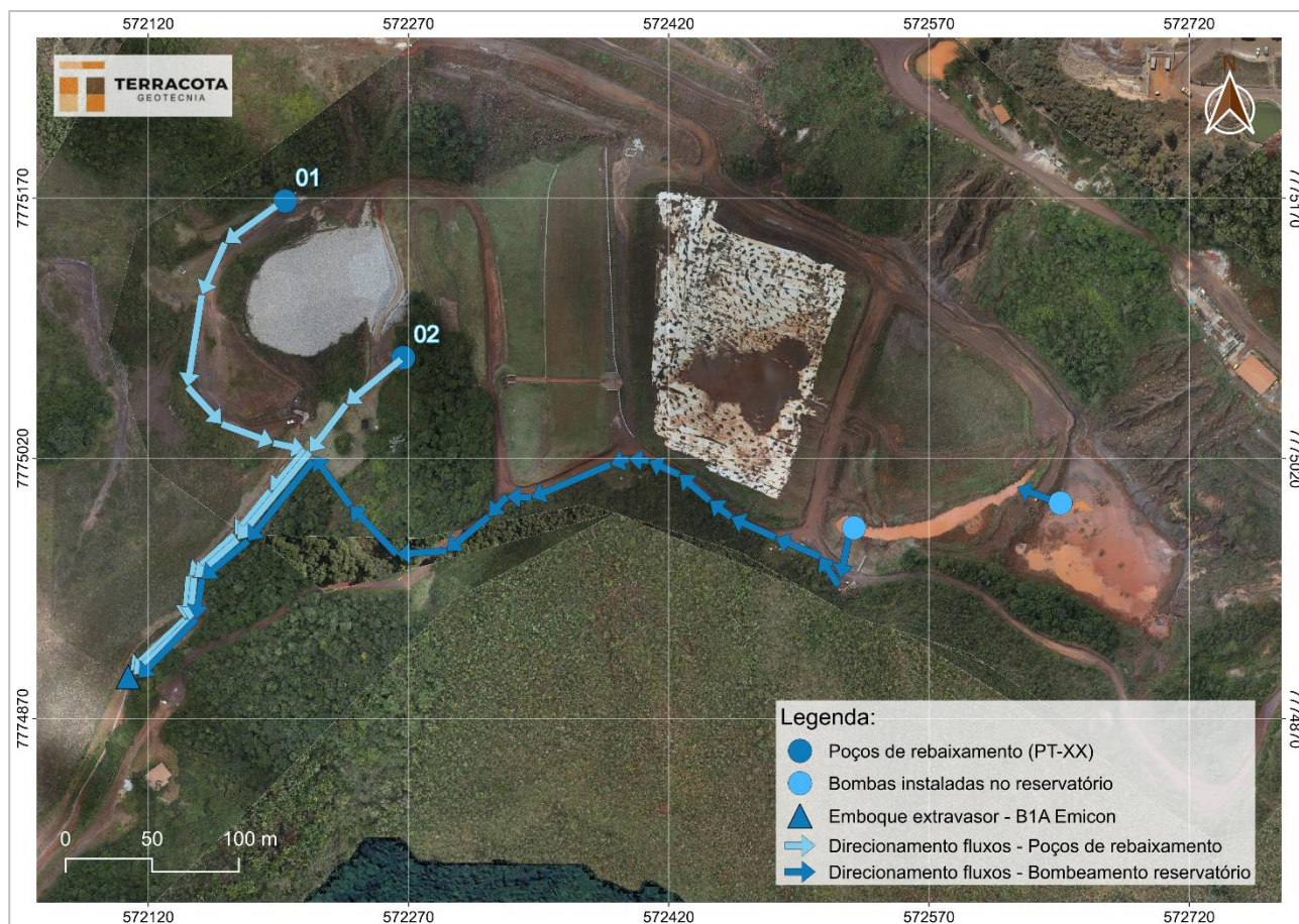
Figura 5.80 – Esquema de direcionamento atual dos fluxos proveniente dos sistemas de bombeamento.
