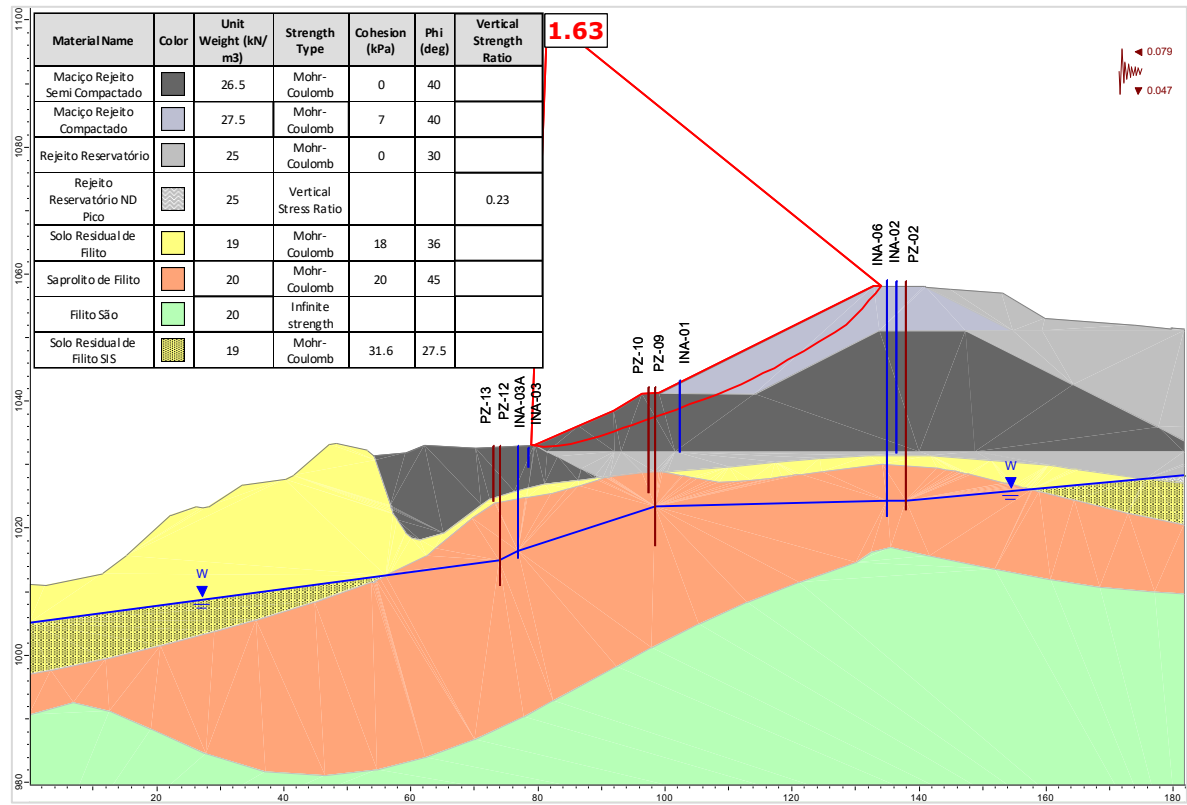
Figura 5.89 – Seção A-A’ – Análise Não Drenada – Superfície de ruptura plano-circular otimizada – Freática 30/07/2025 – Razão de resistência não drenada de pico + sismo ↓ (critério CDA).
