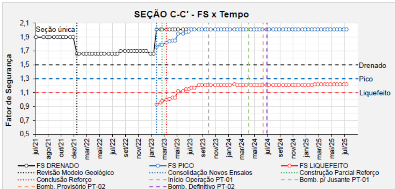
Figura 5.108 – Seção C-C' - Histórico dos F.S. obtidos nas análises de estabilidade.
