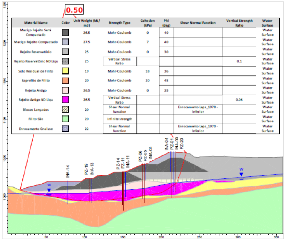
Figura 5.94 – Seção B-B’ – Análise Não Drenada – Superfície de ruptura plano-circular otimizada – Freática 30/07/2025 – Razão de resistência não drenada liquefeito.
