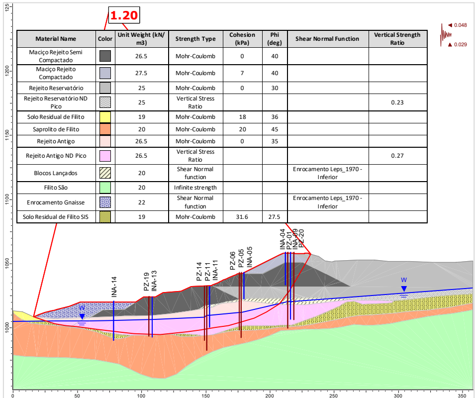
Figura 5.97 – Seção B-B’ – Análise Não Drenada – Superfície de ruptura plano-circular otimizada –
