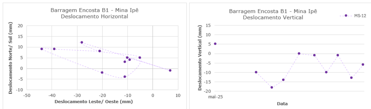
Figura 5.75 – Prisma de monitoramento da encosta MS-12.
