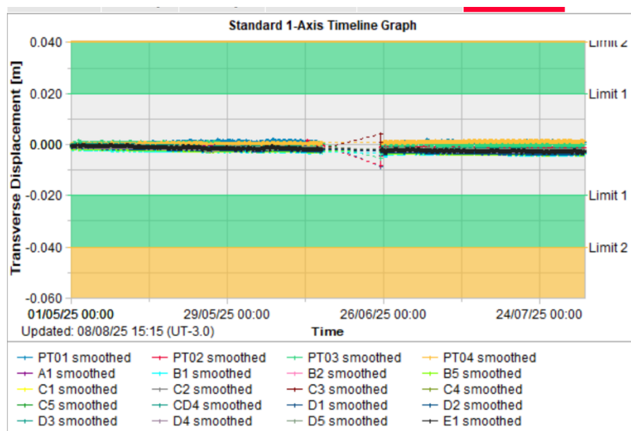
Figura 5.56 – Registros parciais das leituras dos prismas – Transverse Displacement. (ref: 01/05/25 a 31/07/25)
