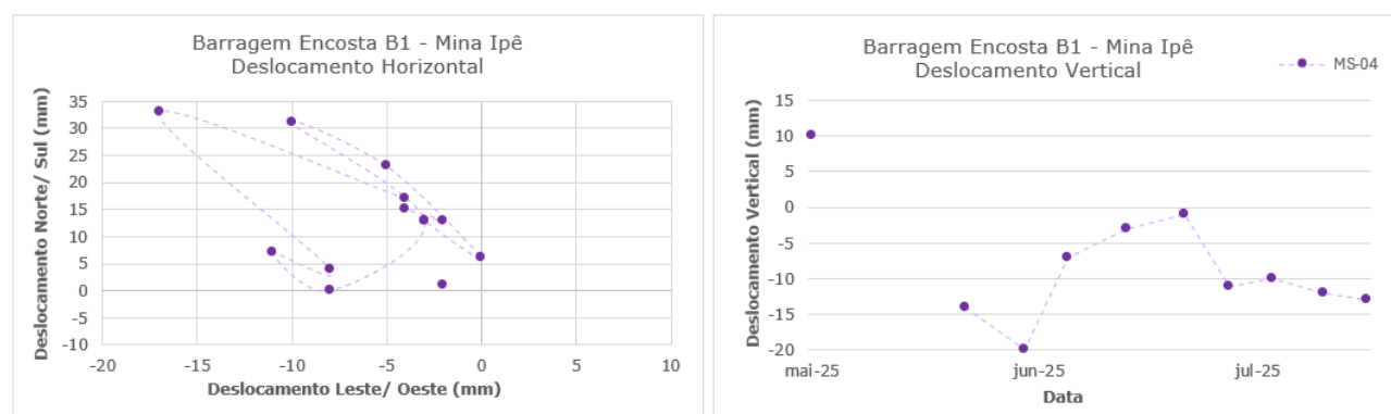
Figura 5.67 – Prisma de monitoramento da encosta MS-04.
