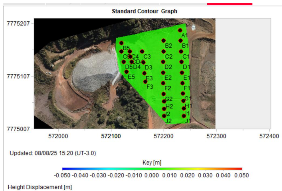
Figura 5.54 – Registros deslocamentos verticais dos prismas. (ref: 01/05/25 a 31/07/25)
