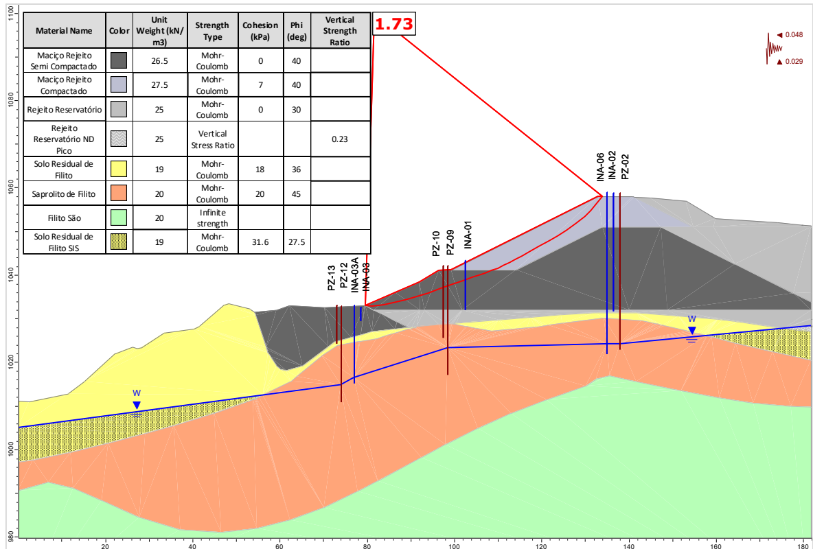
Figura 5.90 – Seção A-A’ – Análise Não Drenada – Superfície de ruptura plano-circular otimizada – Freática 30/07/2025 – Razão de resistência não drenada de pico + sismo ↑ (critério vida útil).
