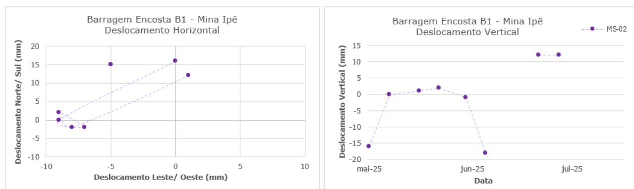
Figura 5.65 – Prisma de monitoramento da encosta MS-02.
