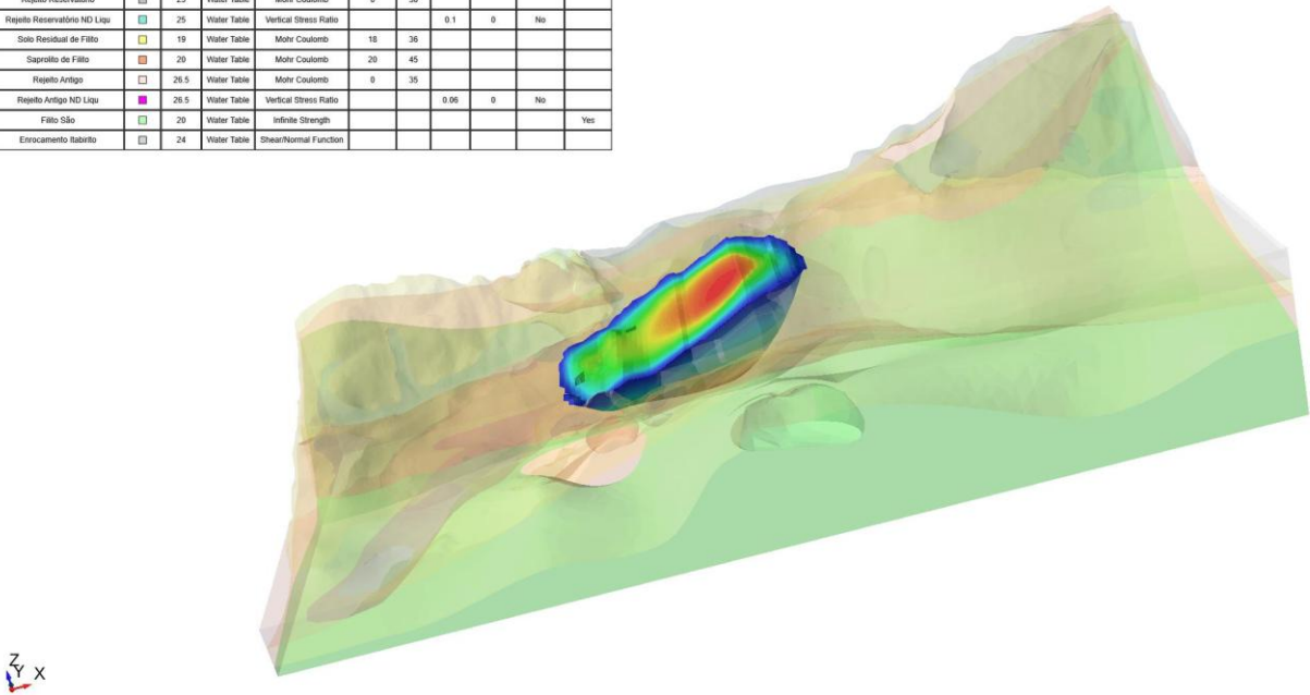
Figura 5.110 – Análise de estabilidade 3D – Rejeitos saturados na condição liquefeita - Vista do mapa de profundidade da superfície de ruptura crítica.
