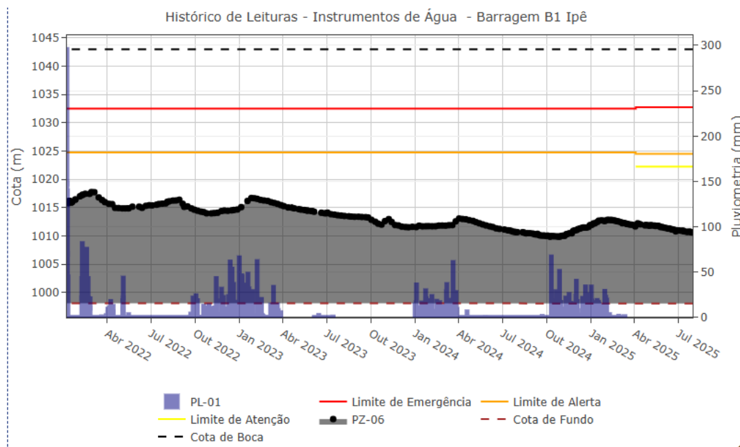
Figura 5.37 – Desempenho do piezômetro de tubo aberto – PZ-06.
