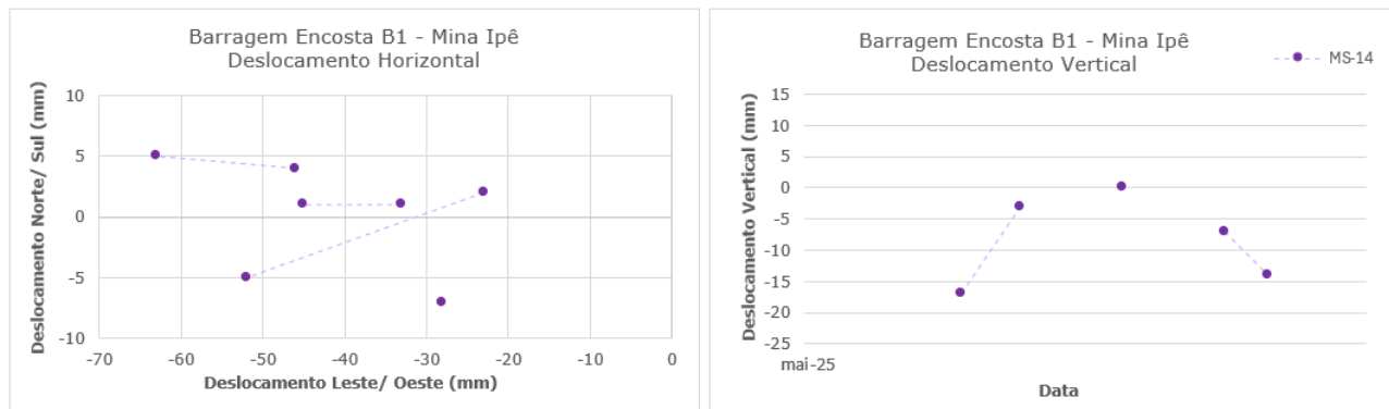
Figura 5.77 – Prisma de monitoramento da encosta MS-14.
