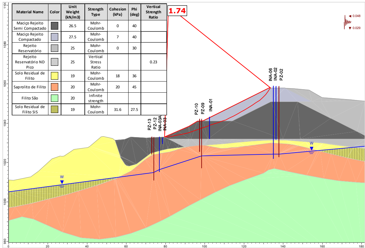
Figura 5.91 – Seção A-A’ – Análise Não Drenada – Superfície de ruptura plano-circular otimizada – Freática 30/07/2025 – Razão de resistência não drenada de pico + sismo ↓ (critério vida útil).
