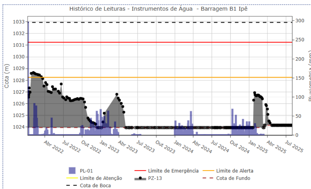
Figura 5.44 – Desempenho do piezômetro de tubo aberto – PZ-13.
