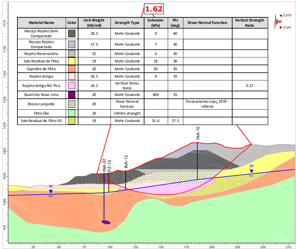
Figura 5.103 – Seção C-C’ – Análise Não Drenada – Superfície de ruptura plano-circular otimizada – Freática 30/07/2025 – Razão de resistência não drenada de pico + sismo ↓ (critério CDA).
