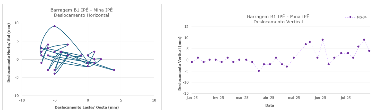
Figura 5.63 – Marco de controle de deformação – MS-04.
