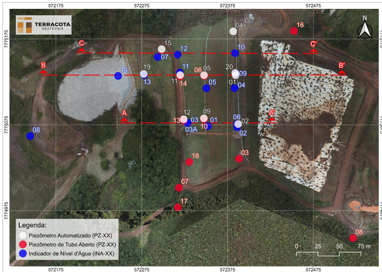
Figura 5.82 – Seções Instrumentadas Barragem B1 – Mina Ipê – Planta.
