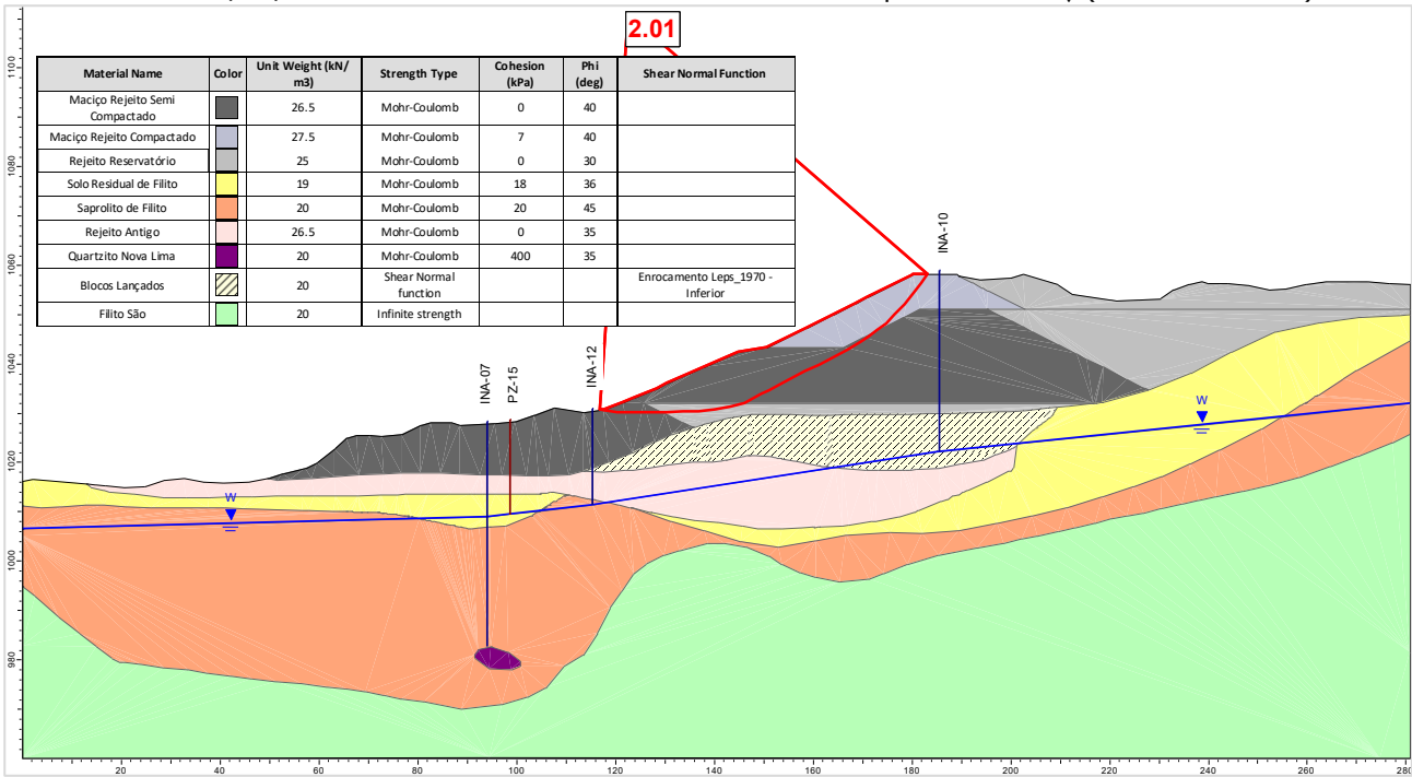
Figura 5.99 – Seção C-C' – Análise Drenada – Superfície de ruptura plano-circular otimizada – Freática 30/07/2025.
