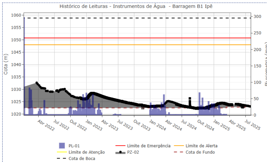
Figura 5.33 – Desempenho do piezômetro automatizado – PZ-02.
