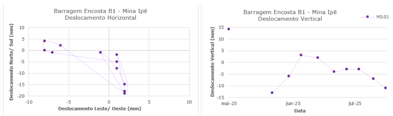
Figura 5.64 – Prisma de monitoramento da encosta MS-01.
