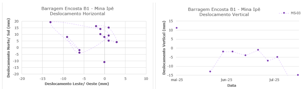
Figura 5.66 – Prisma de monitoramento da encosta MS-03.
