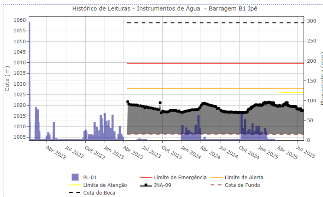
Figura 5.26 – Desempenho do indicador de nível d'água – INA-09.
