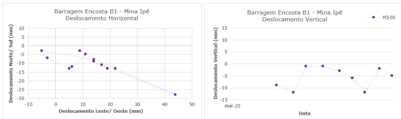
Figura 5.72 – Prisma de monitoramento da encosta MS-09.
