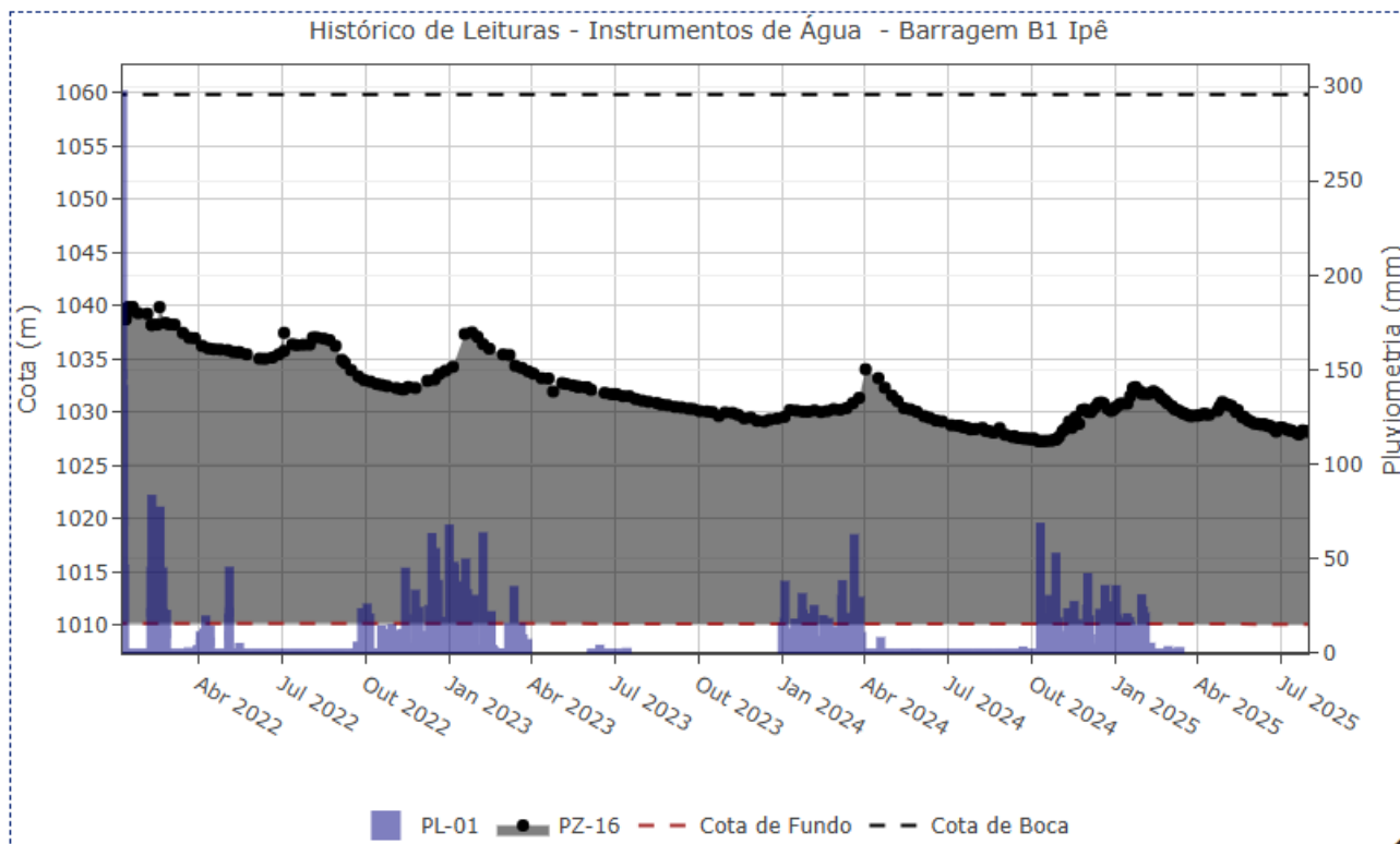
Figura 5.47 – Desempenho do piezômetro de tubo aberto – PZ-16.
