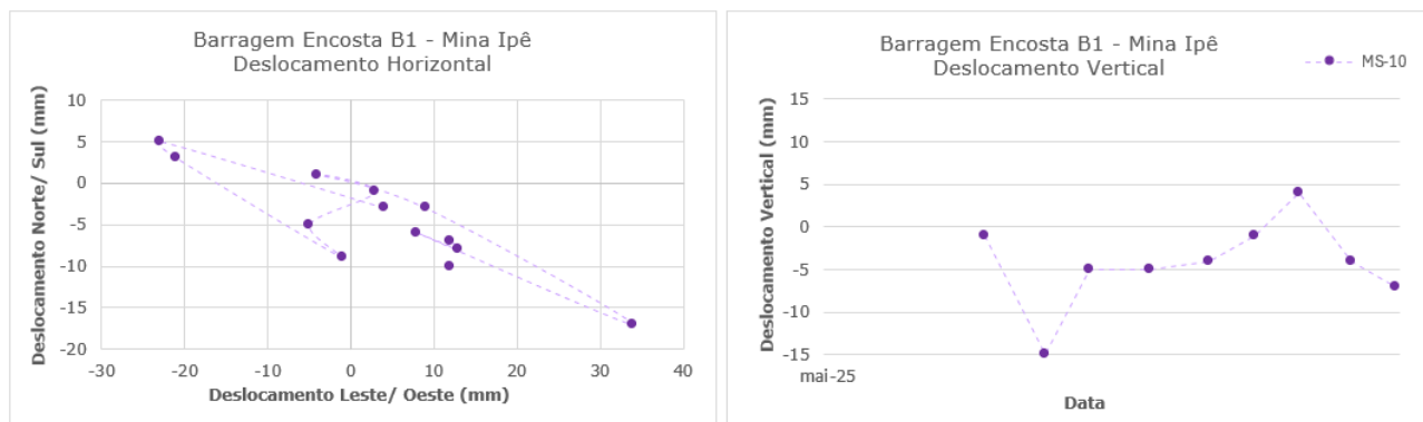
Figura 5.73 – Prisma de monitoramento da encosta MS-10.
