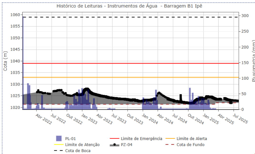
Figura 5.35 – Desempenho do piezômetro automatizado – PZ-04.
