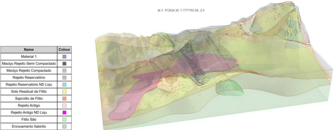
Figura 5.109 – Modelo 3D da Barragem B1 – Mina Ipê no software Slide3.
