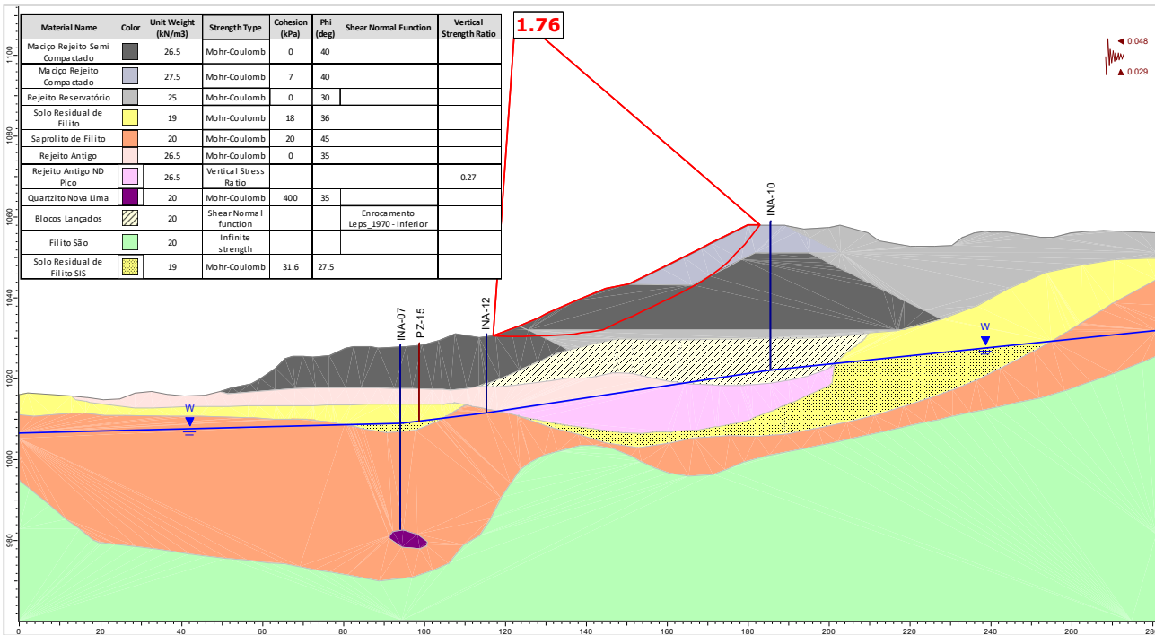
Figura 5.104 – Seção C-C’ – Análise Não Drenada – Superfície de ruptura plano-circular otimizada – Freática 30/07/2025 – Razão de resistência não drenada de pico + sismo ↑ (critério vida útil).
