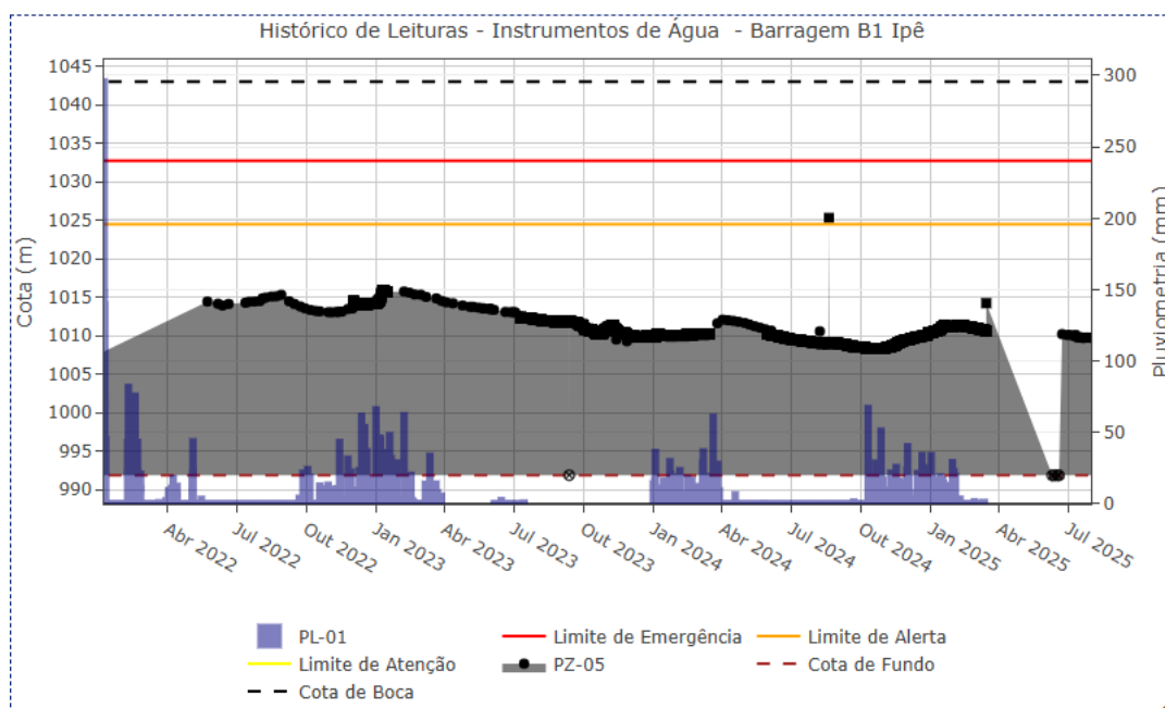
Figura 5.36 – Desempenho do piezômetro automatizado – PZ-05.
