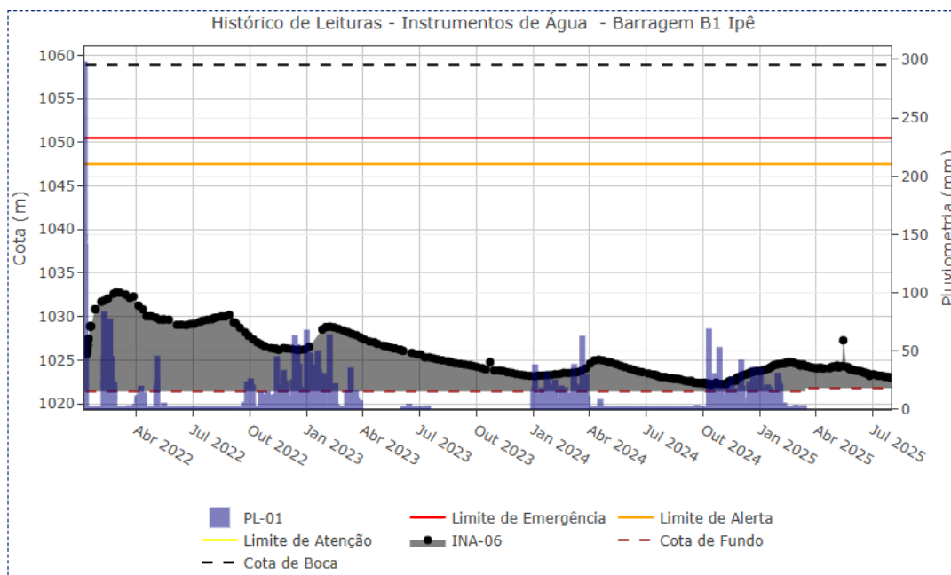
Figura 5.23 – Desempenho do indicador de nível d'água – INA-06.
