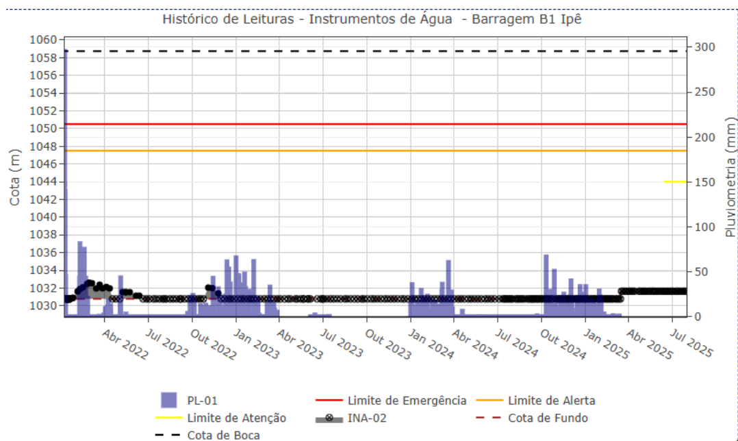
Figura 5.18 – Desempenho do indicador de nível d'água – INA-02.
