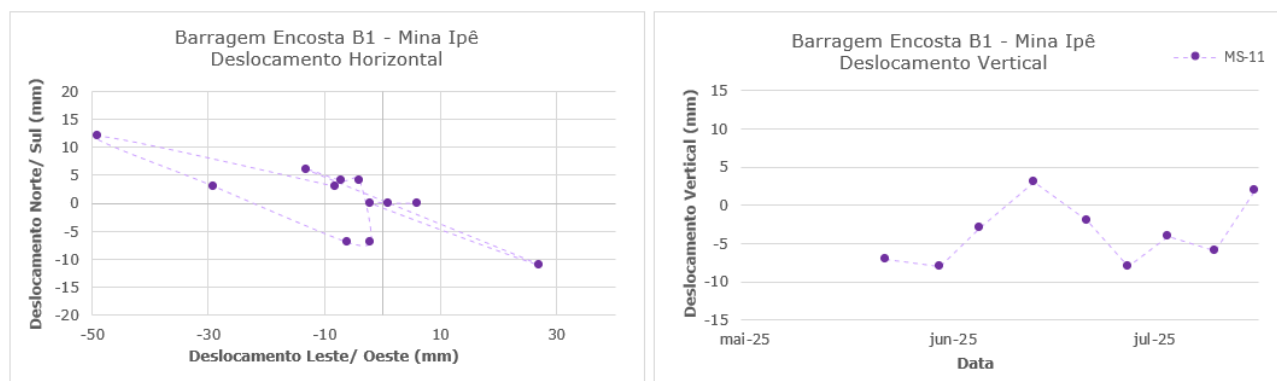
Figura 5.74 – Prisma de monitoramento da encosta MS-11.
