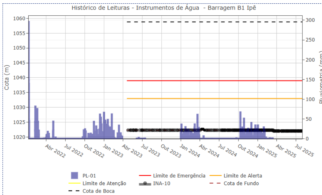
Figura 5.27 – Desempenho do indicador de nível d'água – INA-10.
