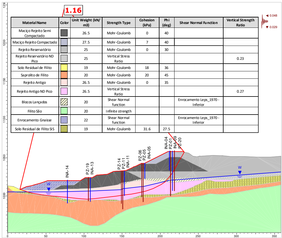
Figura 5.98 – Seção B-B' – Análise Não Drenada – Superfície de ruptura plano-circular otimizada – Freática 30/07/2025 – Razão de resistência não drenada de pico + sismo ↓ (critério vida útil).
