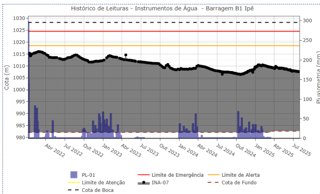
Figura 5.24 - Desempenho do indicador de nível d'água – INA-07.
