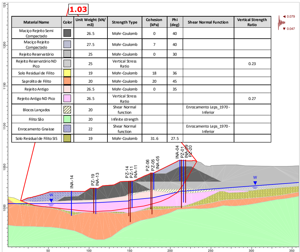
Figura 5.96 – Seção B-B’ – Análise Não Drenada – Superfície de ruptura plano-circular otimizada – Freática 30/07/2025 – Razão de resistência não drenada de pico + sismo ↓ (critério CDA).
