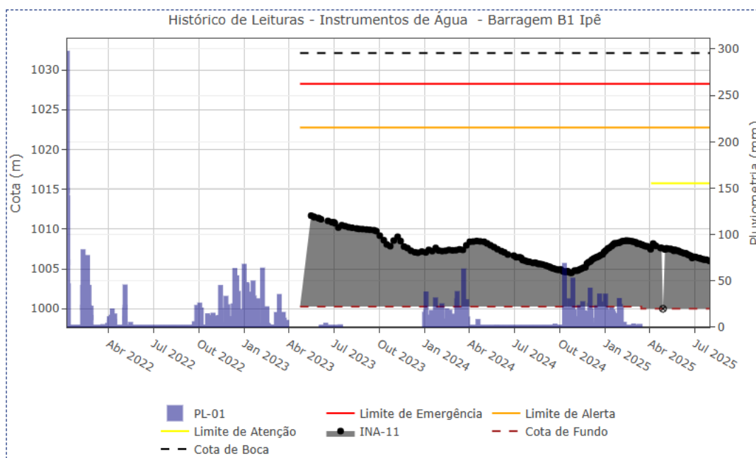
Figura 5.28 – Desempenho do indicador de nível d'água – INA-11.
