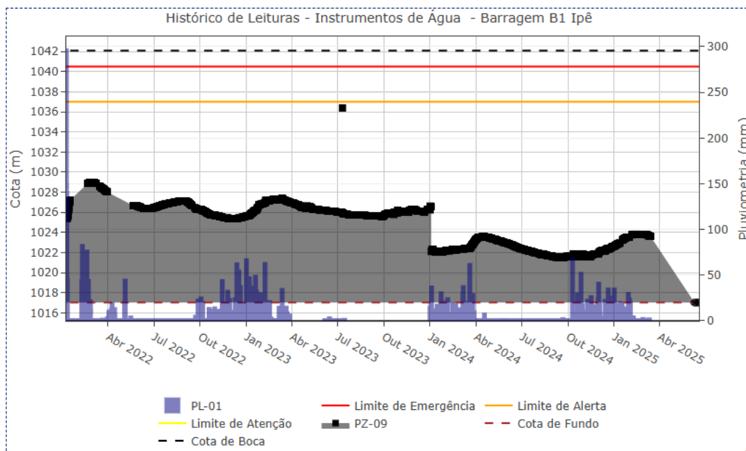
Figura 5.40 – Desempenho do piezômetro automatizado selado – PZ-09.
