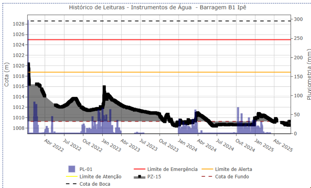
Figura 5.46 – Desempenho do piezômetro automatizado selado – PZ-15.
