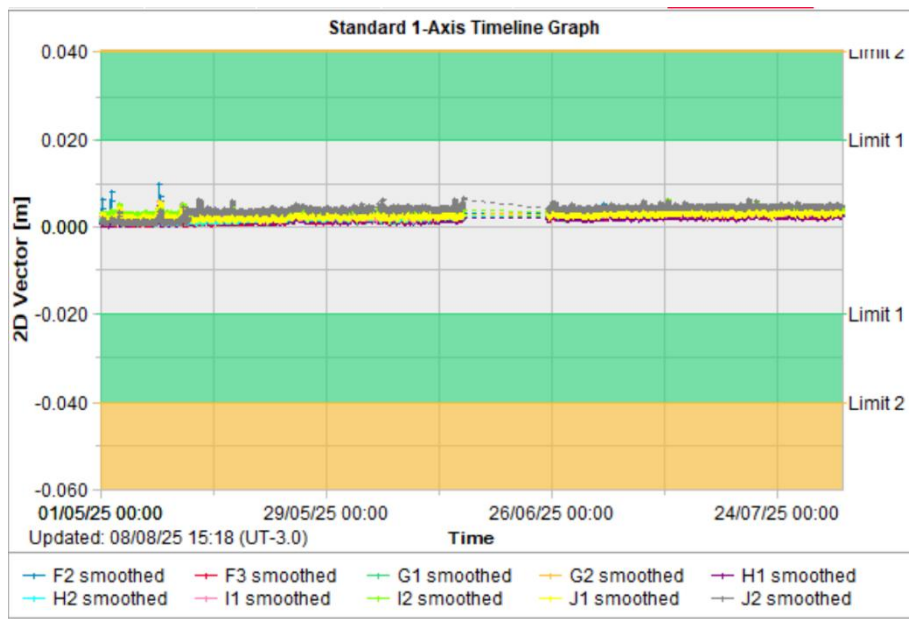
Figura 5.59 – Registros parciais das leituras dos prismas – 2D Vector. (ref: 01/05/25 a 31/07/25)
