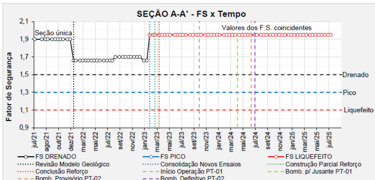
Figura 5.106 – Seção A-A' - Histórico dos F.S. obtidos nas análises de estabilidade.
