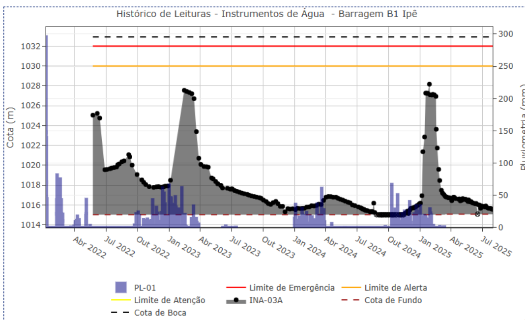
Figura 5.20 – Desempenho do indicador de nível d'água – INA-03A.
