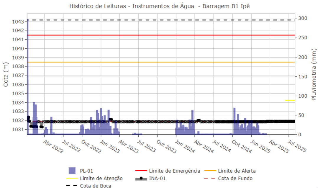
Figura 5.17 – Desempenho do indicador de nível d'água – INA-01.
