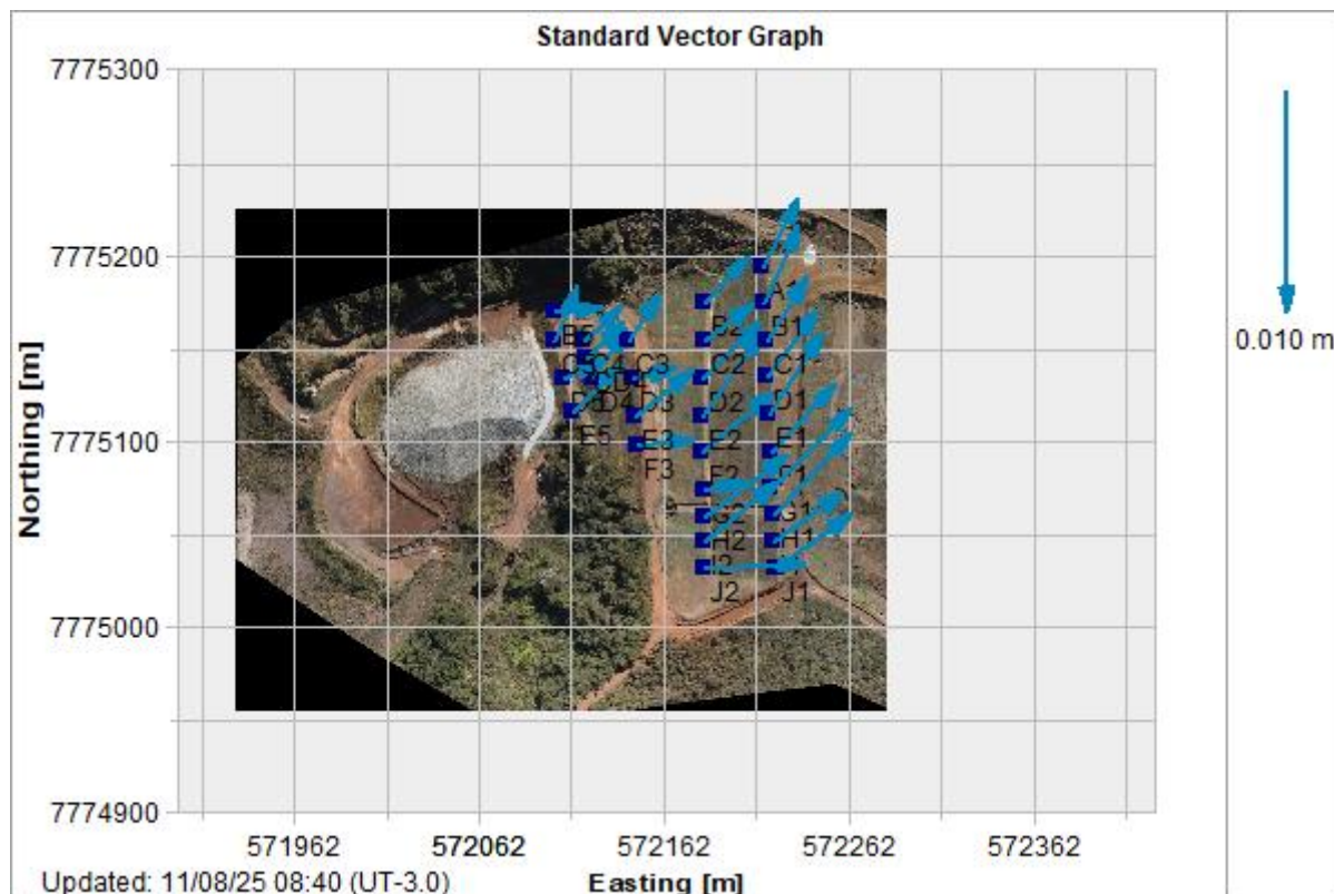
Figura 5.55 – Registros vetores deslocamento dos prismas. (ref: 01/05/25 a 31/07/25)
