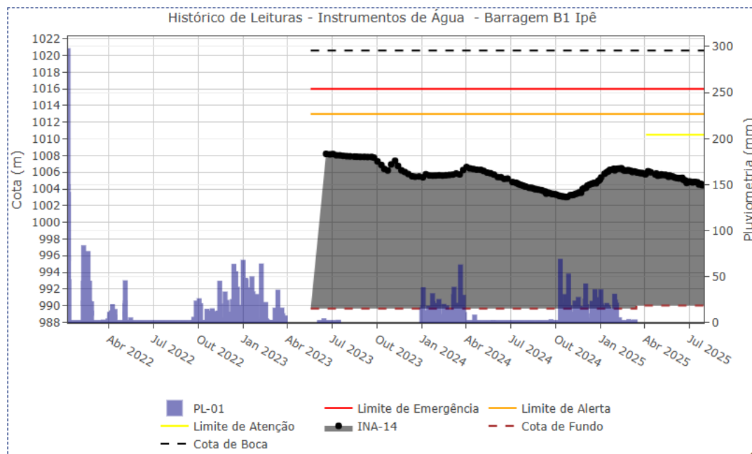
Figura 5.31 – Desempenho do indicador de nível d'água – INA-14.
