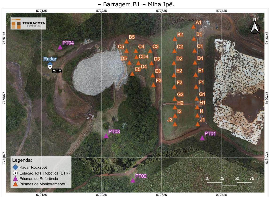
Figura 5.13 – Localização dos prismas instalados no maciço da Barragem B1 – Mina Ipê.
