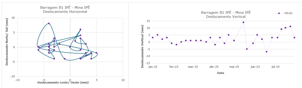
Figura 5.62 – Marco de controle de deformação – MS-03.
