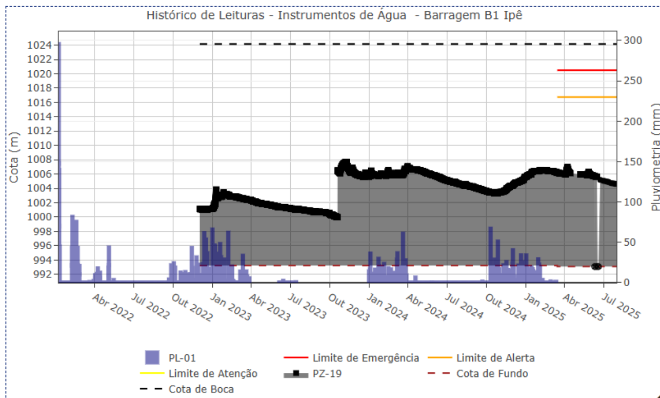
Figura 5.50 – Desempenho do piezômetro automatizado – PZ-19.
