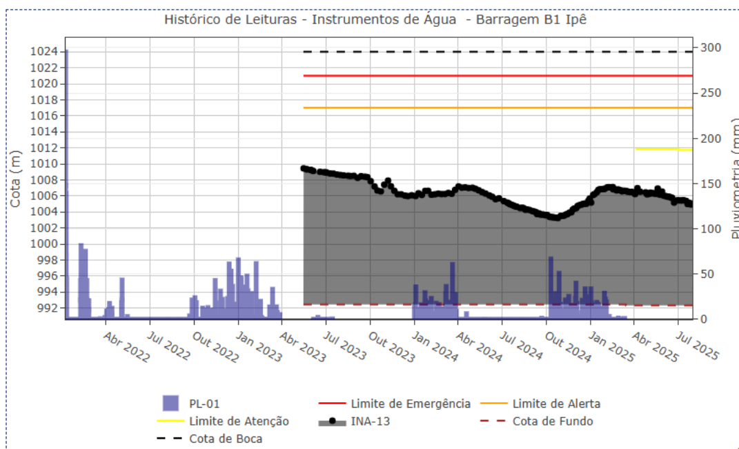
Figura 5.30 – Desempenho do indicador de nível d'água – INA-13.
