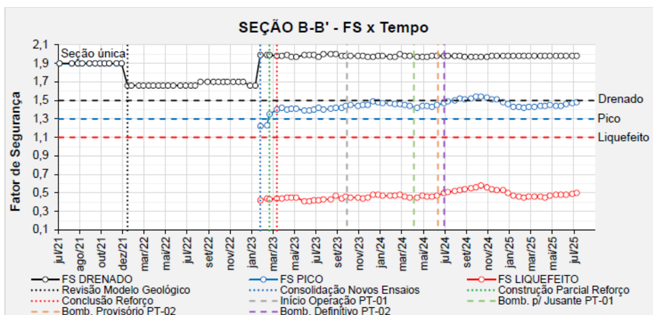
Figura 5.107 – Seção B-B' - Histórico dos F.S. obtidos nas análises de estabilidade.
