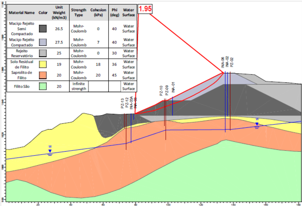
Figura 5.85 – Seção A-A’ – Análise Drenada – Superfície de ruptura plano-circular otimizada – Freática 30/07/2025.
