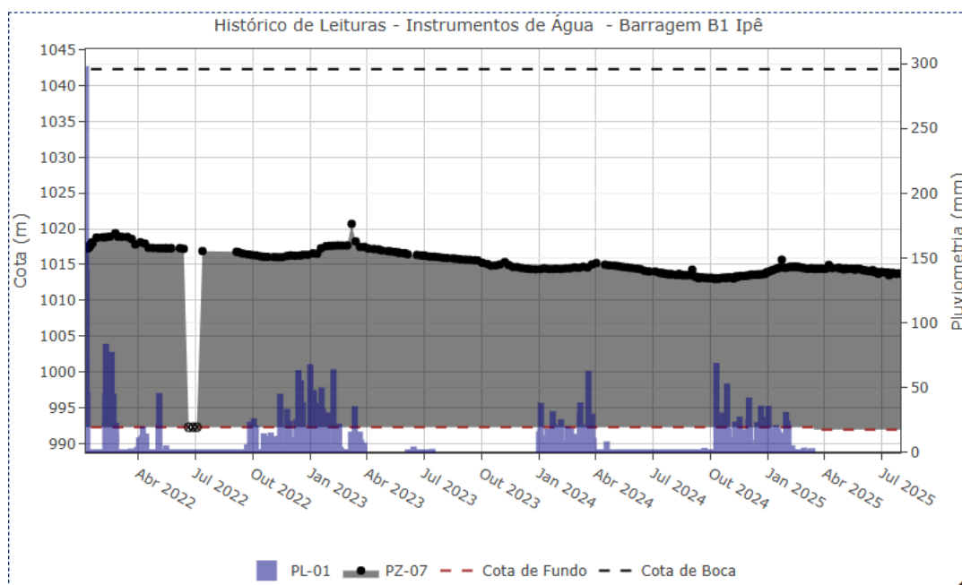
Figura 5.38 – Desempenho do piezômetro de tubo aberto – PZ-07.
