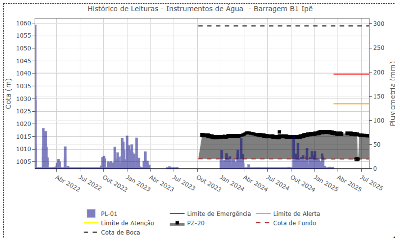
Figura 5.51 – Desempenho do piezômetro automatizado – PZ-20.
