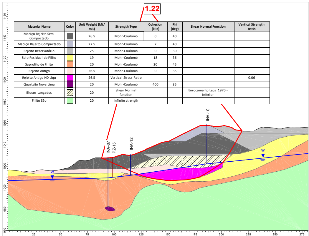
Figura 5.101 – Seção C-C’ – Análise Não Drenada – Superfície de ruptura plano-circular otimizada – Freática 30/07/2025 – Razão de resistência não drenada liquefeito.
