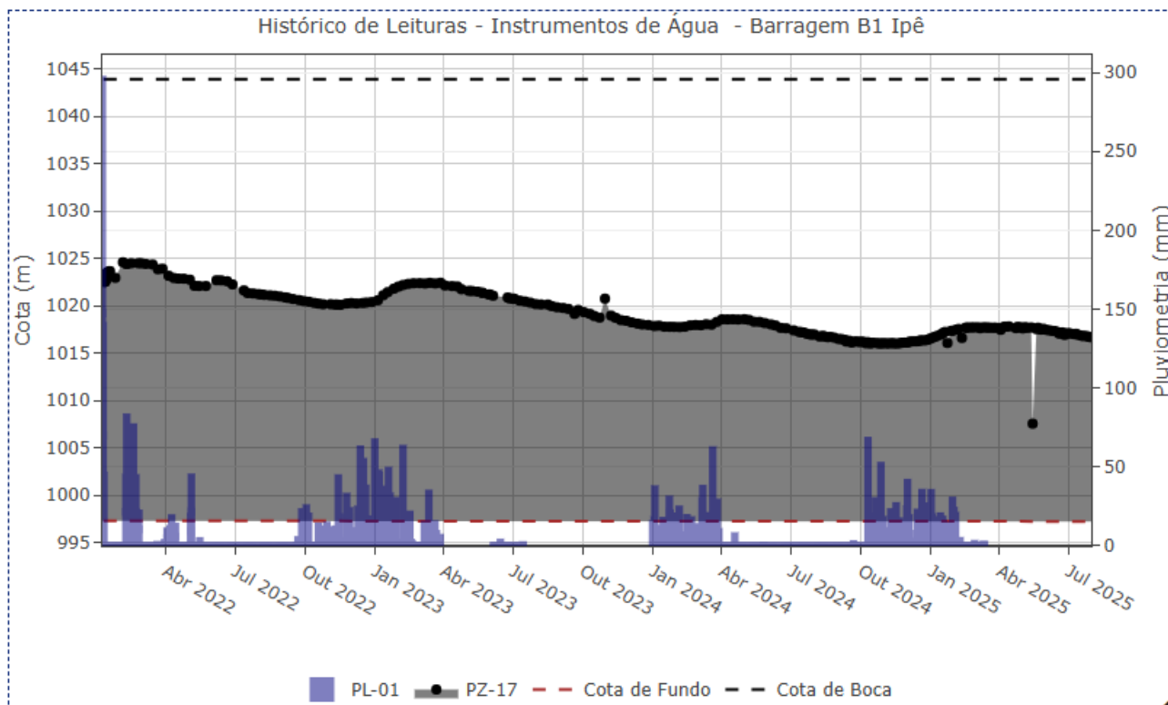
Figura 5.48 – Desempenho do piezômetro de tubo aberto – PZ-17.
