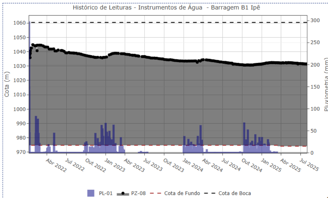
Figura 5.39 – Desempenho do piezômetro de tubo aberto – PZ-08.
