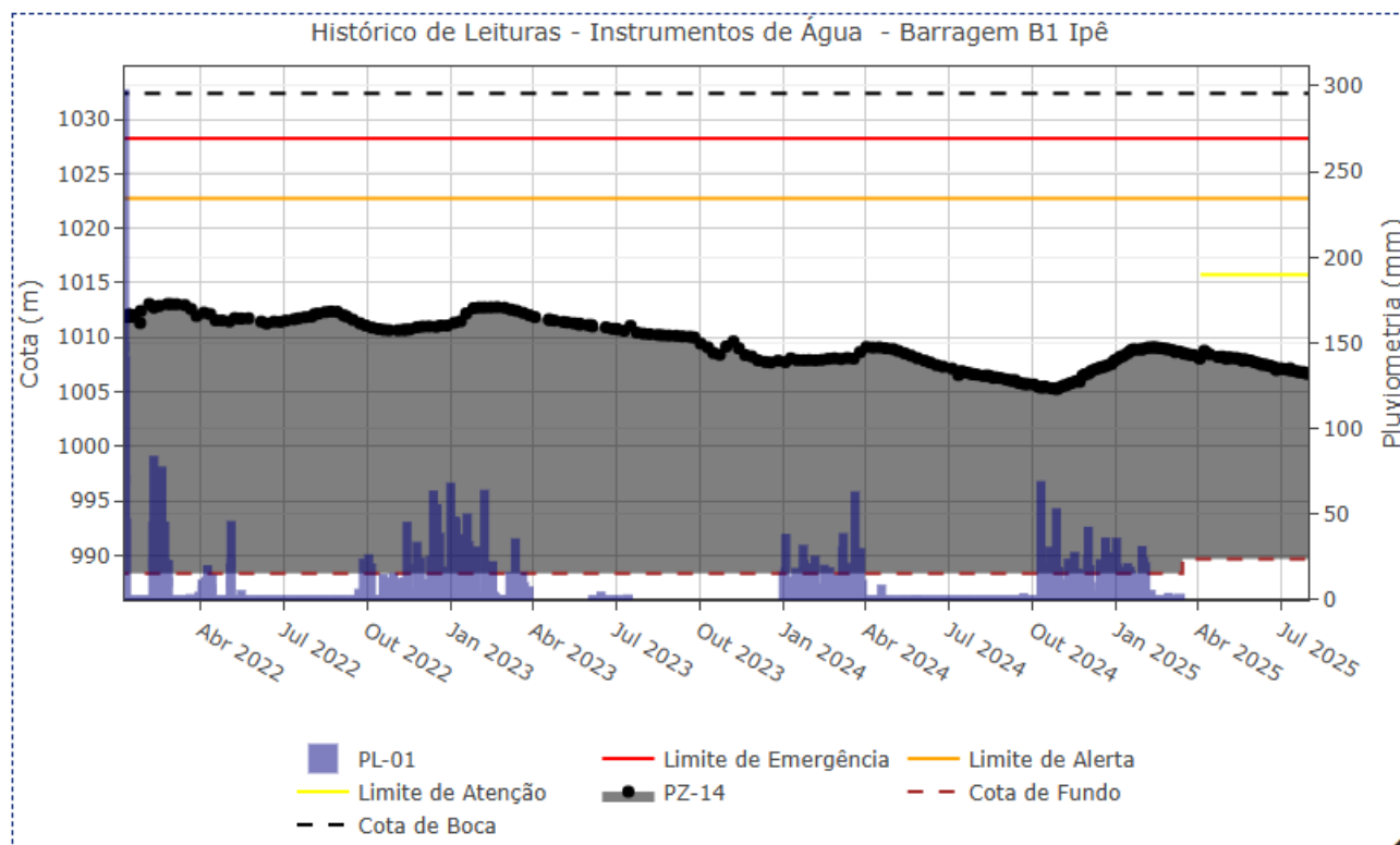
Figura 5.45 – Desempenho do piezômetro de tubo aberto – PZ-14.
