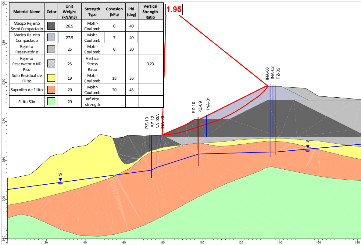
Figura 5.86 – Seção A-A’ – Análise Não Drenada – Superfície de ruptura plano-circular otimizada – Freática 30/07/2025 – Razão de resistência não drenada de pico.
