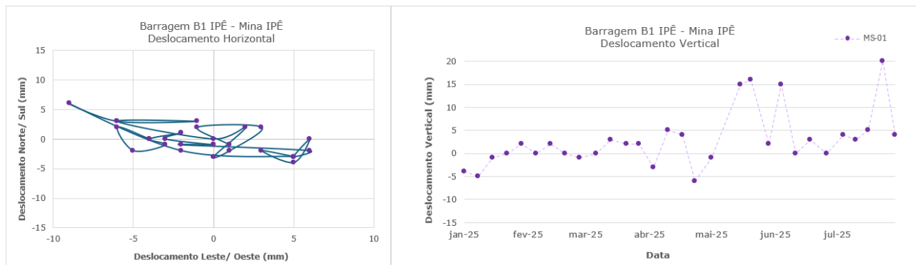
Figura 5.60 – Marco de controle de deformação – MS-01.
