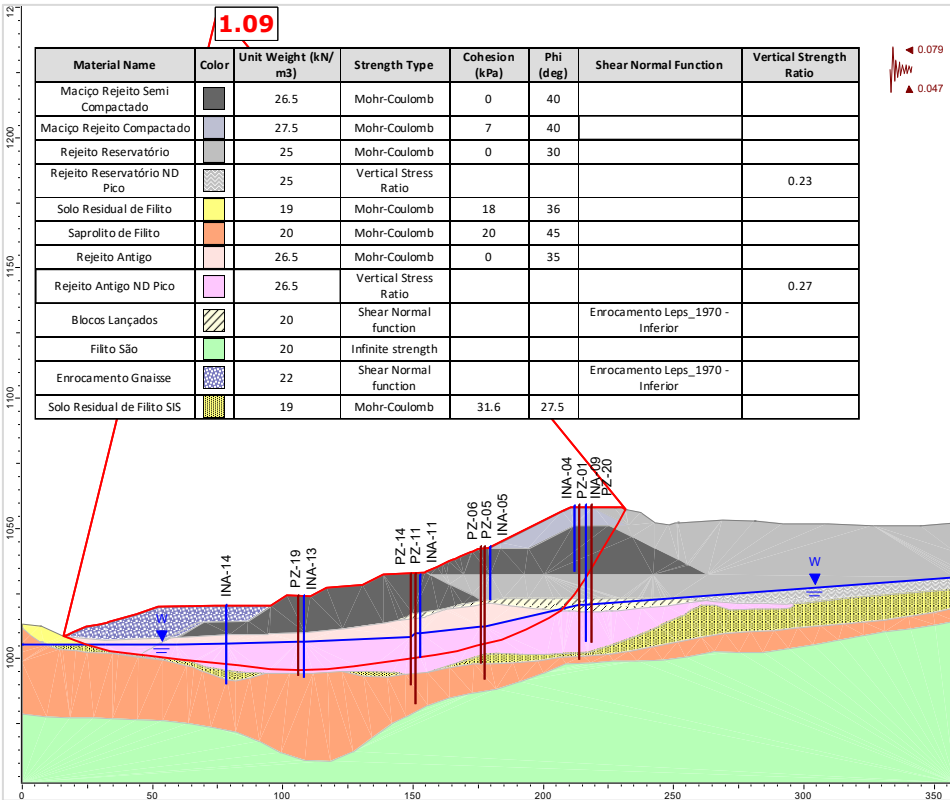
Figura 5.95 – Seção B-B’ – Análise Não Drenada – Superfície de ruptura plano-circular otimizada – Freática 30/07/2025– Razão de resistência não drenada de pico + sismo ↑ (critério CDA).
