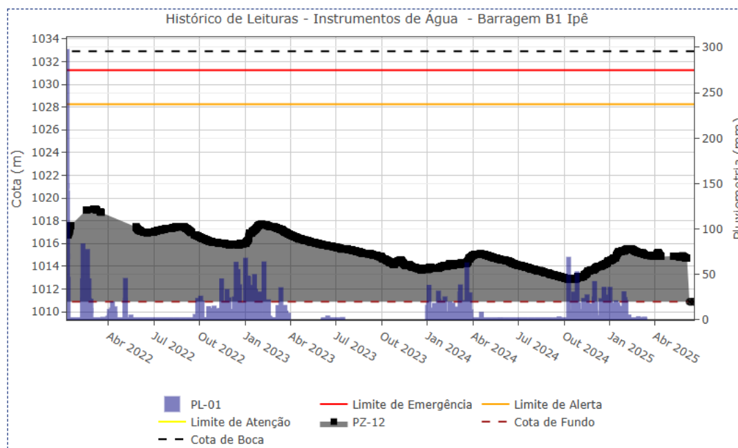
Figura 5.43 – Desempenho do piezômetro automatizado selado – PZ-12.
