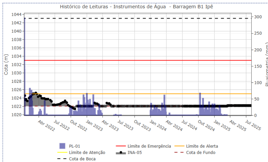
Figura 5.22 – Desempenho do indicador de nível d'água – INA-05.
