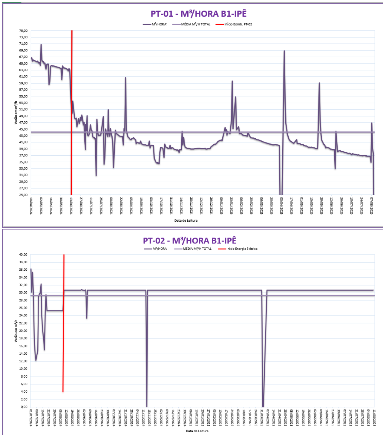
Figura 5.81 – Histórico bombeamento dos poços de rebaixamento.
