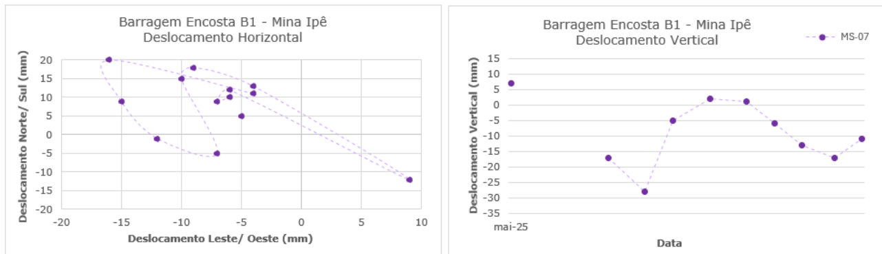
Figura 5.70 – Prisma de monitoramento da encosta MS-07.
