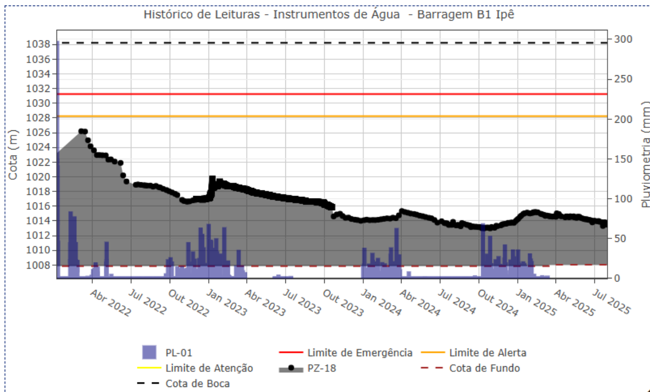
Figura 5.49 – Desempenho do piezômetro de tubo aberto – PZ-18.
