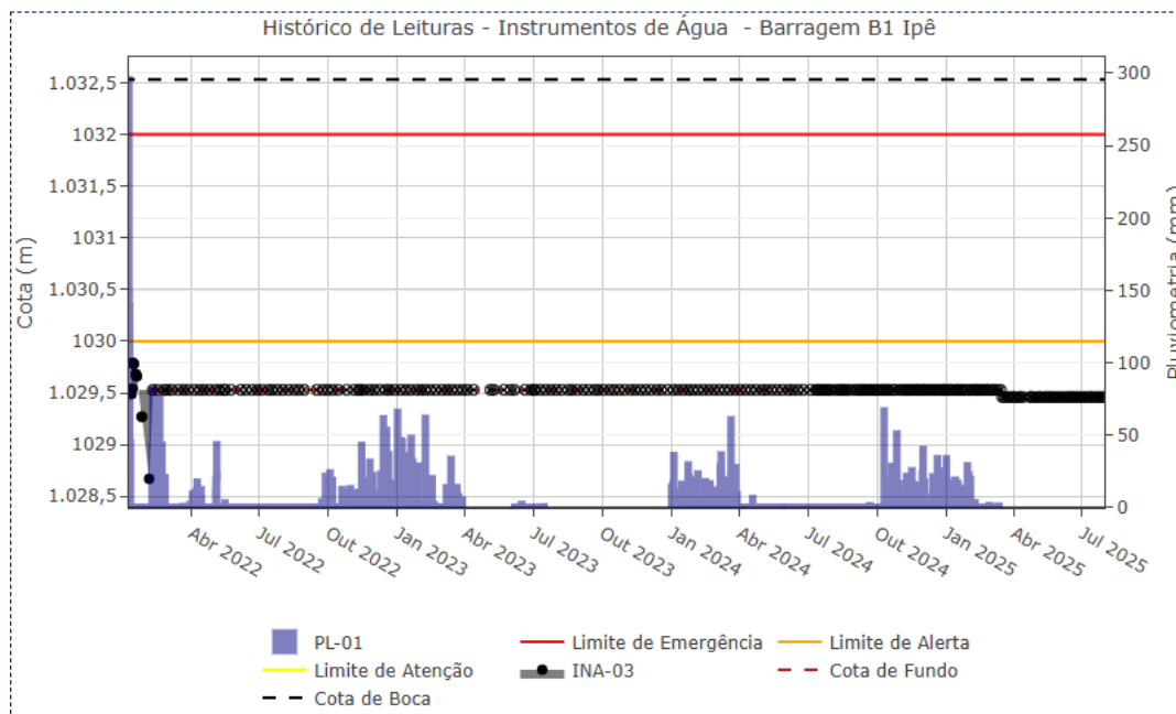
Figura 5.19 – Desempenho do indicador de nível d'água – INA-03.
