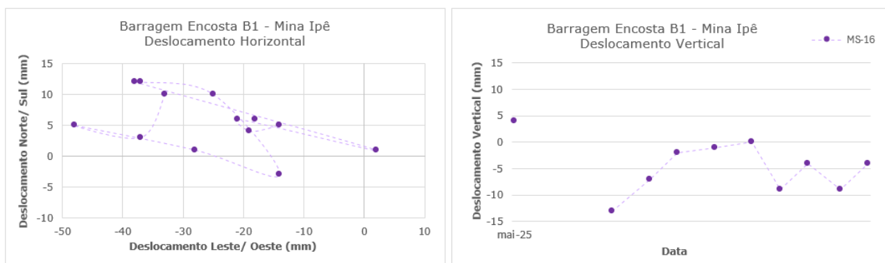
Figura 5.79 – Prisma de monitoramento da encosta MS-16.
