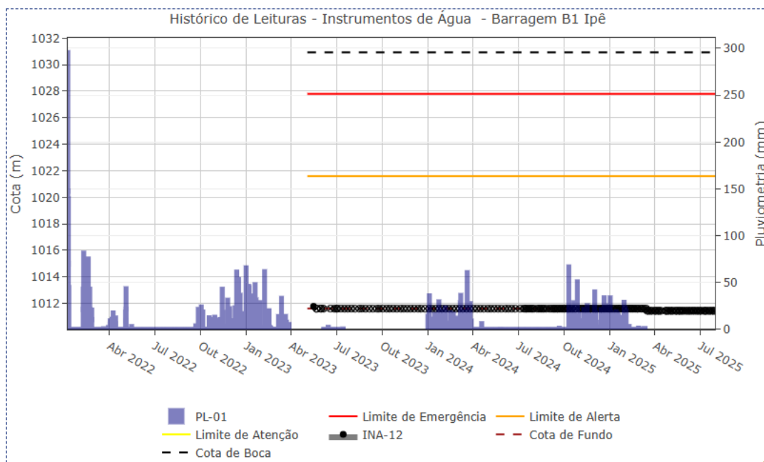
Figura 5.29 – Desempenho do indicador de nível d'água – INA-12.
