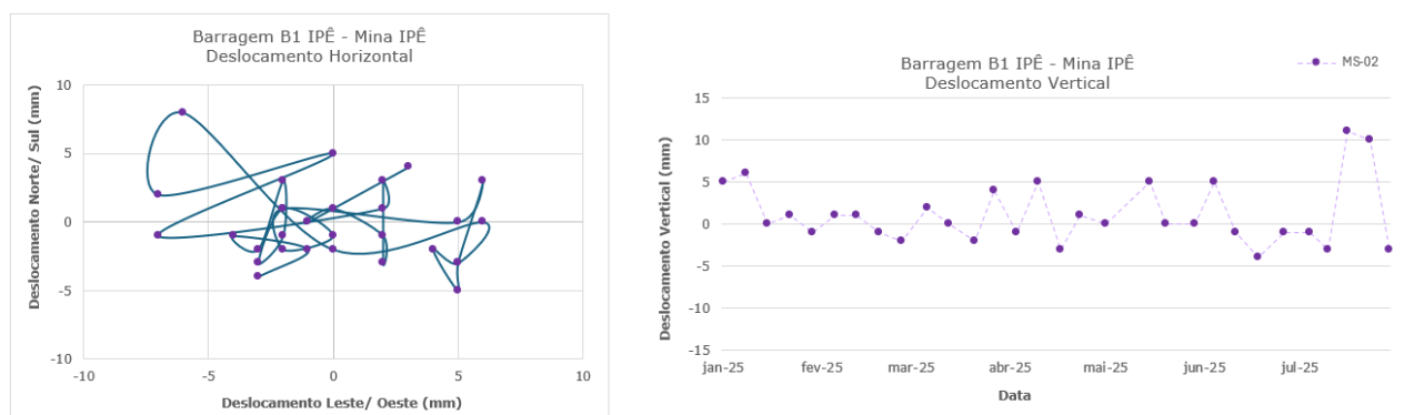
Figura 5.61 – Marco de controle de deformação – MS-02.
