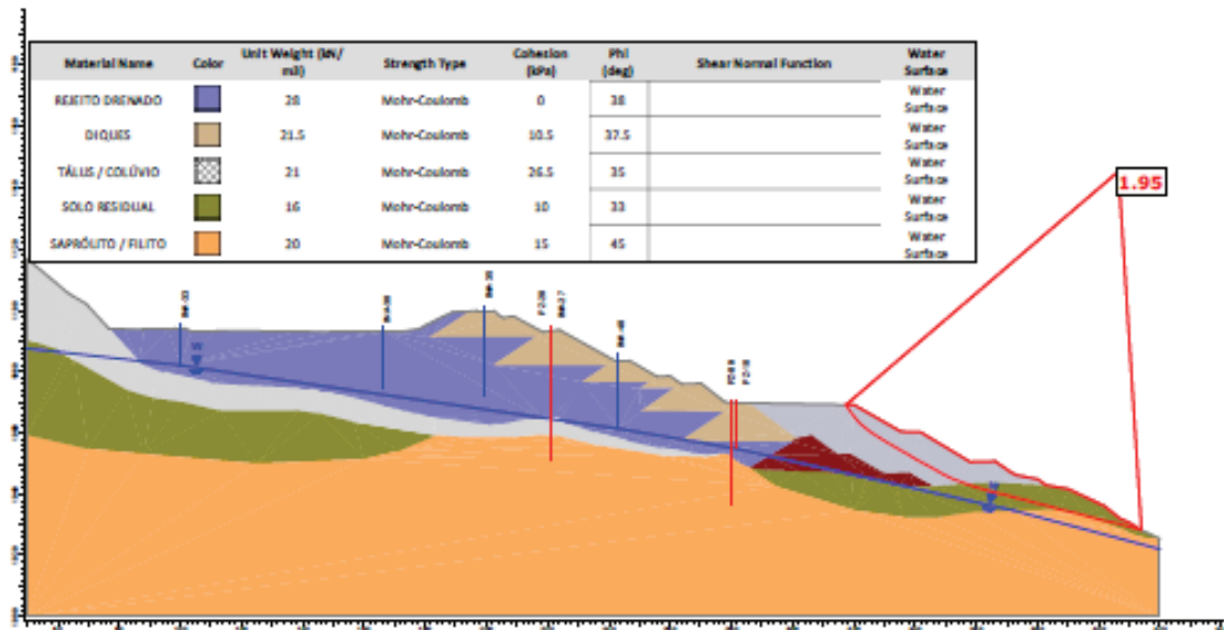
Figura 7.59 - Seção E-E' – Análise Drenada – Superfície de ruptura plano-circular otimizada – Freática atual (27/04/2026).
