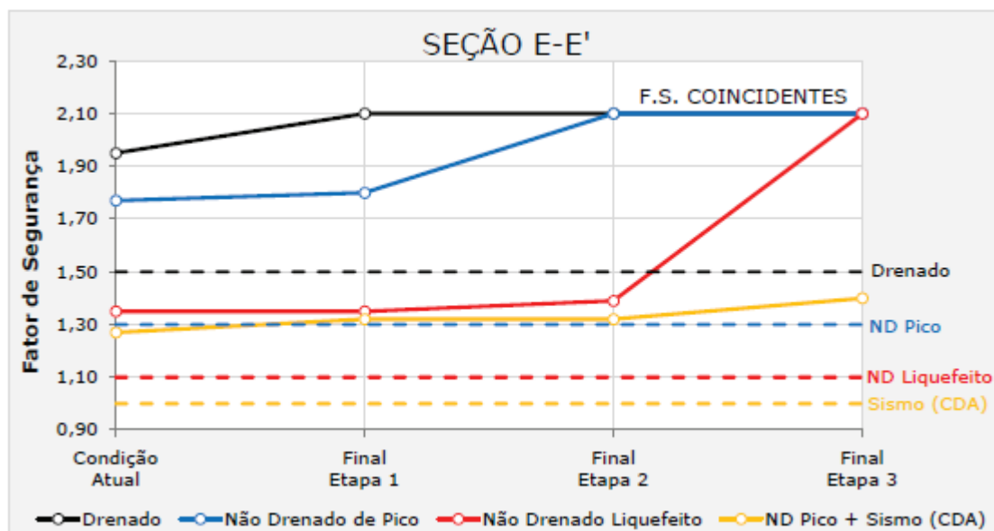
Figura 7.95 - Seção E-E' – Projeção da evolução dos fatores de segurança durante obra.
