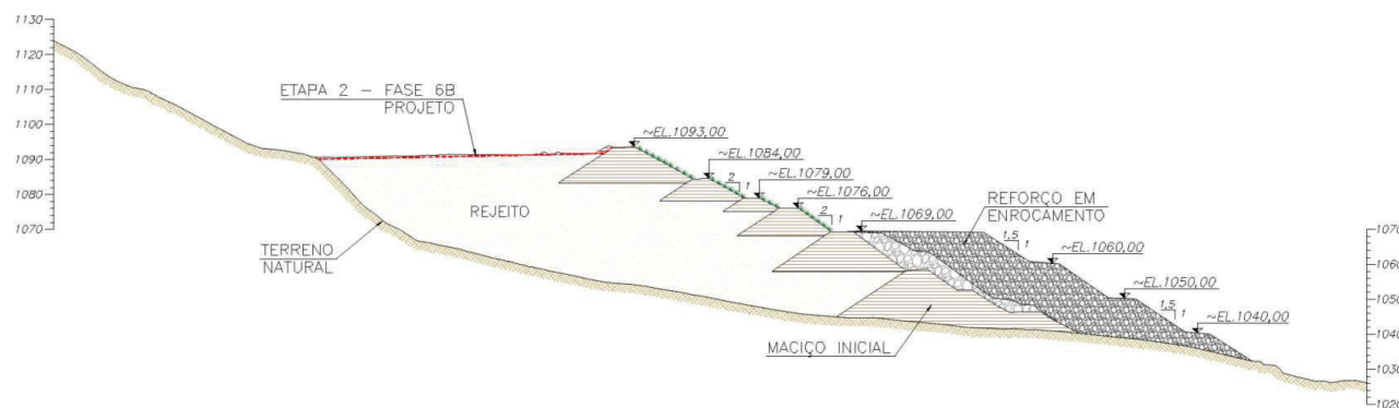
Figura 6.10 – Comparativo Projeto (Etapa 2 - Fase 6B) x Executado – Seção B-B'.
