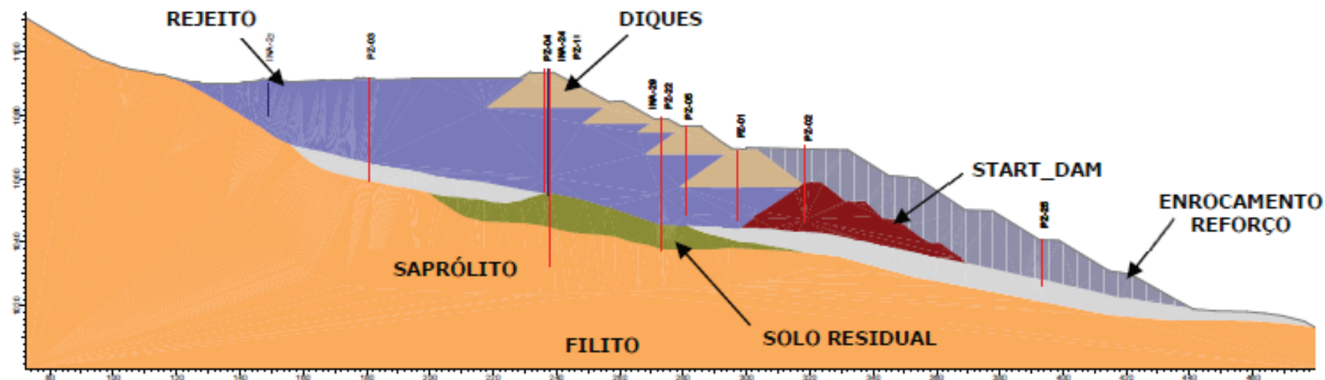
Figura 4.3 – Seção de maior altura (D-D') da Barragem B2 – Mina Tico-Tico.
