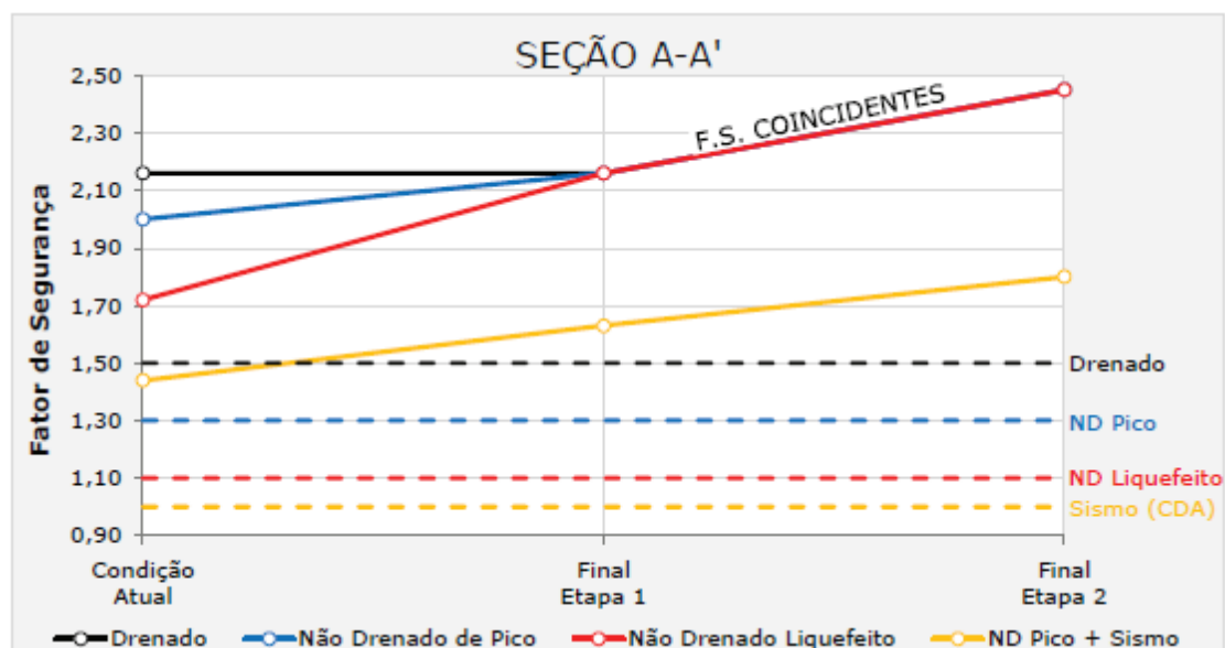
Figura 7.91 - Seção A-A' – Projeção da evolução dos fatores de segurança durante obra.
