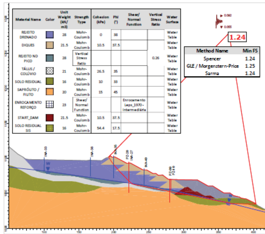
Figura 7.48 – Seção E-E’ – Análise Não Drenada – Superfície de ruptura plano-circular otimizada – Freática atual (28/02/2026) – Razão de resistência não drenada de pico + sismo ↓. – RISR – Março/2026.
