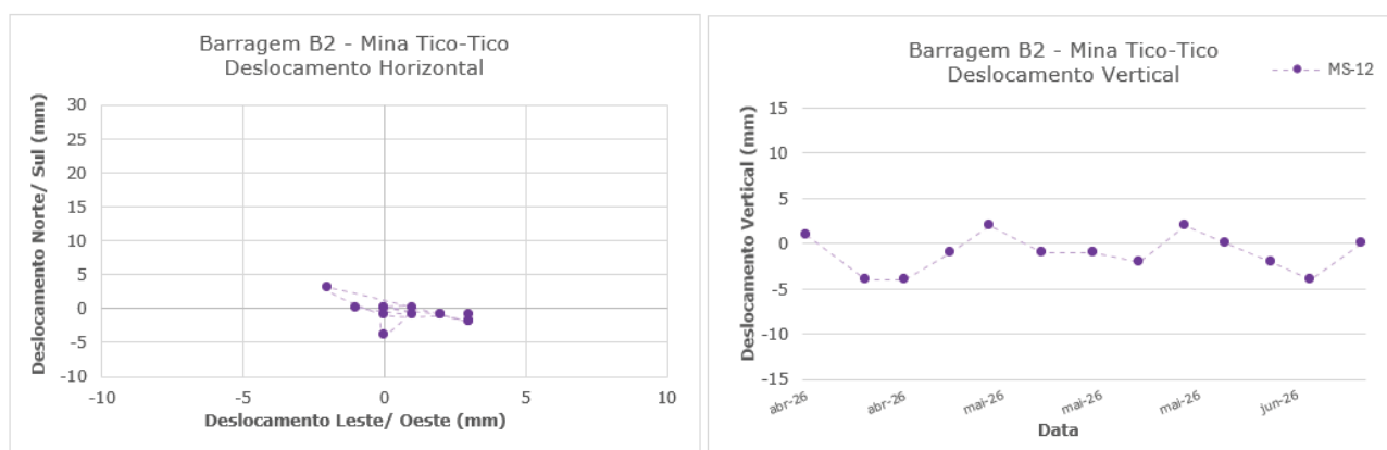
Figura 7.15 – Marco de controle de deformação – MS-12.
