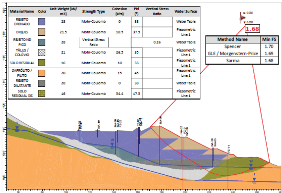
Figura 7.30 – Seção A-A’ – Análise Não Drenada – Superfície de ruptura plano-circular otimizada – Freática atual (28/02/2026) – Razão de resistência não drenada de pico + sismo ↓. – RISR – Março/2026.
