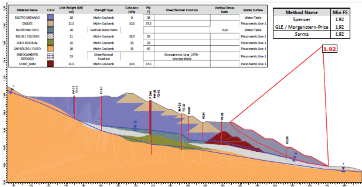
Figura 7.40 – Seção D-D’ – Análise Não Drenada – Superfície de ruptura plano-circular otimizada - Freática atual (28/02/2026) – Razão de resistência não drenada de pico. – RISR – Março/2026.
