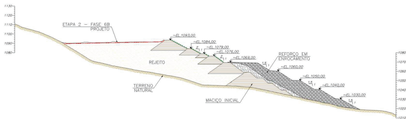
Figura 6.12 – Comparativo Projeto (Etapa 2 - Fase 6A) x Executado – Seção D-D’.
