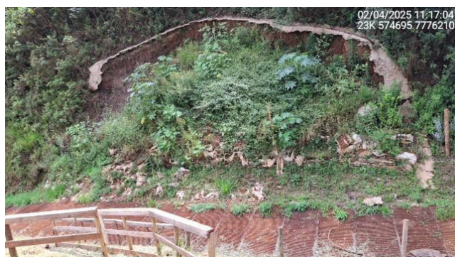
Foto 5.7 – Grades metálicas instaladas sobre o canal extravasor de emergência.
