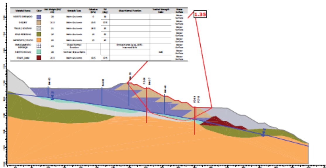
Figura 7.61 - Seção E-E' – Análise Não Drenada – Superfície de ruptura plano-circular otimizada - Freática atual (27/04/2026) – Razão de resistência não drenada liquefeita.
