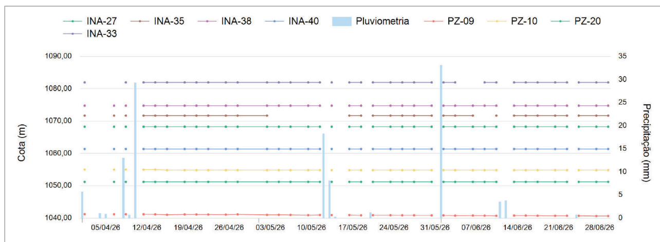
Figura 7.8 – Instrumentos Seção E-E.
