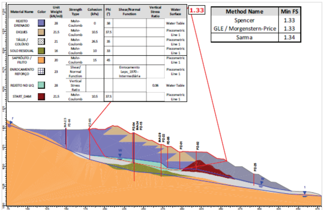
Figura 7.41 – Seção D-D’ – Análise Não Drenada – Superfície de ruptura plano-circular – Freática atual (28/02/2026) – Razão de resistência não drenada liquefeita. – RISR – Março/2026.
