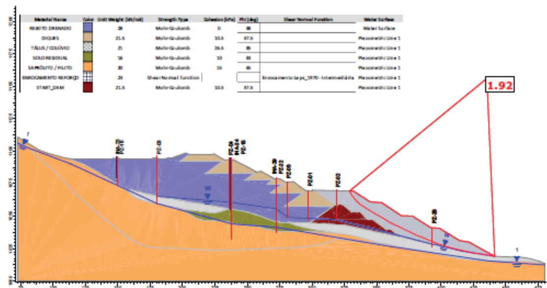
Figura 7.56 - Seção D-D' – Análise Drenada – Superfície de ruptura plano-circular otimizada – Freática atual (27/04/2026).
