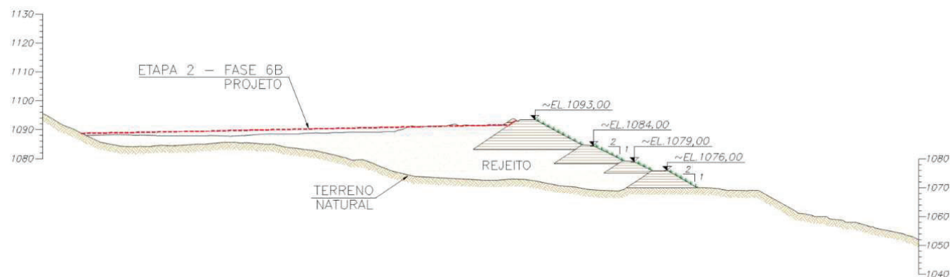
Figura 6.11 – Comparativo Projeto (Etapa 2 - Fase 6A) x Executado – Seção C-C’.
