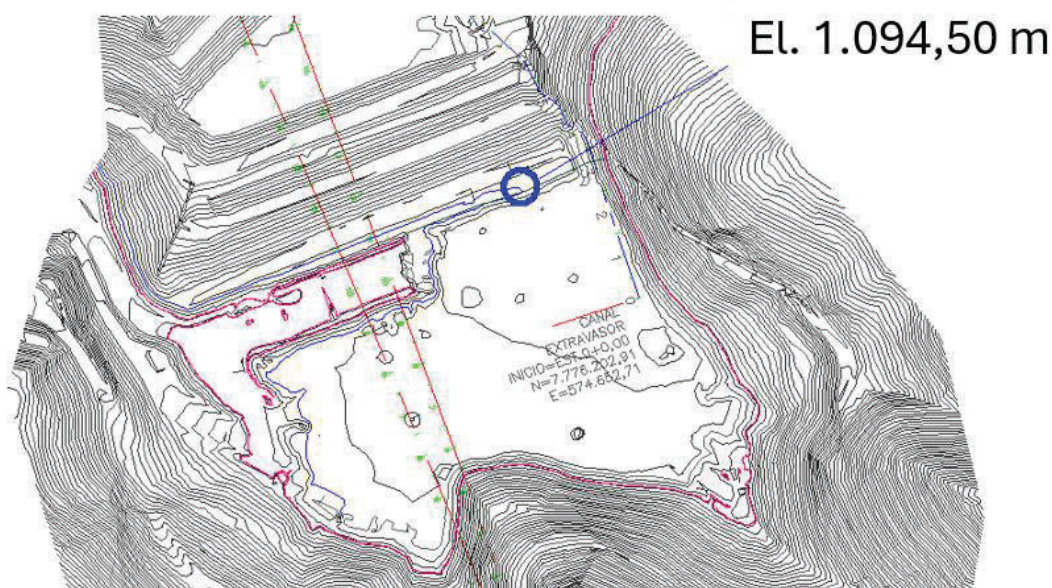
Figura 7.19 - Levantamento utilizado para definição da Curva Cota x Volume da Barragem B2.
