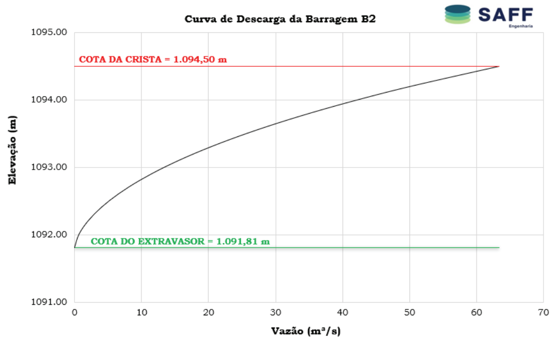
Figura 7.21 - Curva Cota x Descarga da Barragem B2 - Mina Tico-Tico.
