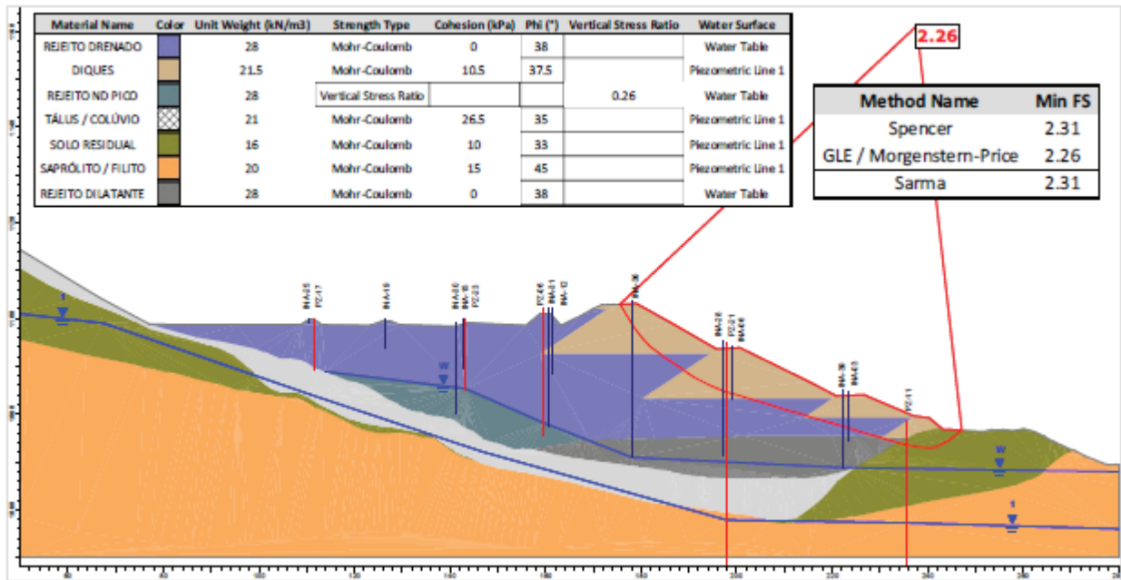
Figura 7.27 – Seção A-A’ – Análise Não Drenada – Superfície de ruptura plano-circular otimizada - Freática atual (28/02/2026) – Razão de resistência não drenada de pico. – RISR – Março/2026.
