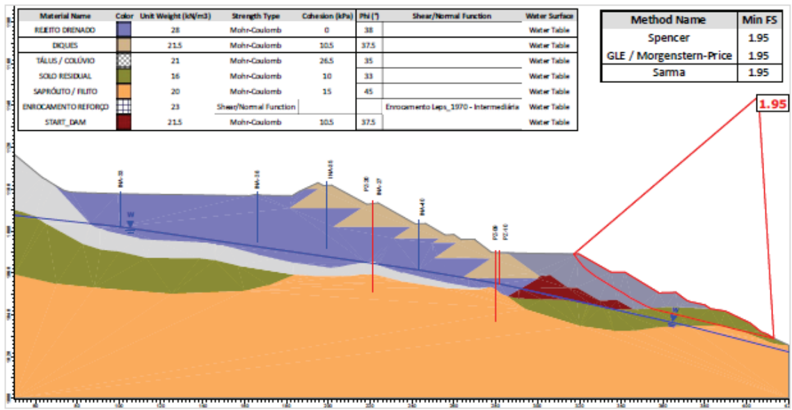
Figura 7.44 – Seção E-E’ – Análise Drenada – Superfície de ruptura plano-circular otimizada – Freática atual (28/02/2026). – RISR – Março/2026.
