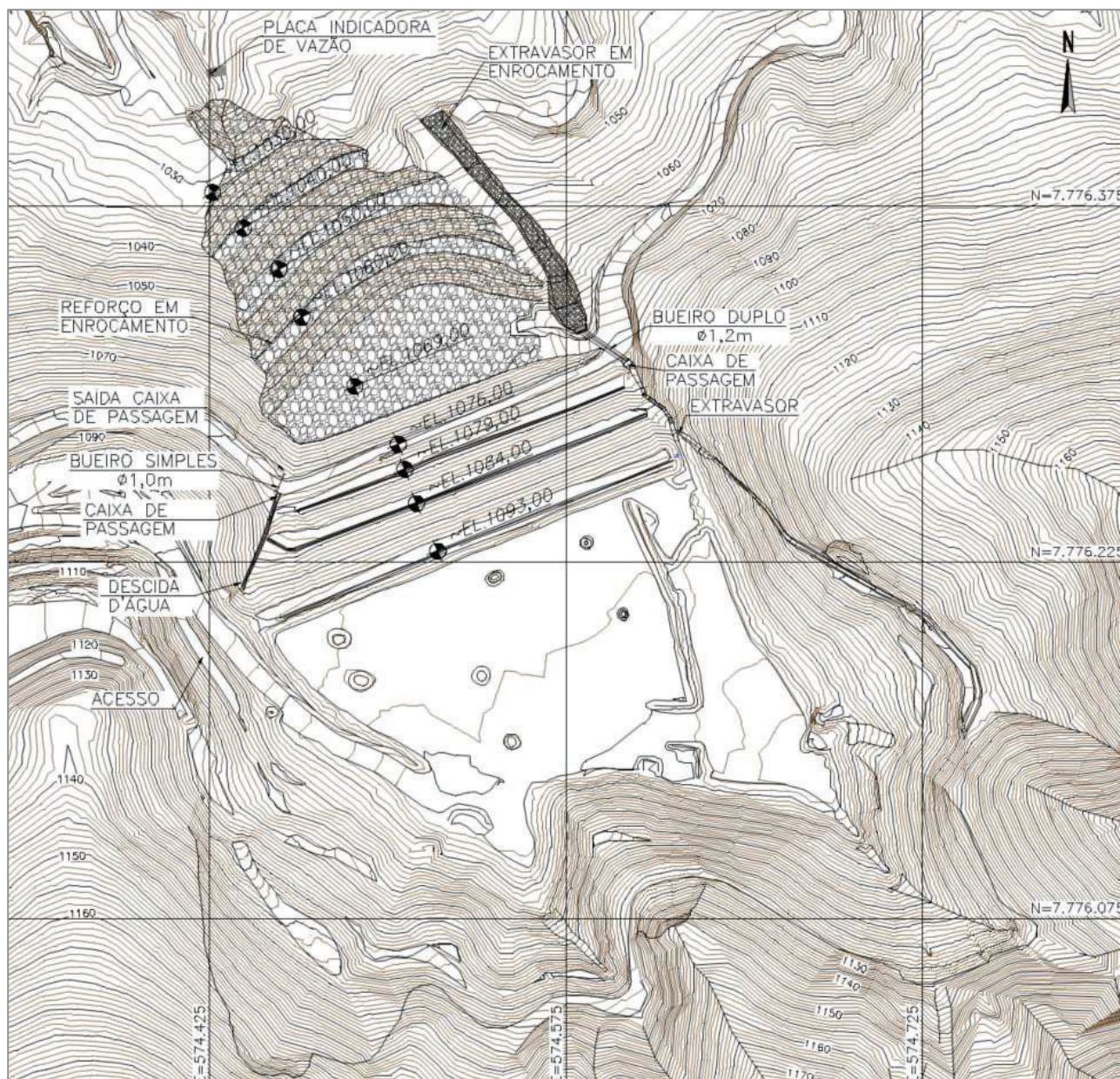
Figura 6.6 – Levantamento topográfico 01/07/2026 – Obras Executadas - Planta.
