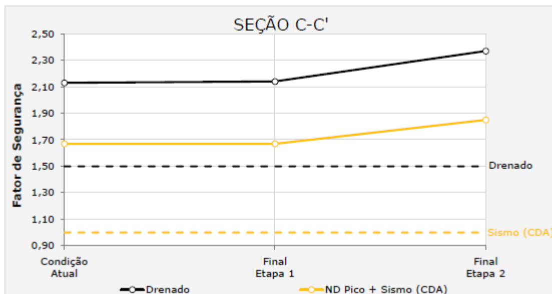
Figura 7.93 - Seção C-C' – Projeção da evolução dos fatores de segurança durante obra.
