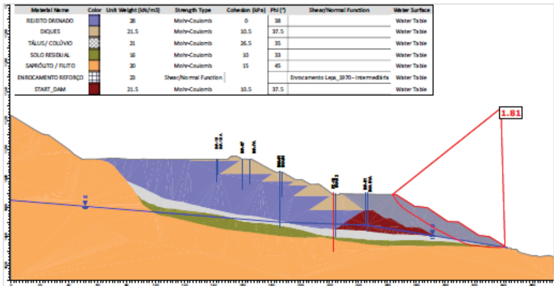
Figura 7.65 - Seção B-B' – Análise Drenada – Superfície de ruptura plano-circular otimizada – Freática atual (30/05/2026).
