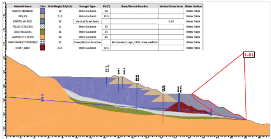
Figura 7.66 - Seção B-B' – Análise Não Drenada – Superfície de ruptura plano-circular otimizada - Freática atual (30/05/2026) – Razão de resistência não drenada de pico.
