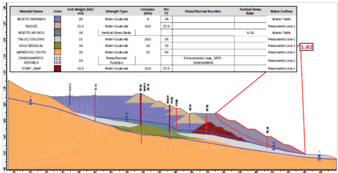
Figura 7.83 - Seção D-D' – Análise Não Drenada – Superfície de ruptura plano-circular otimizada - Freática atual (29/06/2026) – Razão de resistência não drenada de pico.
