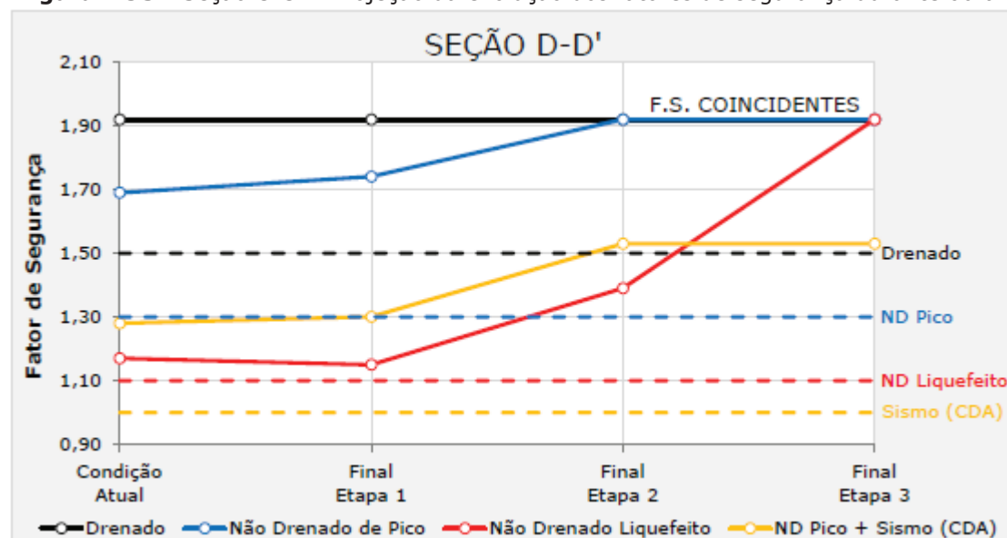
Figura 7.94 - Seção D-D' – Projeção da evolução dos fatores de segurança durante obra.
