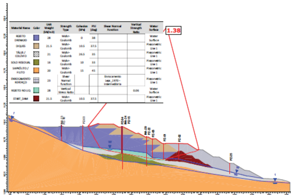
Figura 7.58 - Seção D-D' – Análise Não Drenada – Superfície de ruptura plano-circular otimizada - Freática atual (27/04/2026) – Razão de resistência não drenada liquefeita.
