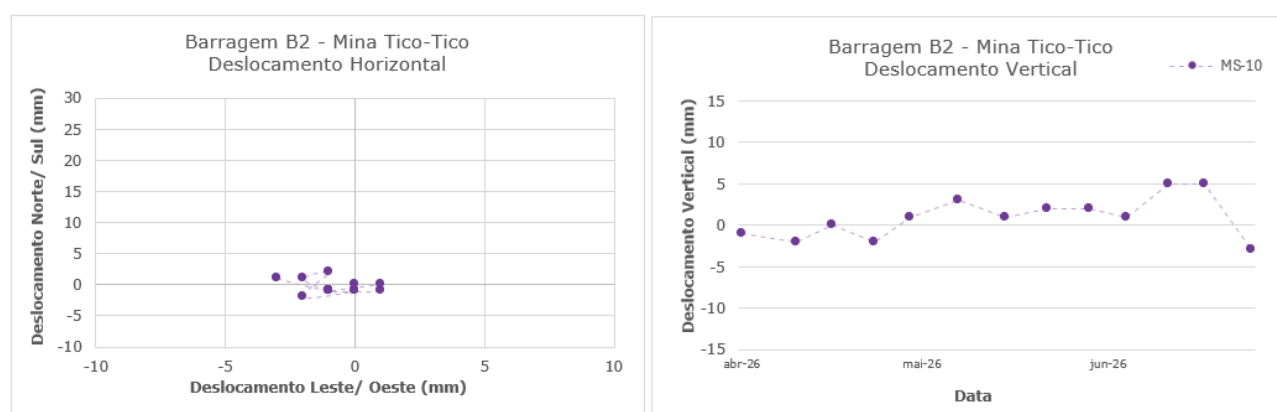
Figura 7.13 – Marco de controle de deformação – MS-10.
