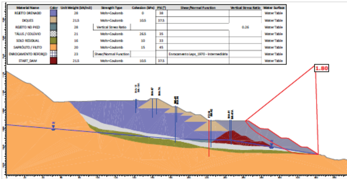
Figura 7.79 - Seção B-B' – Análise Não Drenada – Superfície de ruptura plano-circular otimizada - Freática atual (29/06/2026) – Razão de resistência não drenada de pico.
