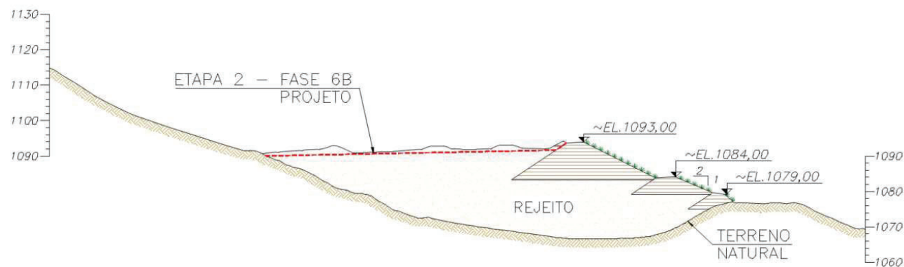
Figura 6.9 – Comparativo Projeto (Etapa 2 - Fase 6B) x Executado – Seção A-A'.
