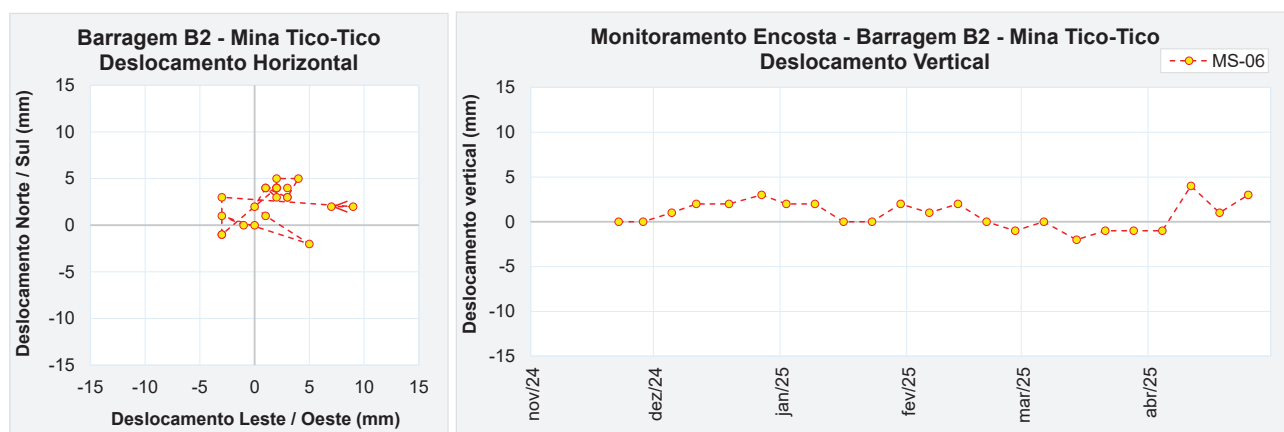
Figura 5.17 – Histórico do Marco de controle de monitoramento da encosta – MS-06.
