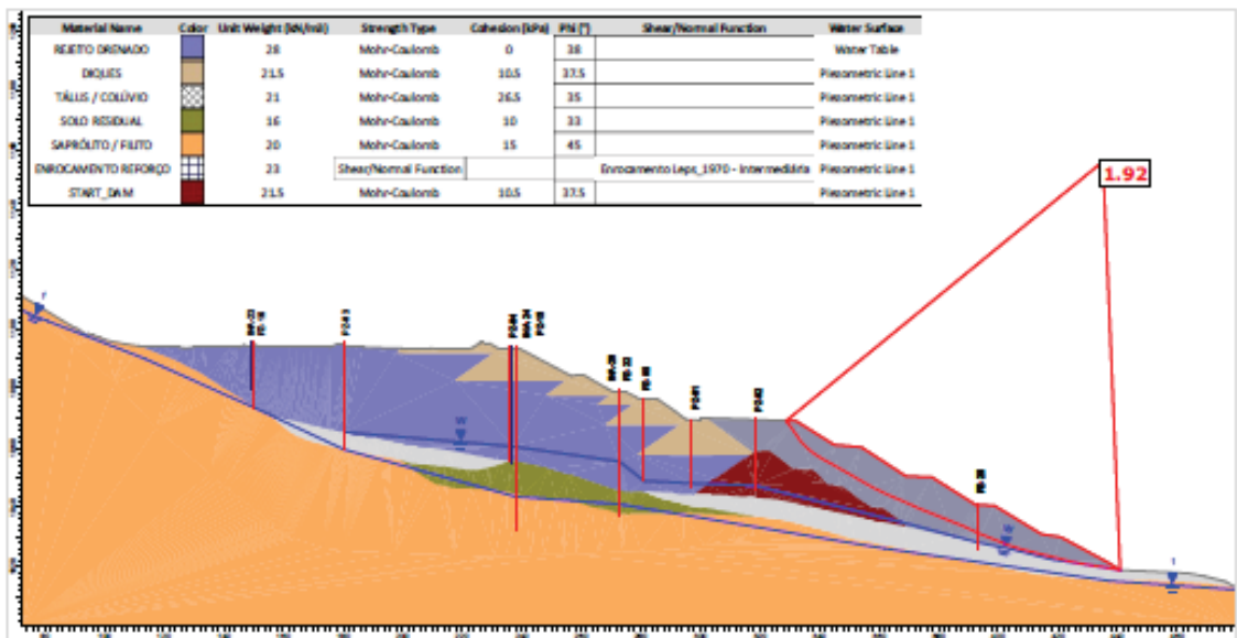
Figura 7.69 - Seção D-D' – Análise Drenada – Superfície de ruptura plano-circular otimizada – Freática atual (30/05/2026).
