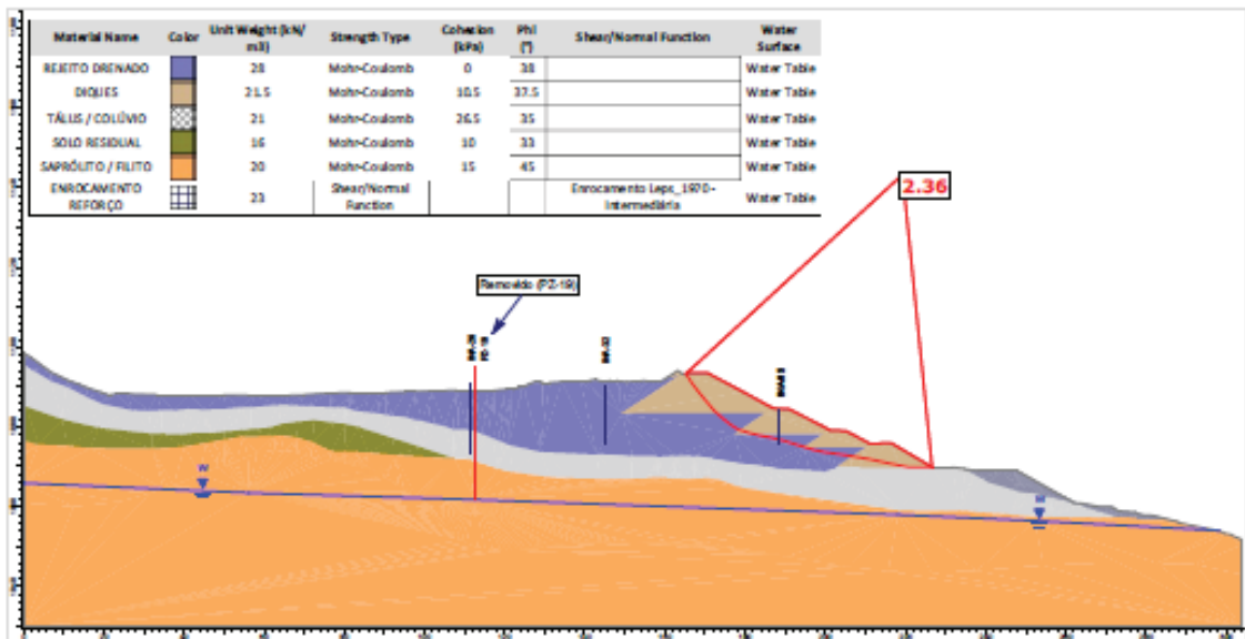
Figura 7.81 - Seção C-C' – Análise Drenada – Superfície de ruptura plano-circular otimizada – Freática atual (29/06/2026).
