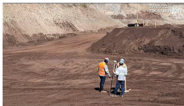
Foto 6.44 – Execução de levantamento Topográfico (Maio/26).
