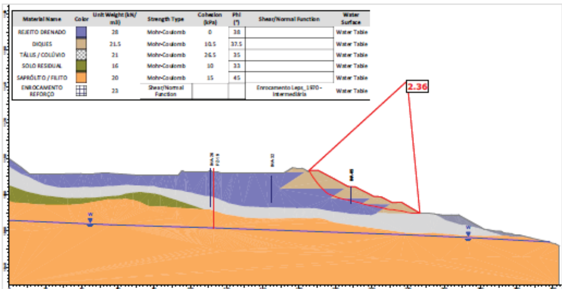
Figura 7.68 - Seção C-C' – Análise Drenada – Superfície de ruptura plano-circular otimizada – Freática atual (30/05/2026).
