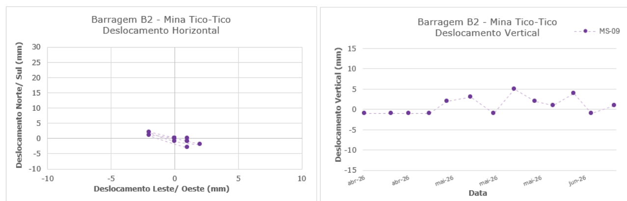
Figura 7.12 – Marco de controle de deformação – MS-09.
