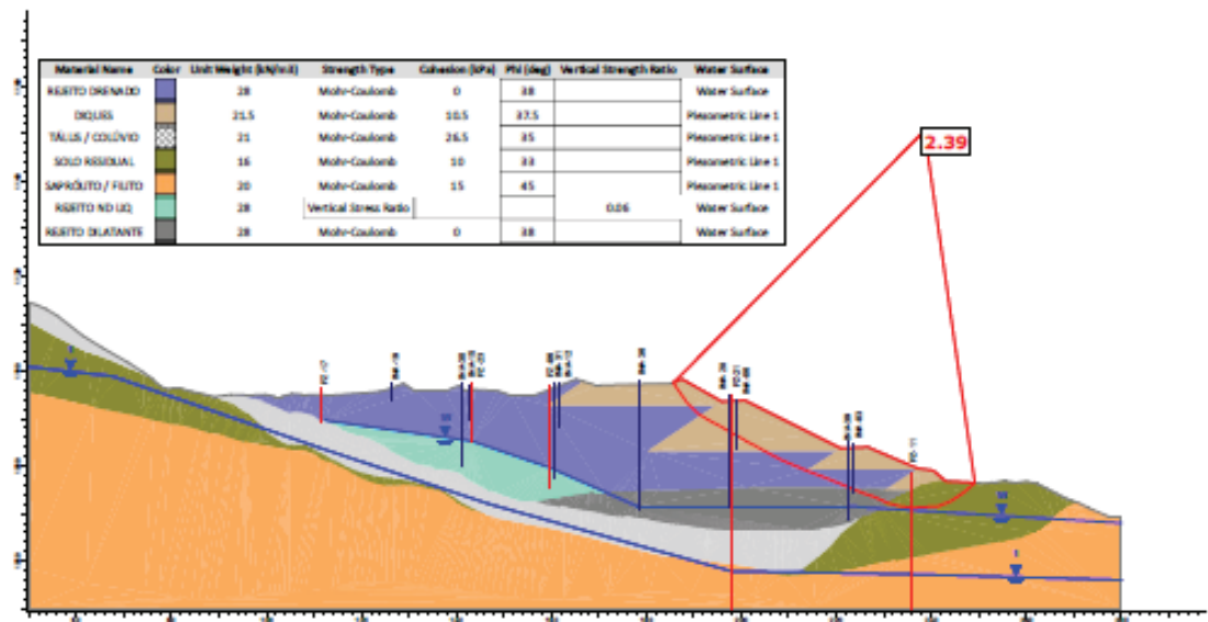
Figura 7.51 - Seção A-A' – Análise Não Drenada – Superfície de ruptura plano-circular otimizada - Freática atual (27/04/2026) – Razão de resistência não drenada liquefeita.
