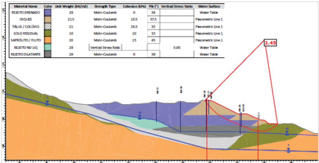
Figura 7.77 - Seção A-A' – Análise Não Drenada – Superfície de ruptura plano-circular otimizada - Freática atual (29/06/2026) – Razão de resistência não drenada liquefeita.
