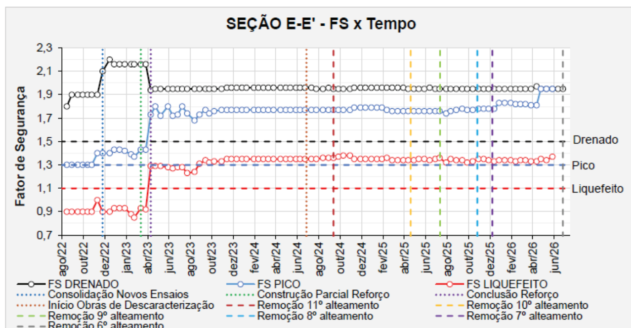
Figura 7.90 – Seção E-E' - Histórico dos F.S. obtidos nas análises de estabilidade.
