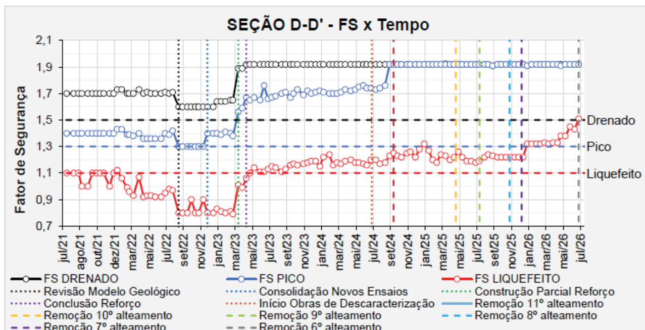
Figura 7.89 – Seção D-D' - Histórico dos F.S. obtidos nas análises de estabilidade.
