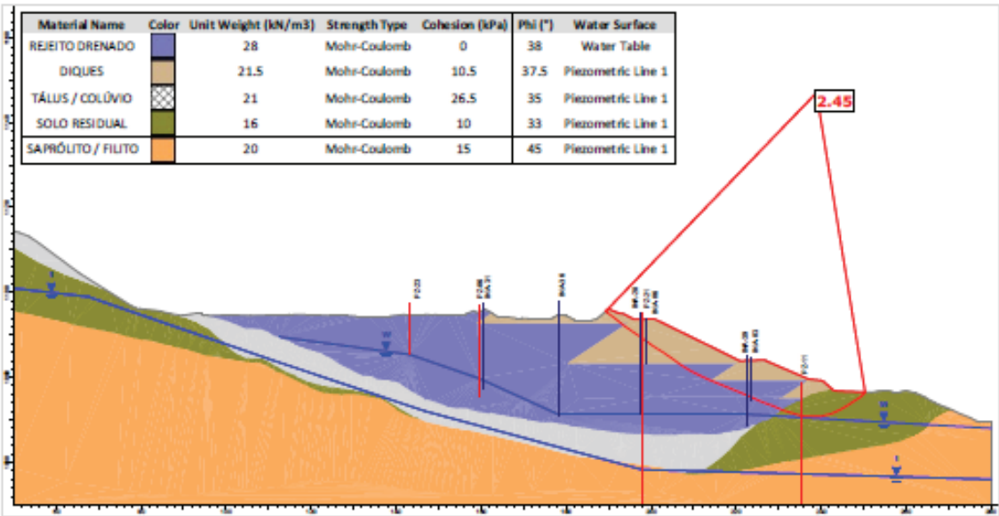
Figura 7.62 - Seção A-A' – Análise Drenada – Superfície de ruptura plano-circular otimizada – Freática atual (30/05/2026).
