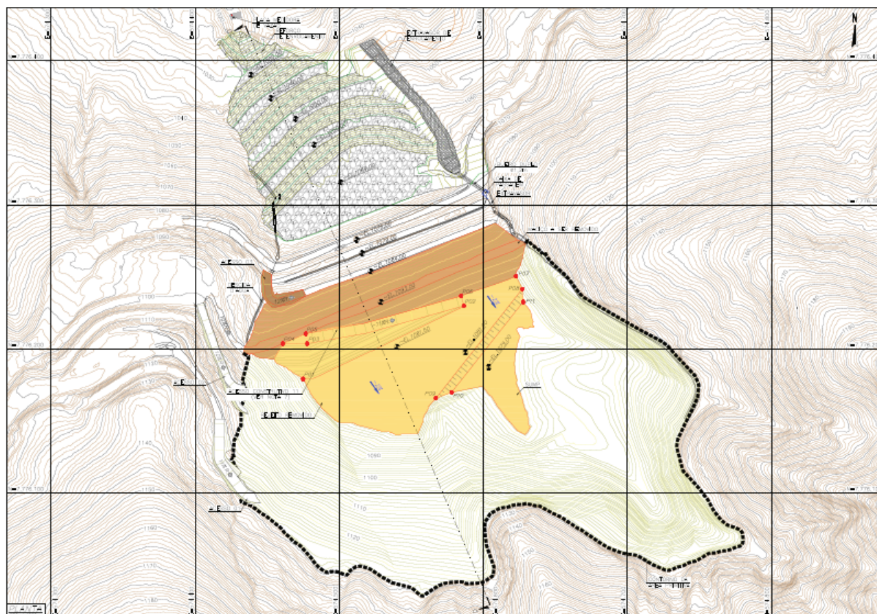
Figura 6.3 - Sequência Construtiva – Planta – Etapa 3 - Fase 7A (IPE.OP.DE.8000.GT.20.729).
