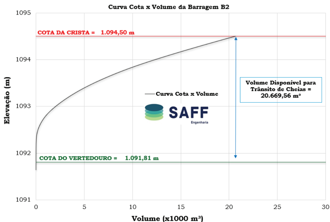
Figura 7.20 - Curva Cota x Volume da Barragem B2 - Mina Tico-Tico.
