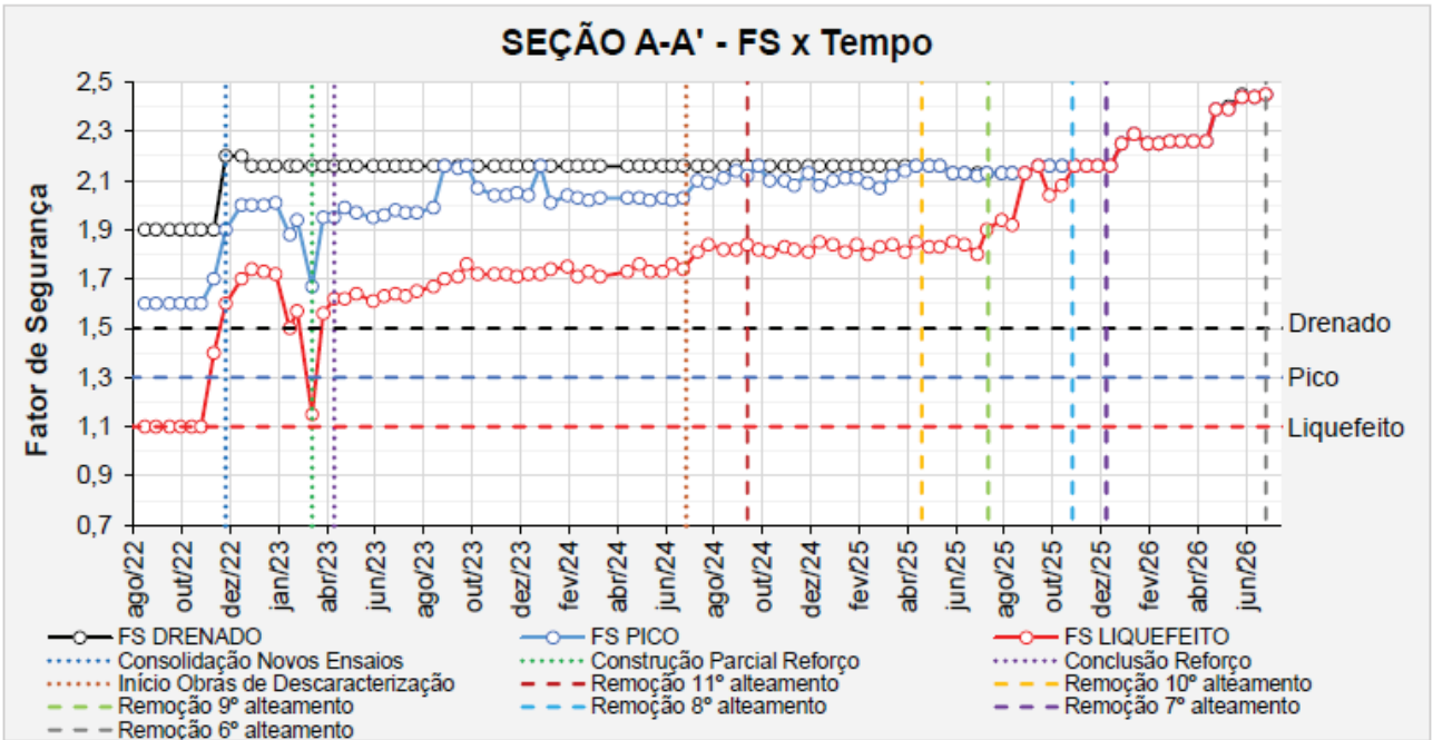
Figura 7.86 – Seção A-A' - Histórico dos F.S. obtidos nas análises de estabilidade.
