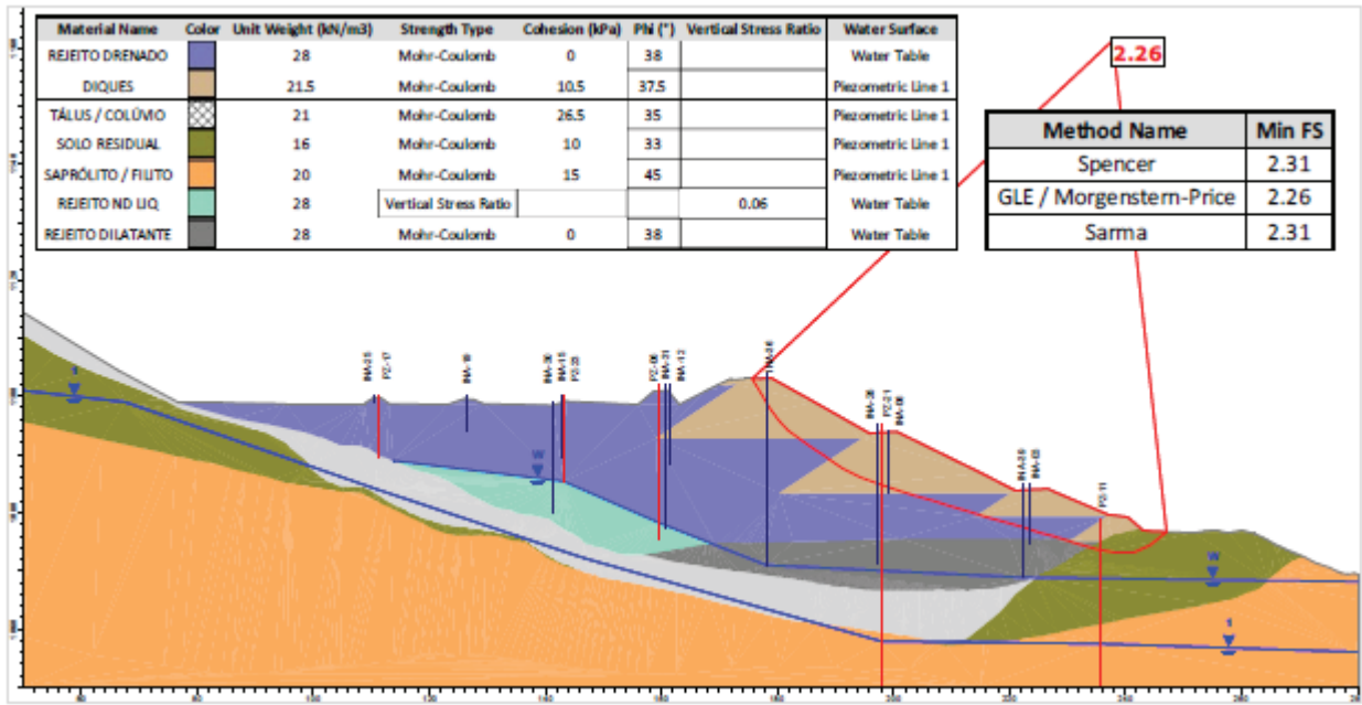
Figura 7.28 – Seção A-A’ – Análise Não Drenada – Superfície de ruptura plano-circular otimizada - Freática atual (28/02/2026) – Razão de resistência não drenada liquefeita. – RISR – Março/2026.
