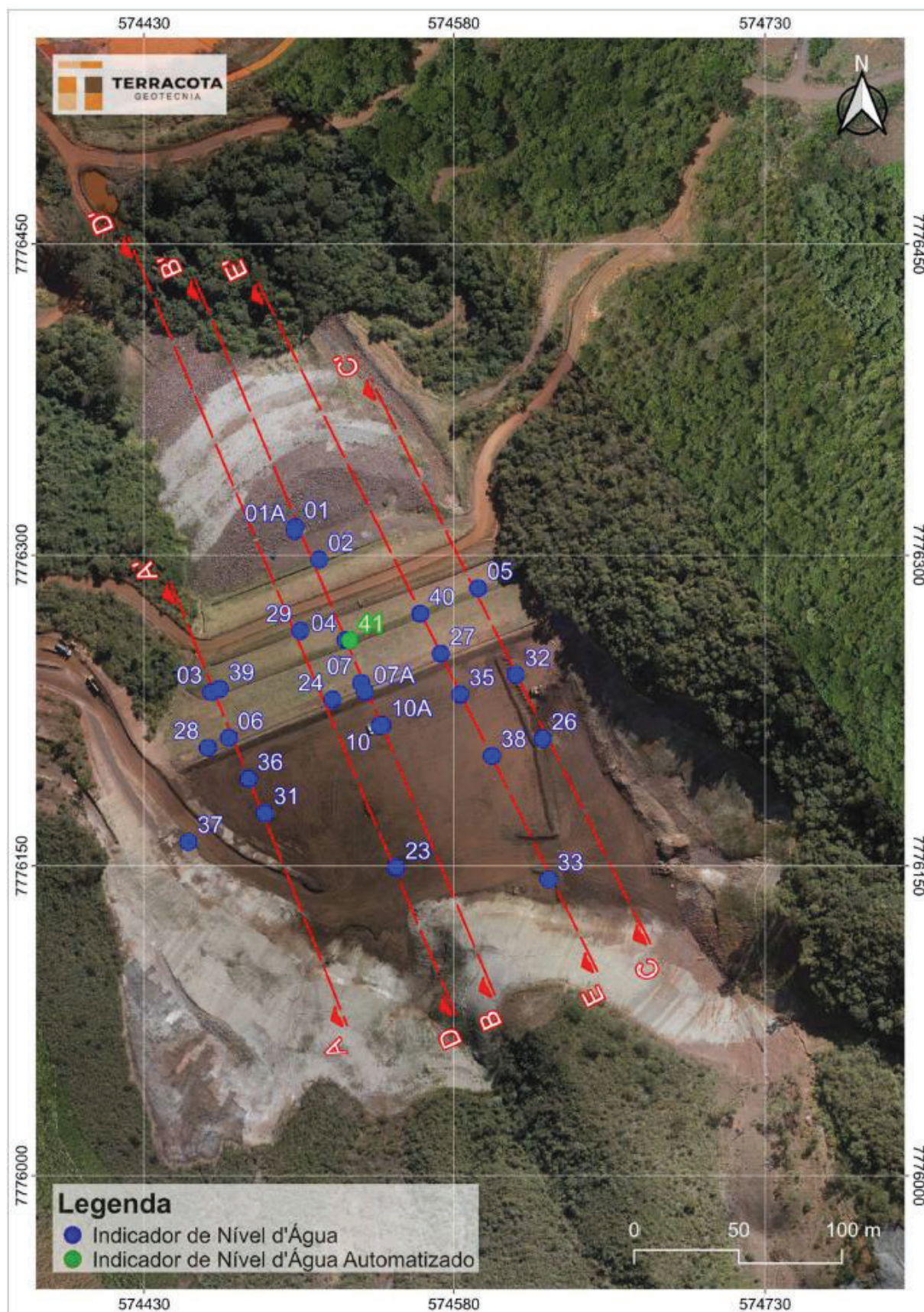
Figura 7.1 – Localização dos indicadores de nível d'água.
