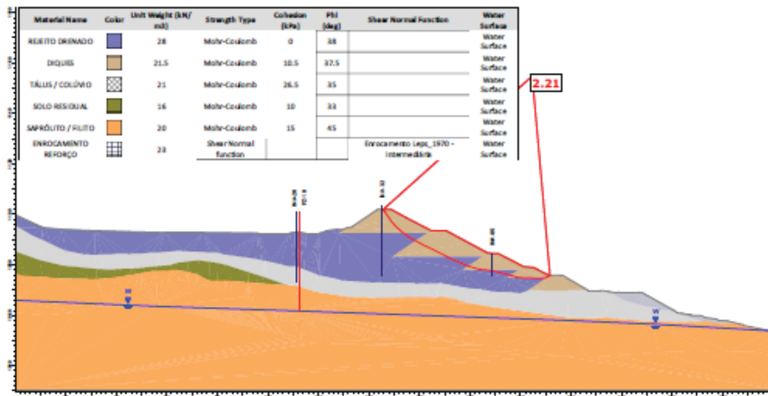
Figura 7.55 - Seção C-C' – Análise Drenada – Superfície de ruptura plano-circular otimizada – Freática atual (27/04/2026).
