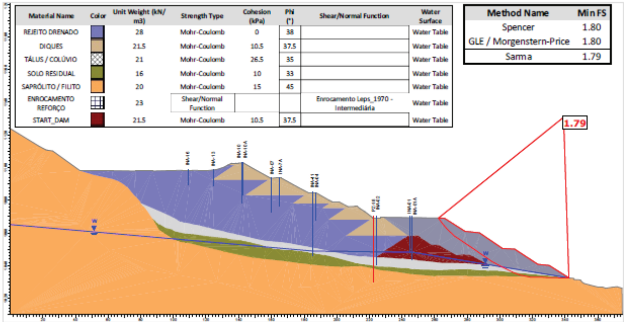
Figura 7.31 – Seção B-B’ – Análise Drenada – Superfície de ruptura plano-circular otimizada – Freática atual (28/02/2026). – RISR – Março/2026.
