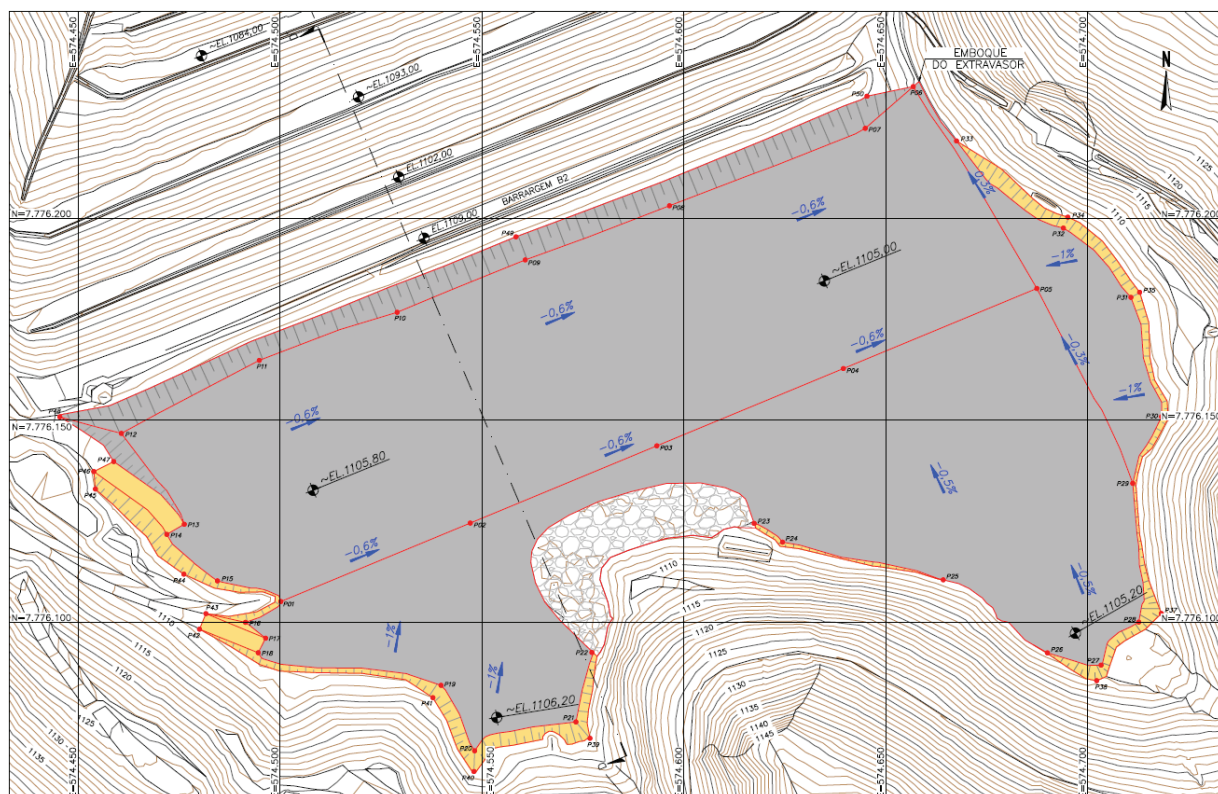
Figura 6.17 - Escavações complementares - Planta (Fonte: IPE.OP.DE.8000.GT.20.1414).
