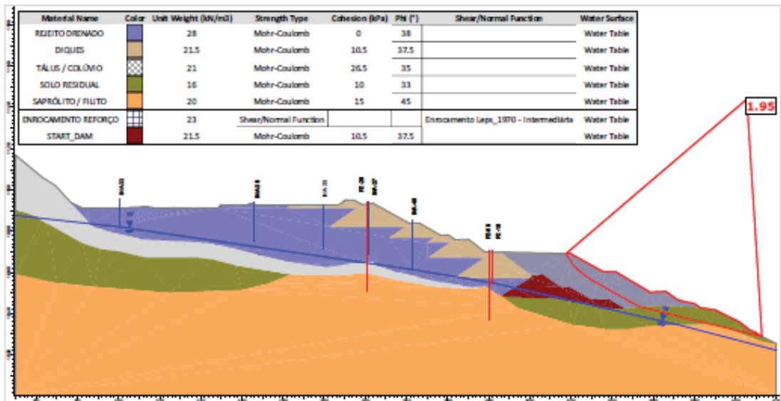
Figura 7.72 - Seção E-E' – Análise Drenada – Superfície de ruptura plano-circular otimizada – Freática atual (30/05/2026).
