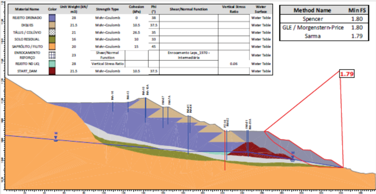
Figura 7.33 – Seção B-B’ – Análise Não Drenada – Superfície de ruptura plano-circular otimizada - Freática atual (28/02/2026) – Razão de resistência não drenada liquefeita. – RISR – Março/2026.
