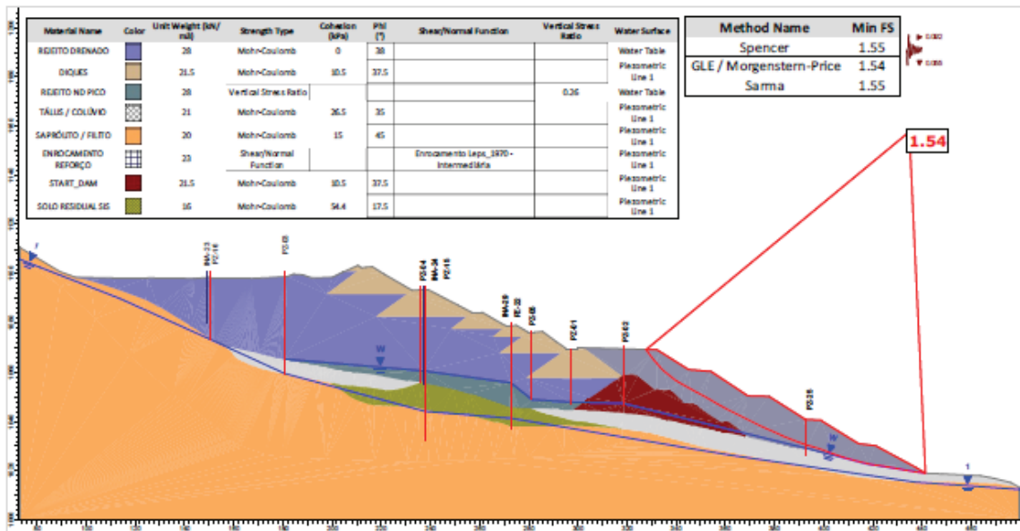
Figura 7.43 – Seção D-D’ – Análise Não Drenada – Superfície de ruptura plano-circular otimizada – Freática atual (28/02/2026) – Razão de resistência não drenada de pico + sismo \downarrow . – RISR – Março/2026.
