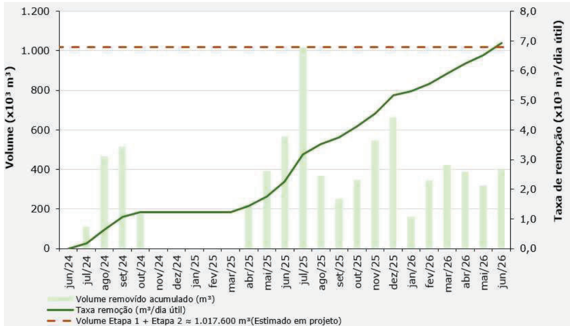
Figura 6.16 – Volume acumulado e taxa de remoção diária da obra de Descaracterização da Barragem B2 – Mina Tico-Tico.
