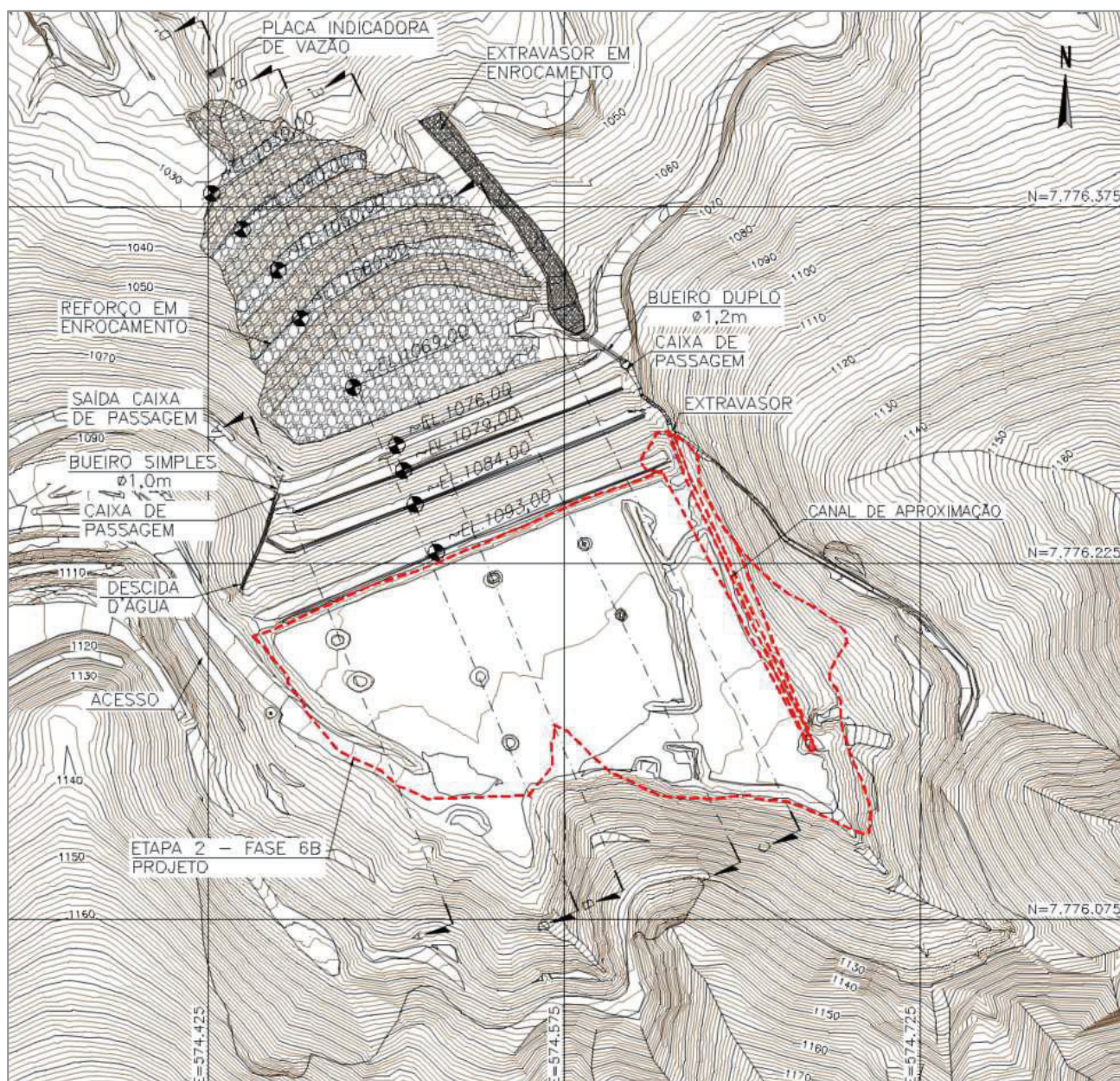
Figura 6.8 – Comparativo Projeto (Etapa 2 - Fase 6B) x Executado – Planta.
