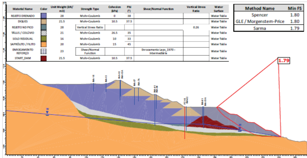
Figura 7.32 – Seção B-B’ – Análise Não Drenada – Superfície de ruptura plano-circular otimizada – Freática atual (28/02/2026) – Razão de resistência não drenada de pico. – RISR – Março/2026.
