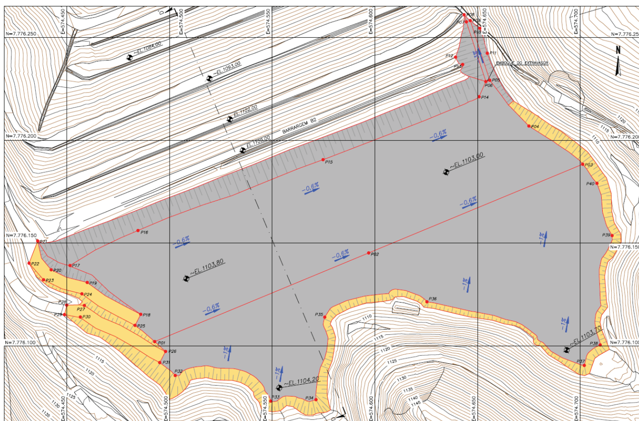
Figura 6.19 – Escavações complementares - Planta (Fonte: IPE.OP.DE.8000.GT.20.1415).
