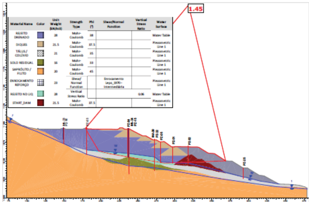
Figura 7.71 - Seção D-D' – Análise Não Drenada – Superfície de ruptura plano-circular otimizada - Freática atual (30/05/2026) – Razão de resistência não drenada liquefeita.
