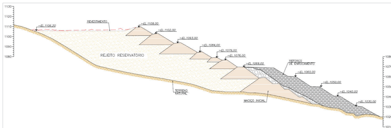
Figura 6.18 - Escavações complementares – Seção Transversal D-D'. (Fonte: IPE.OP.DE.8000.GT.20. 1414).
