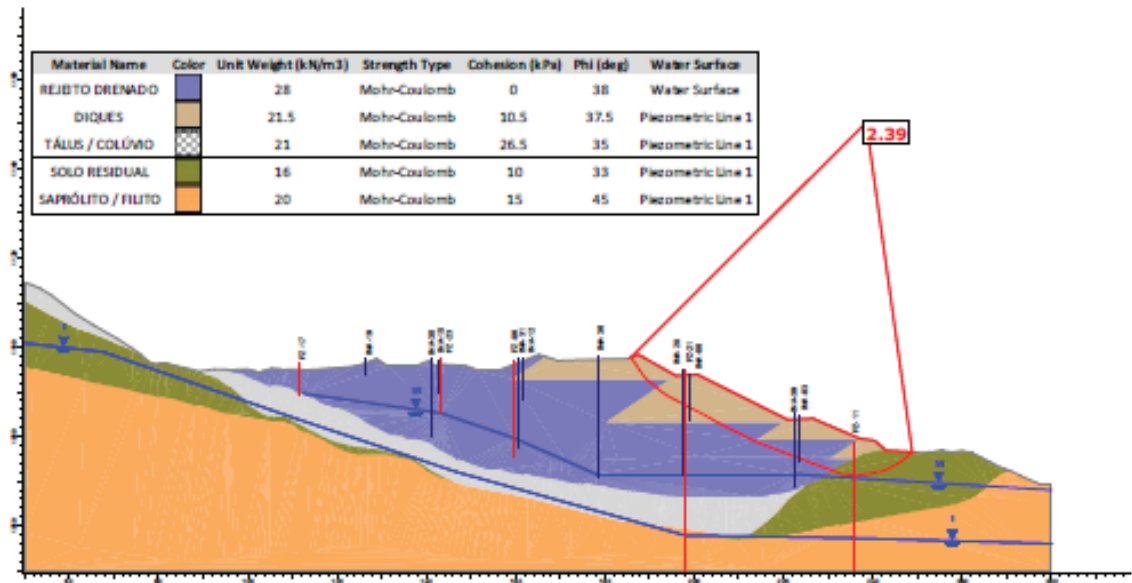
Figura 7.49 - Seção A-A' – Análise Drenada – Superfície de ruptura plano-circular otimizada – Freática atual (27/04/2026).
