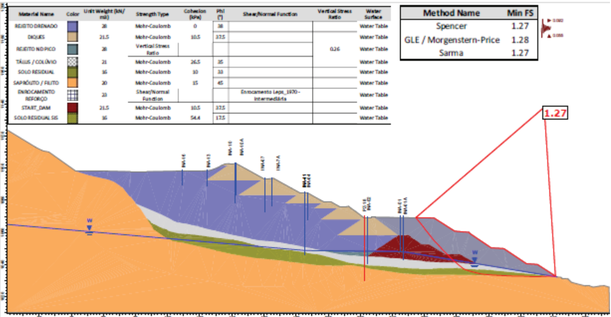
Figura 7.34 – Seção B-B’ – Análise Não Drenada – Superfície de ruptura plano-circular otimizada – Freática atual (28/02/2026) – Razão de resistência não drenada de pico + sismo ↑. – RISR – Março/2026.
