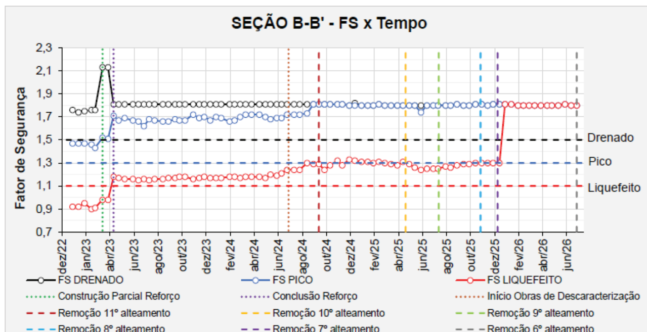
Figura 7.87 – Seção B-B' - Histórico dos F.S. obtidos nas análises de estabilidade.
