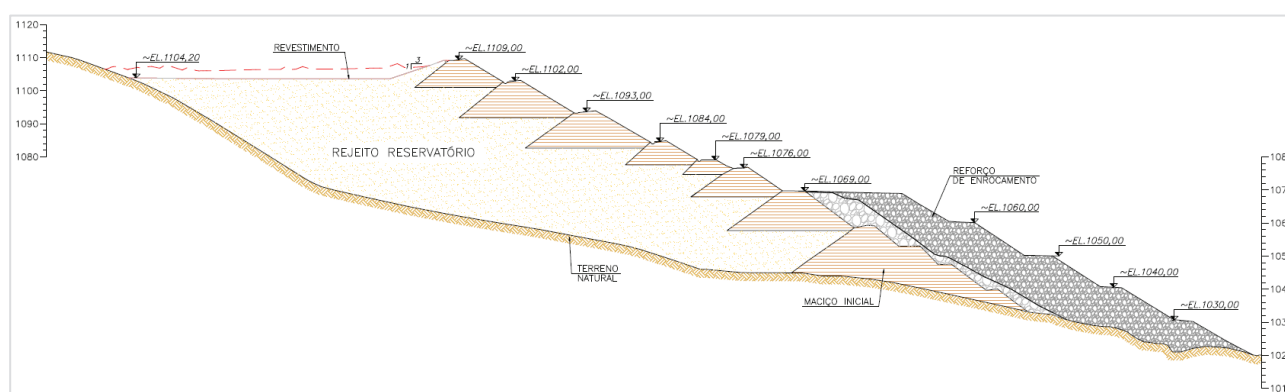
Figura 6.20 – Escavações complementares – Seção Transversal D-D' (Fonte: IPE.OP.DE.8000.GT.20.1415).
