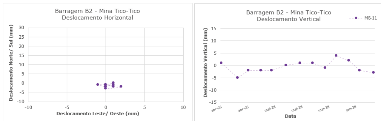
Figura 7.14 – Marco de controle de deformação – MS-11.
