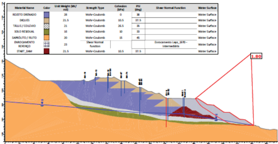
Figura 7.52 - Seção B-B' – Análise Drenada – Superfície de ruptura plano-circular otimizada – Freática atual (27/04/2026).
