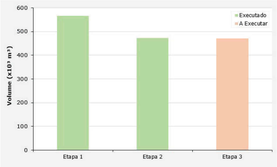
Figura 6.15 – Avanço das obras de Descaracterização da Barragem B2 – Mina Tico-Tico.
