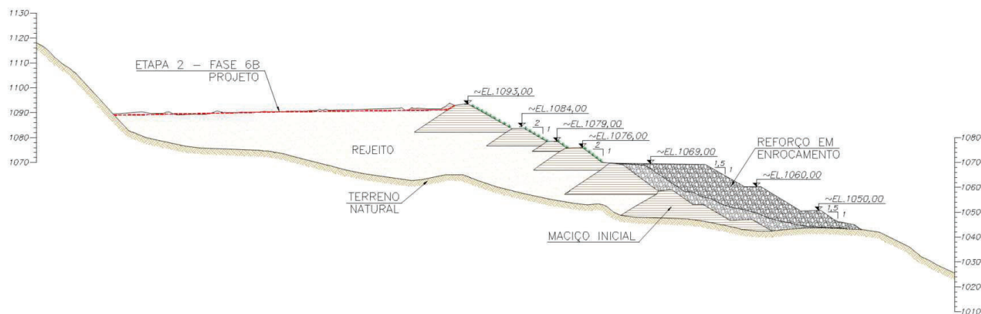
Figura 6.13 – Comparativo Projeto (Etapa 2 - Fase 6A) x Executado – Seção E-E’.
