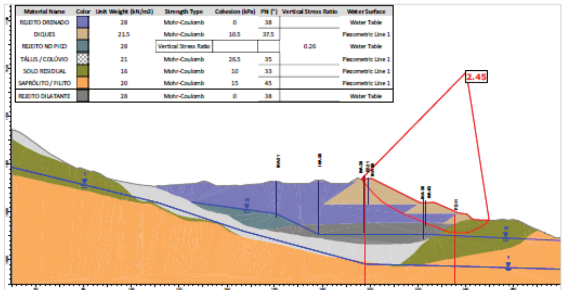
Figura 7.76 - Seção A-A' – Análise Não Drenada – Superfície de ruptura plano-circular otimizada - Freática atual (29/06/2026) – Razão de resistência não drenada de pico.
