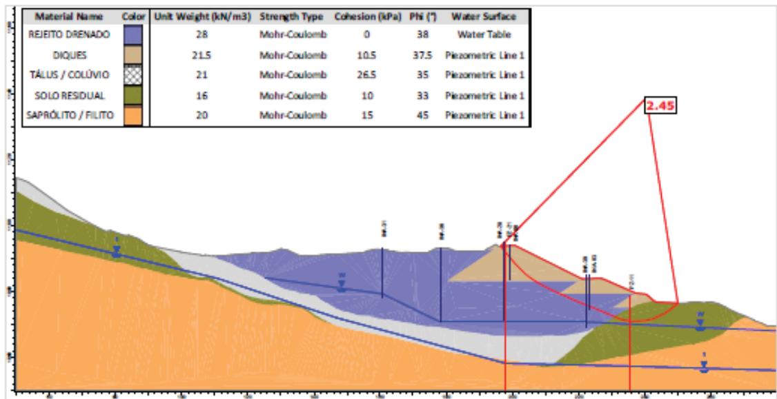
Figura 7.75 - Seção A-A' – Análise Drenada – Superfície de ruptura plano-circular otimizada – Freática atual (29/06/2026).
