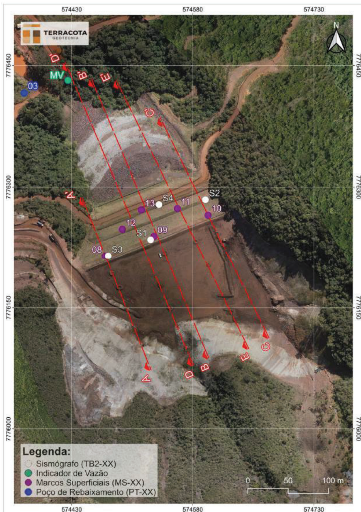
Figura 7.3 – Localização dos marcos superficiais, sismógrafos, indicador de vazão e poço de rebaixamento.
