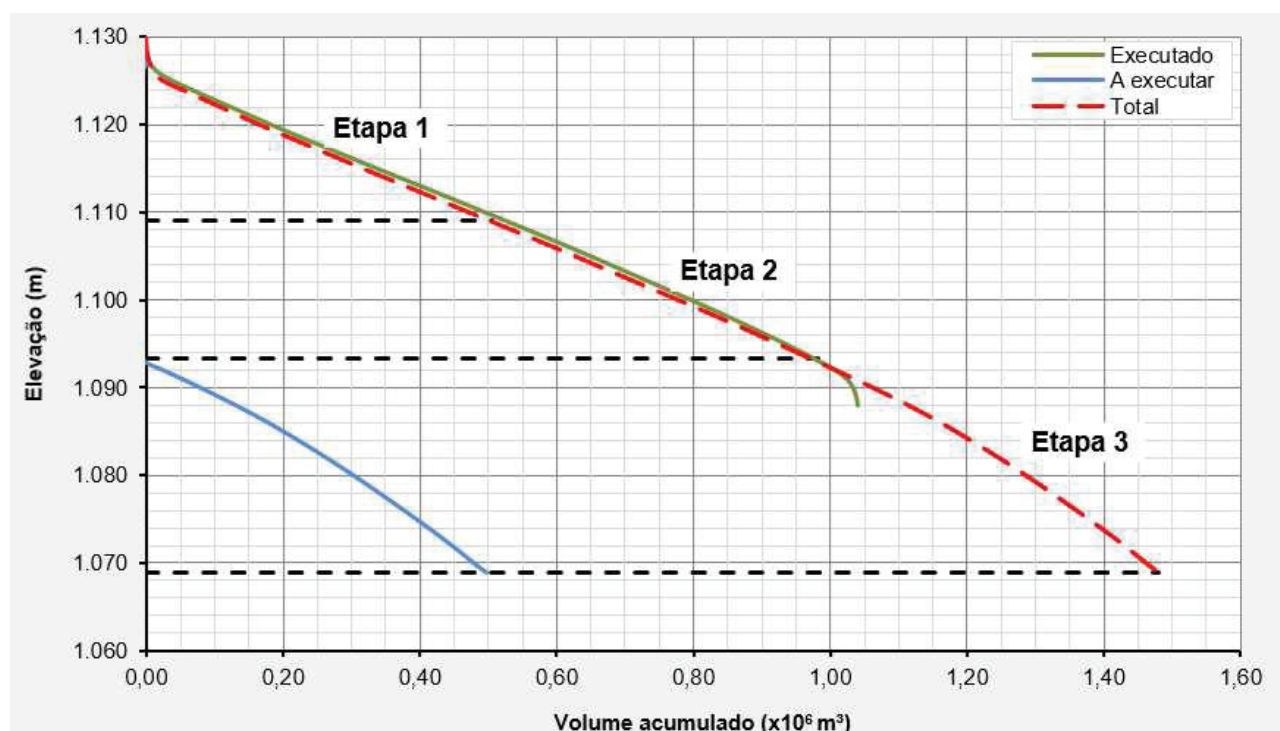
Figura 6.14 – Curva elevação-volume – Comparativo andamento das obras.
