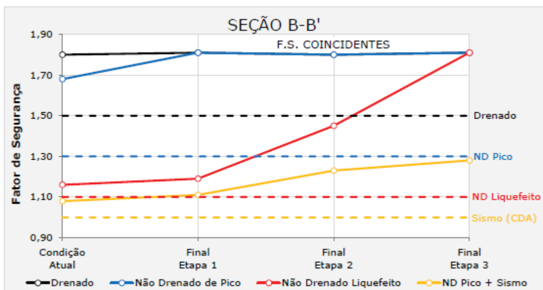
Figura 7.92 - Seção B-B' – Projeção da evolução dos fatores de segurança durante obra.
