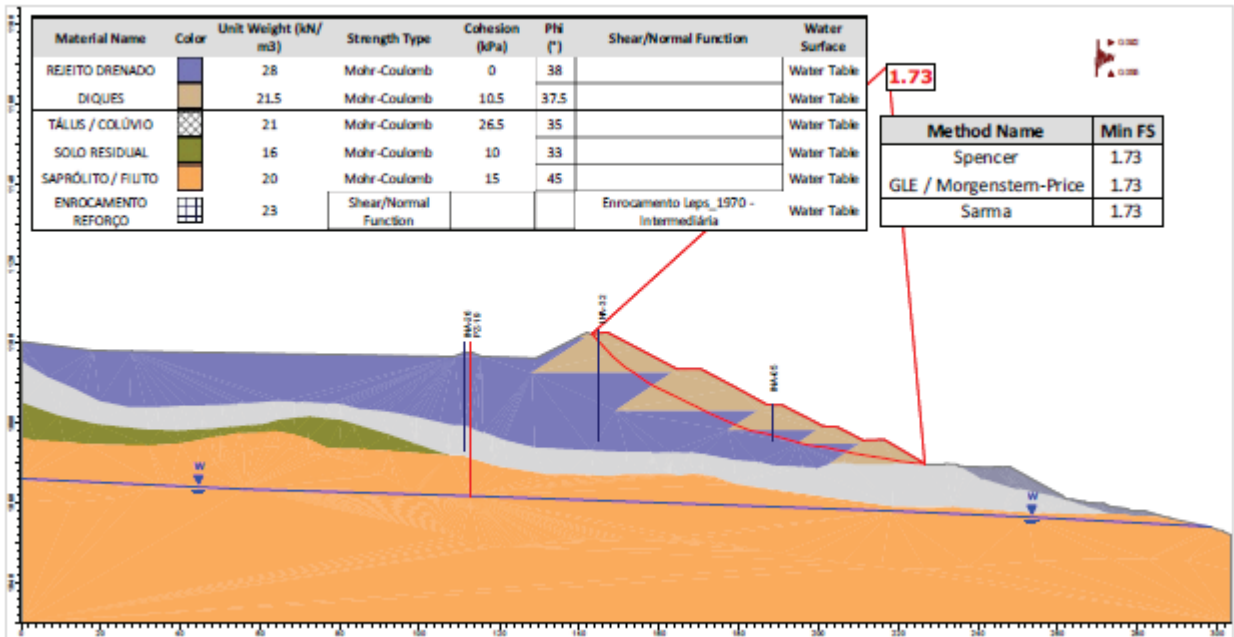
Figura 7.37 – Seção C-C’ – Análise Drenada – Superfície de ruptura plano-circular otimizada – Freática atual (28/02/2026) – Carregamento Sísmico ↑. – RISR – Março/2026.
