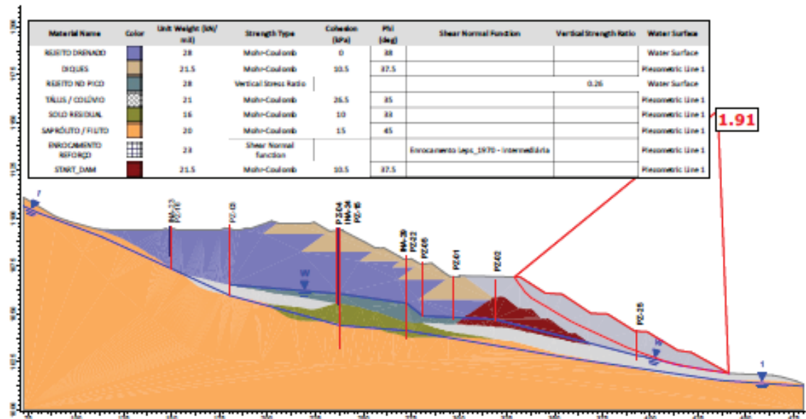
Figura 7.57 - Seção D-D' – Análise Não Drenada – Superfície de ruptura plano-circular otimizada - Freática atual (27/04/2026) – Razão de resistência não drenada de pico.
