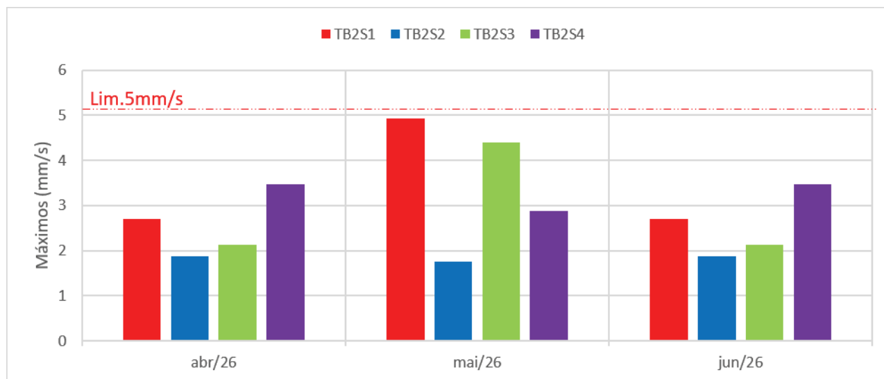
Figura 7.18 - Evolução das amplitudes máximas (mm/s).
