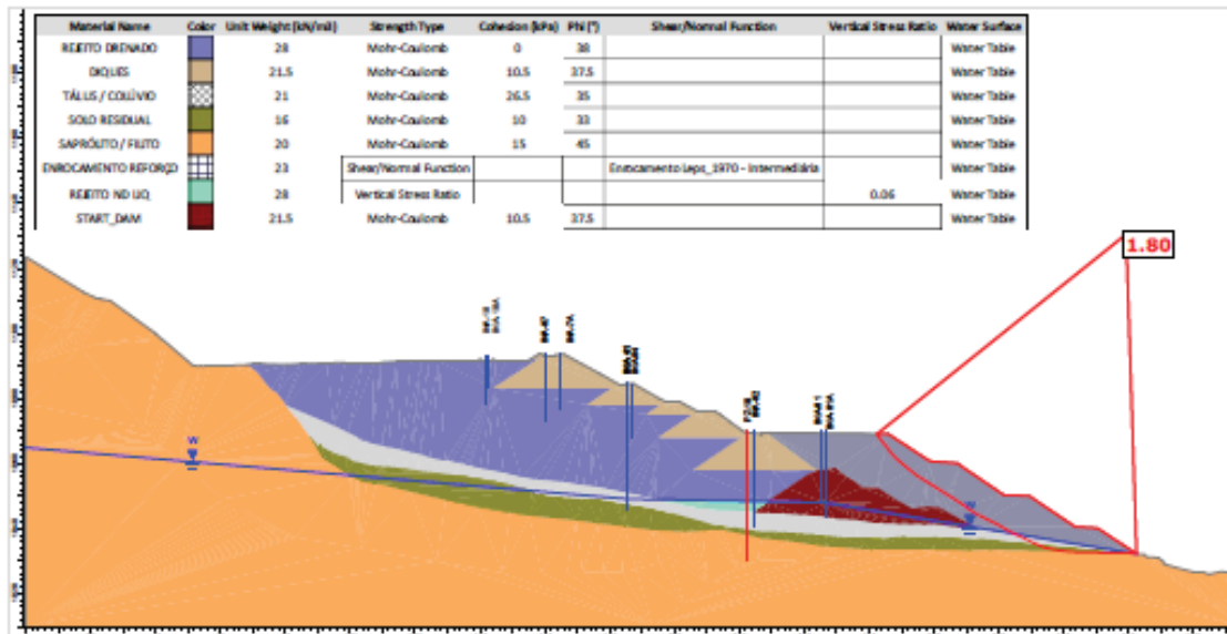
Figura 7.80 - Seção B-B' – Análise Não Drenada – Superfície de ruptura plano-circular otimizada - Freática atual (29/06/2026) – Razão de resistência não drenada liquefeita.
