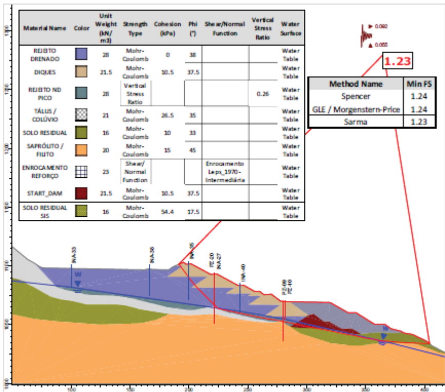
Figura 7.47 – Seção E-E’ – Análise Não Drenada – Superfície de ruptura plano-circular otimizada – Freática atual (28/02/2026) – Razão de resistência não drenada de pico + sismo ↑. – RISR – Março/2026.
