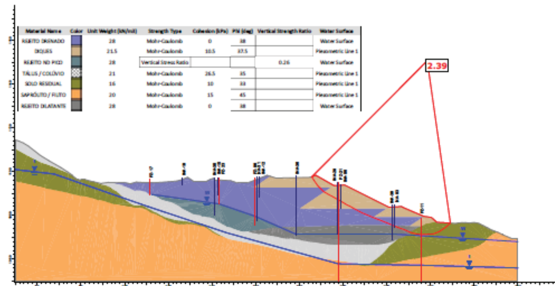
Figura 7.50 - Seção A-A' – Análise Não Drenada – Superfície de ruptura plano-circular otimizada - Freática atual (27/04/2026) – Razão de resistência não drenada de pico.
