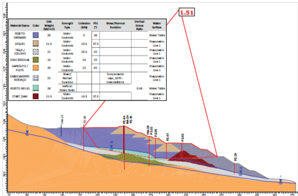
Figura 7.84 - Seção D-D' – Análise Não Drenada – Superfície de ruptura plano-circular otimizada - Freática atual (29/06/2026) – Razão de resistência não drenada liquefeita.
