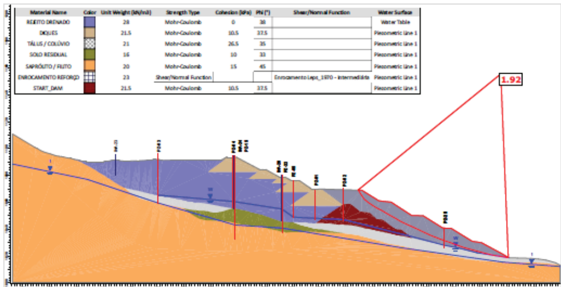
Figura 7.82 - Seção D-D' – Análise Drenada – Superfície de ruptura plano-circular otimizada – Freática atual (29/06/2026).
