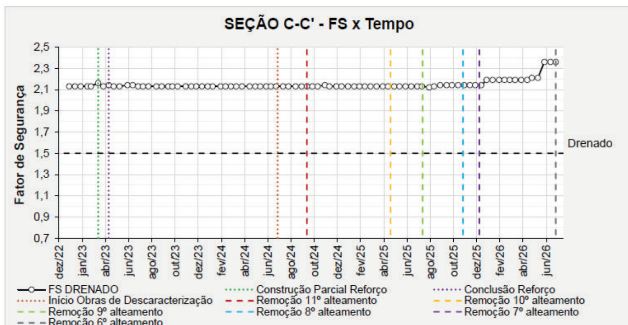
Figura 7.88 – Seção C-C' - Histórico dos F.S. obtidos nas análises de estabilidade.
