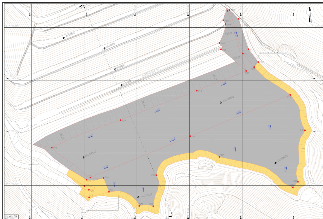
Figura 7.96 – Escavação e direcionamento de drenagem do reservatório.
