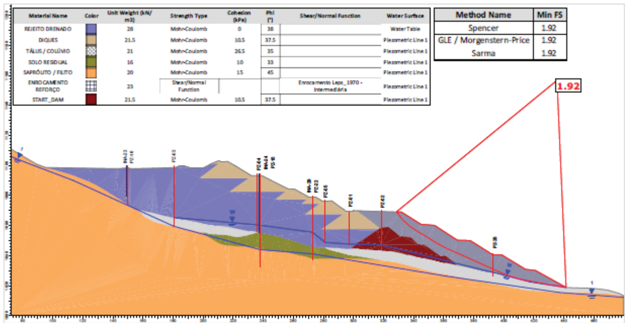
Figura 7.39 – Seção D-D’ – Análise Drenada – Superfície de ruptura plano-circular otimizada – Freática atual (28/02/2026). – RISR – Março/2026.
