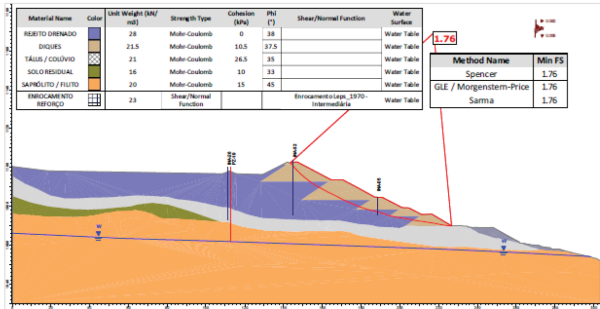
Figura 7.38 – Seção C-C’ – Análise Drenada – Superfície de ruptura plano-circular otimizada – Freática atual (28/02/2026) – Carregamento Sísmico ↓. – RISR – Março/2026.
