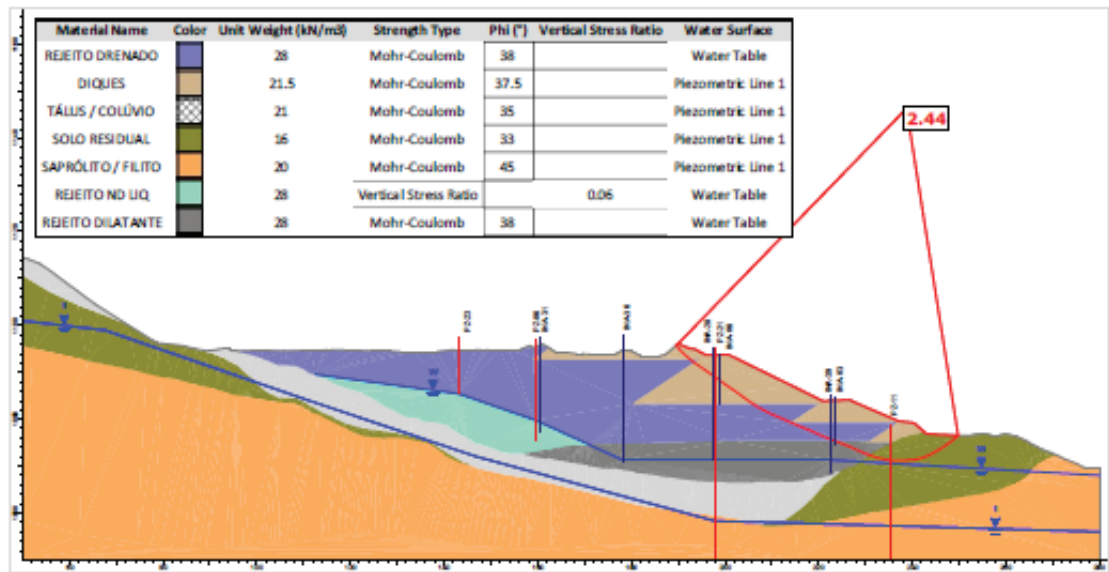
Figura 7.64 - Seção A-A' – Análise Não Drenada – Superfície de ruptura plano-circular otimizada - Freática atual (30/05/2026) – Razão de resistência não drenada liquefeita.
