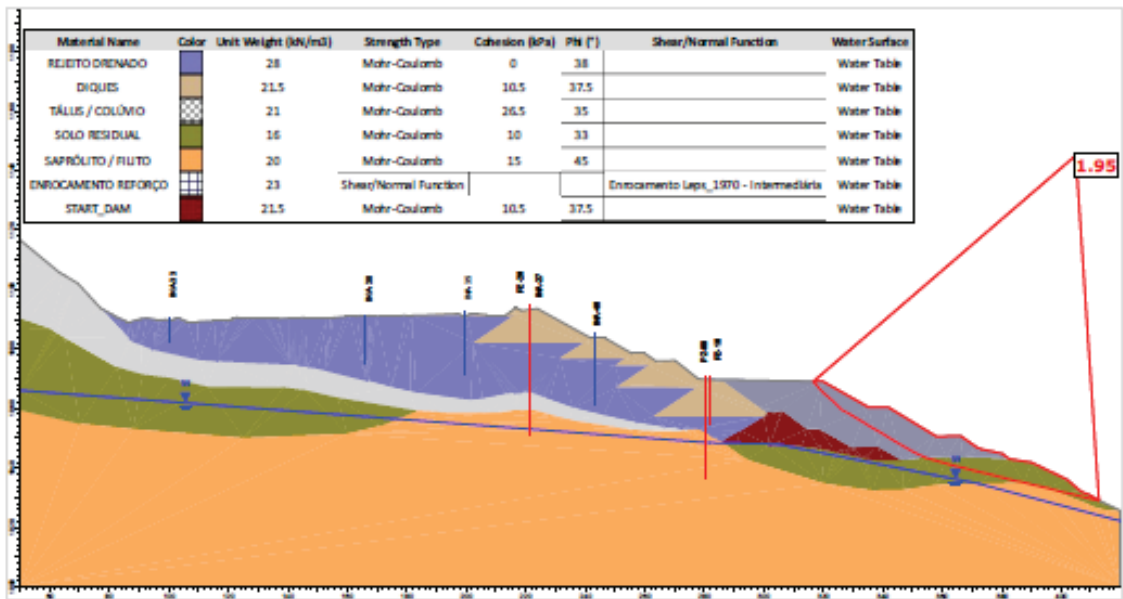
Figura 7.85 - Seção E-E' – Análise Drenada – Superfície de ruptura plano-circular otimizada – Freática atual (29/06/2026).
