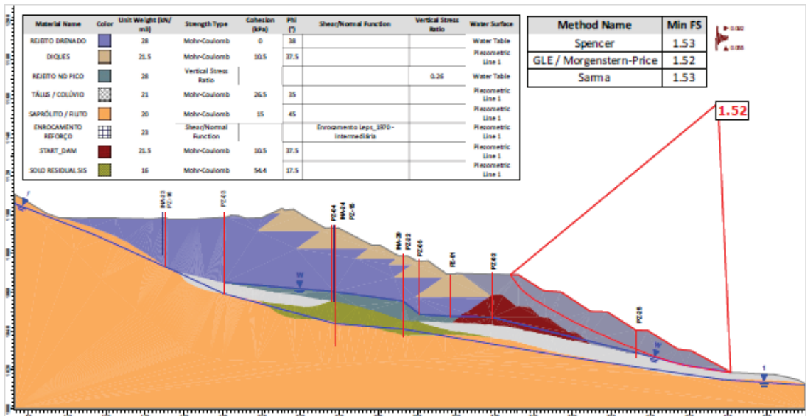
Figura 7.42 – Seção D-D’ – Análise Não Drenada – Superfície de ruptura plano-circular otimizada – Freática atual (28/02/2026) – Razão de resistência não drenada de pico + sismo ↑. – RISR – Março/2026.
