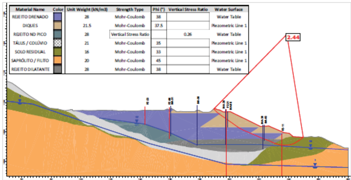
Figura 7.63 - Seção A-A' – Análise Não Drenada – Superfície de ruptura plano-circular otimizada - Freática atual (30/05/2026) – Razão de resistência não drenada de pico.
