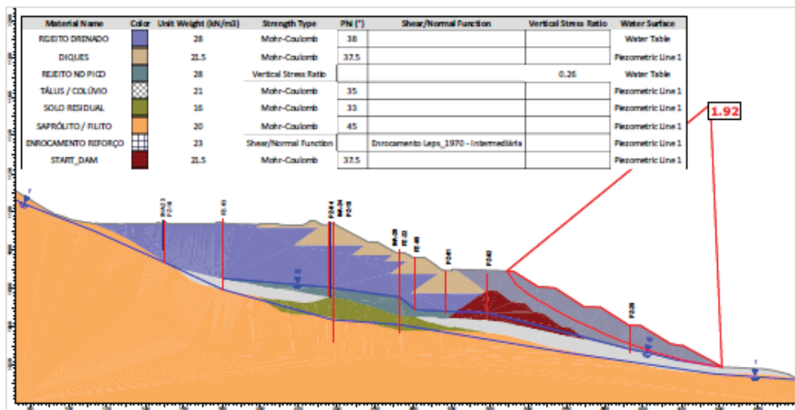
Figura 7.70 - Seção D-D' – Análise Não Drenada – Superfície de ruptura plano-circular otimizada - Freática atual (30/05/2026) – Razão de resistência não drenada de pico.
