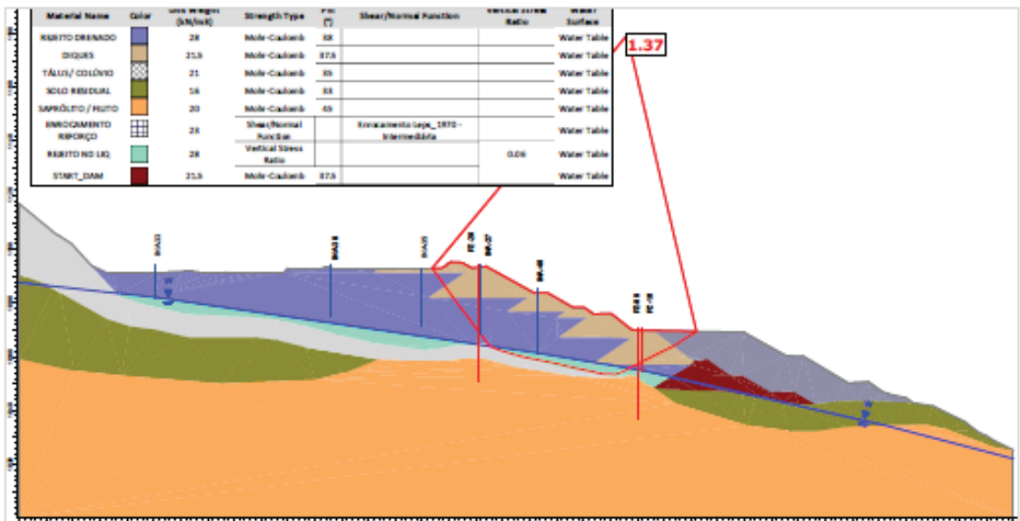
Figura 7.74 - Seção E-E' – Análise Não Drenada – Superfície de ruptura plano-circular otimizada - Freática atual (30/05/2026) – Razão de resistência não drenada liquefeita.
