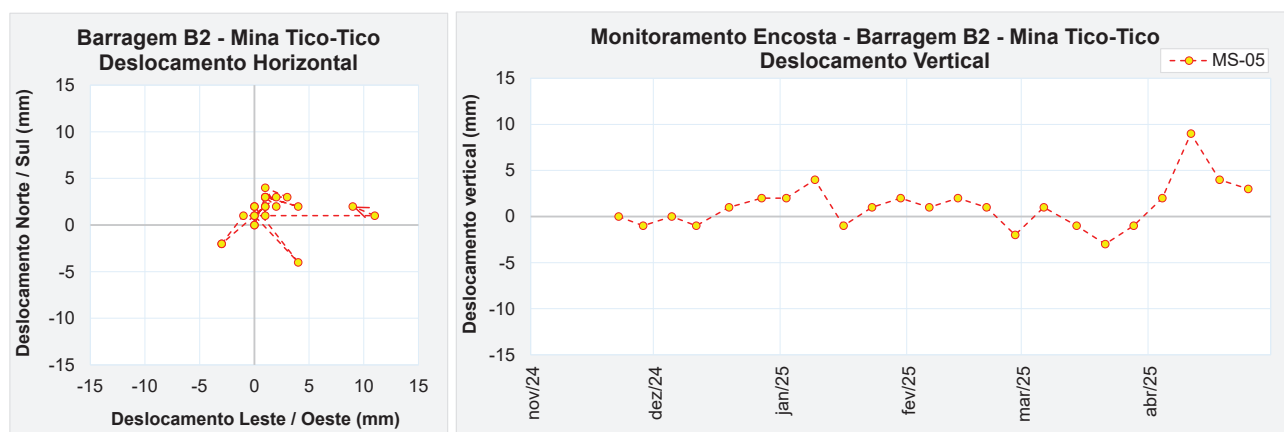
Figura 5.16 – Histórico do Marco de controle de monitoramento da encosta – MS-05.
