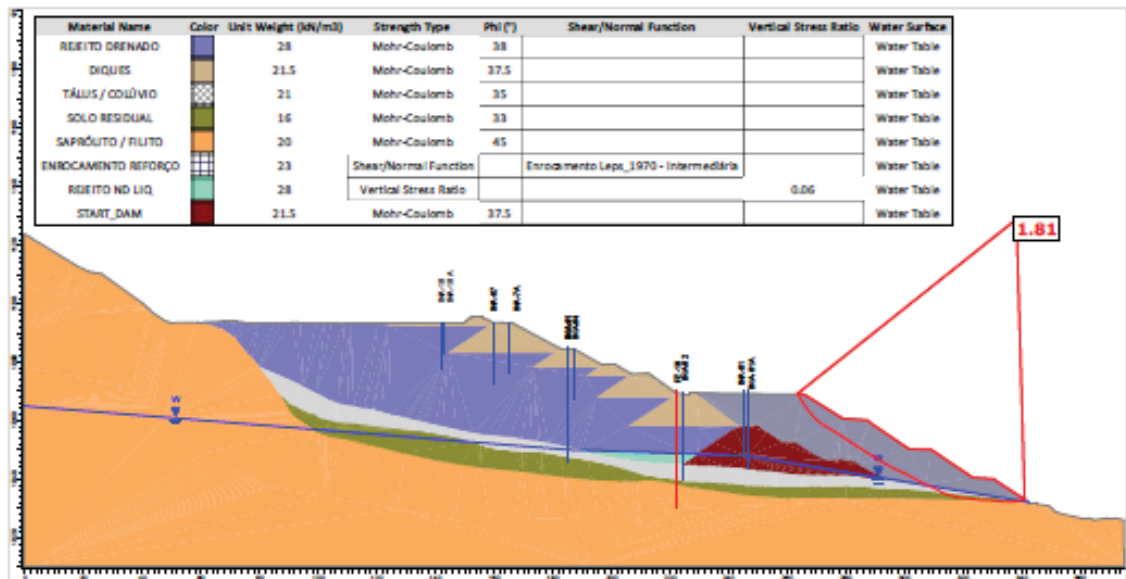
Figura 7.67 - Seção B-B' – Análise Não Drenada – Superfície de ruptura plano-circular otimizada - Freática atual (30/05/2026) – Razão de resistência não drenada liquefeita.
