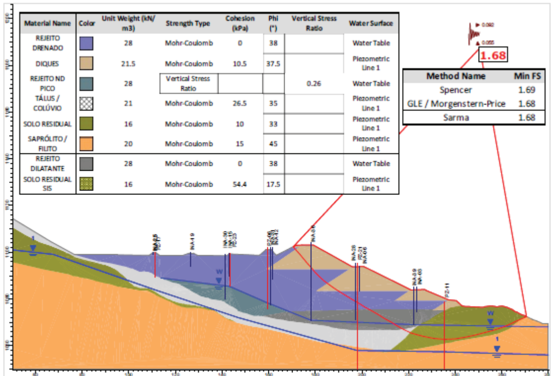
Figura 7.29 – Seção A-A’ – Análise Não Drenada – Superfície de ruptura plano-circular otimizada – Freática atual (28/02/2026) – Razão de resistência não drenada de pico + sismo ↑. – RISR – Março/2026.
