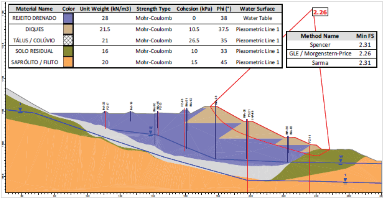
Figura 7.26 – Seção A-A’ – Análise Drenada – Superfície de ruptura plano-circular otimizada – Freática atual (28/02/2026) – RISR – Março/2026.
