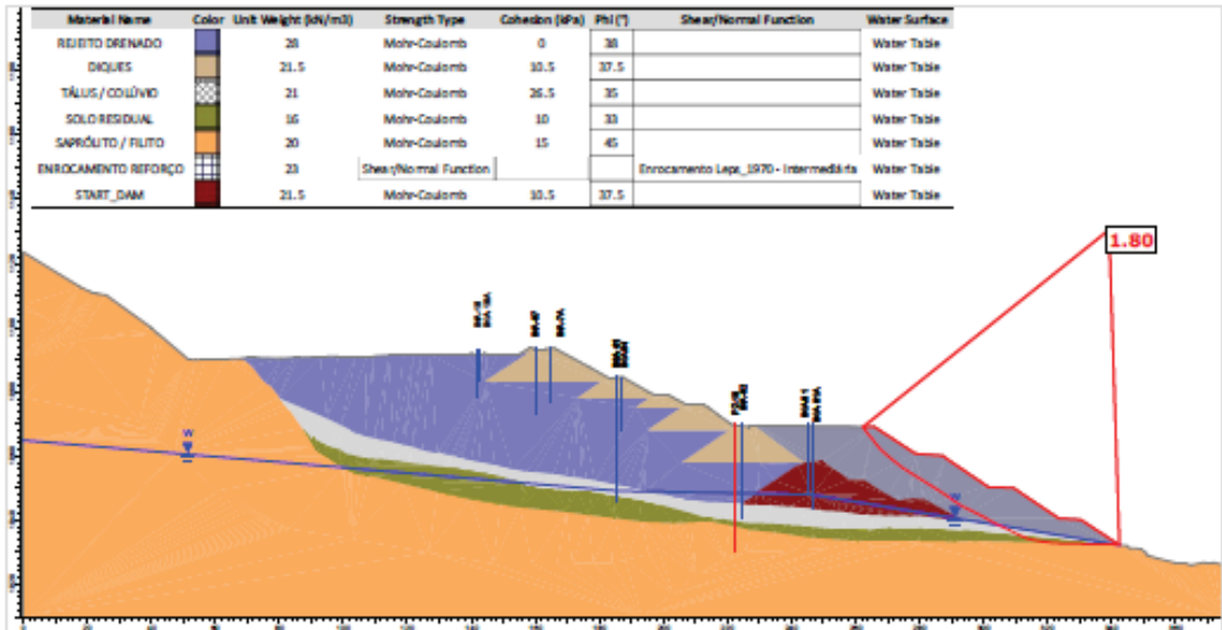
Figura 7.78 - Seção B-B' – Análise Drenada – Superfície de ruptura plano-circular otimizada – Freática atual (29/06/2026).
