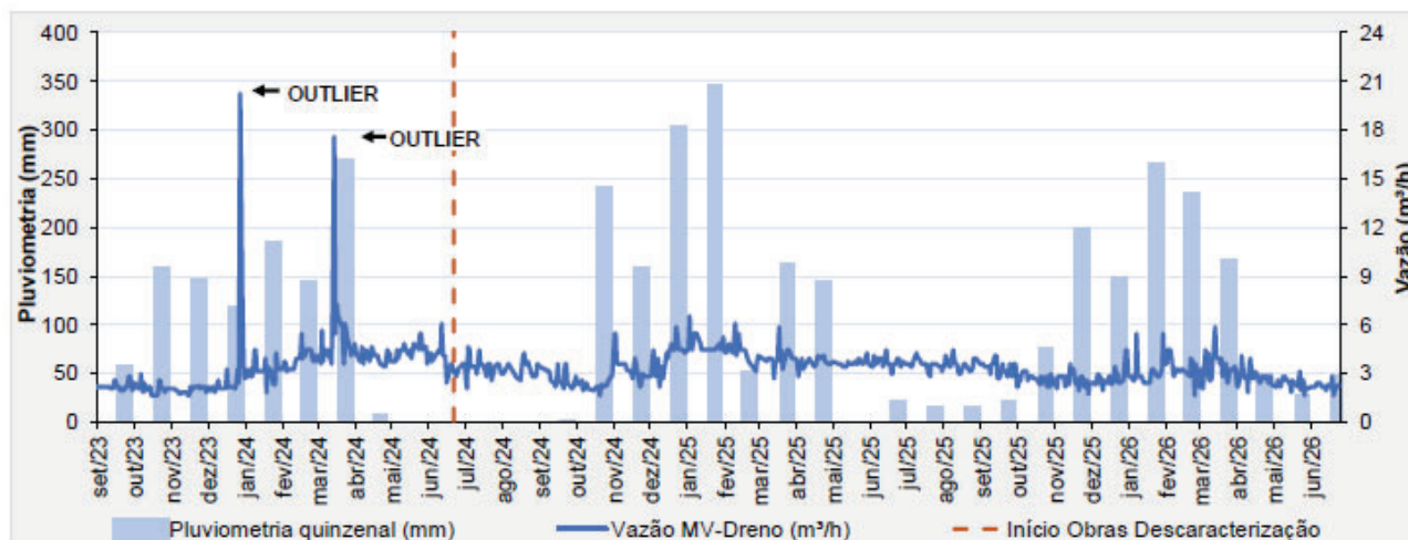
Figura 7.10 – Vazão – MV-Dreno – Barragem B2 – Mina Tico-Tico.
