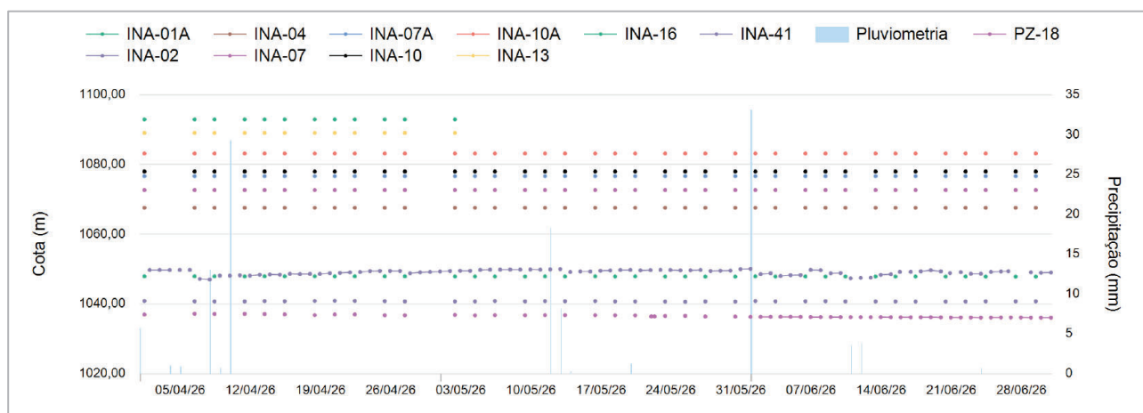
Figura 7.5 – Instrumentos Seção B-B.
