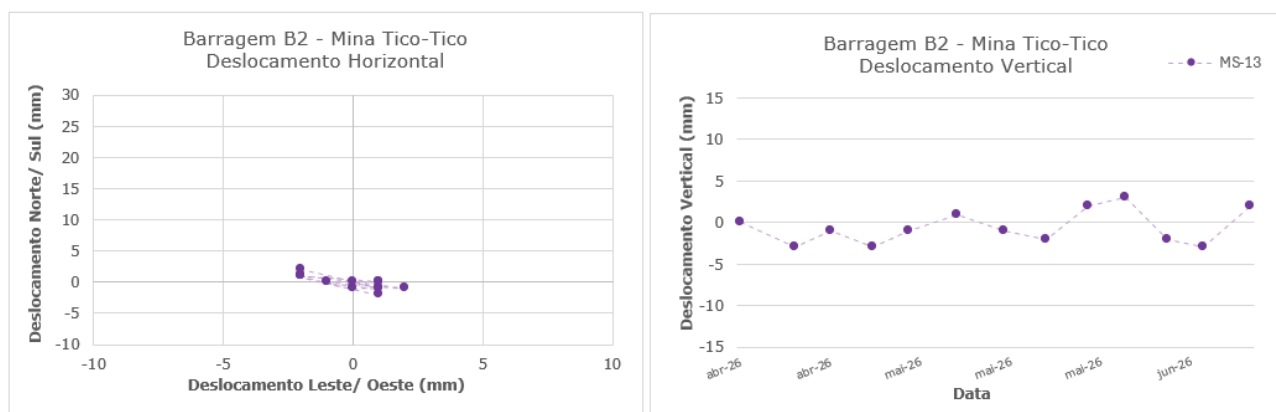
Figura 7.16 – Marco de controle de deformação – MS-13.
