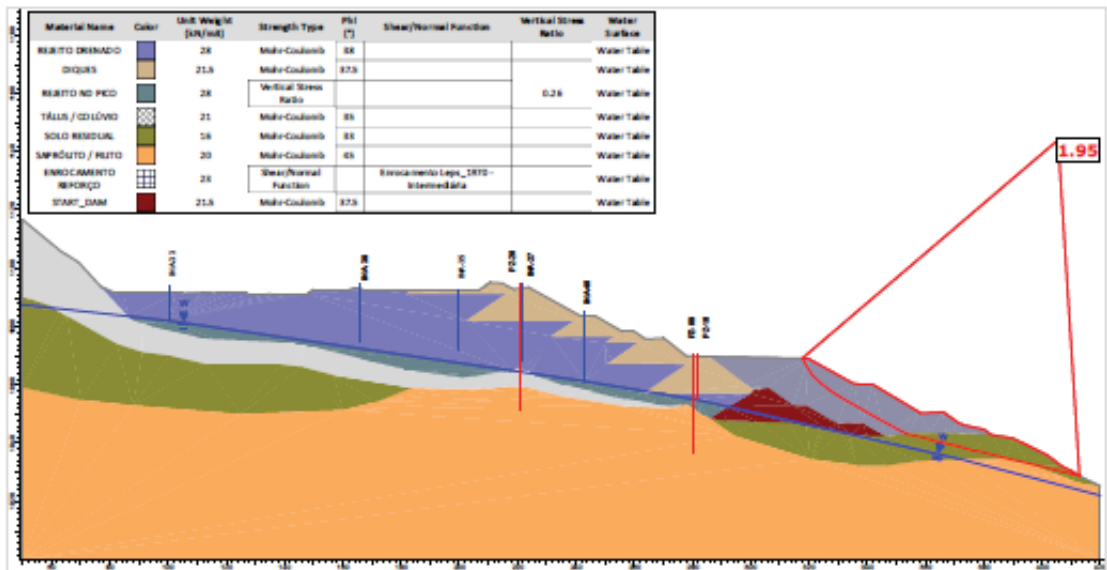
Figura 7.73 - Seção E-E' – Análise Não Drenada – Superfície de ruptura plano-circular otimizada - Freática atual (30/05/2026) – Razão de resistência não drenada de pico.
