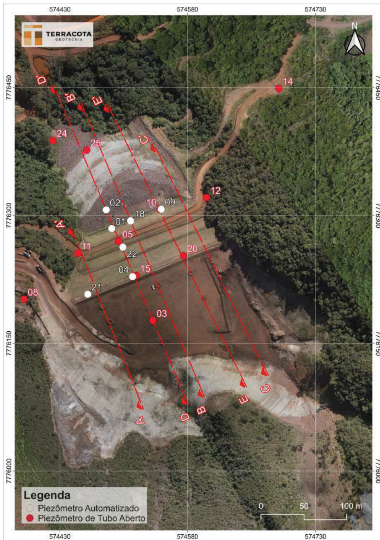
Figura 7.2 – Localização dos piezômetros.
