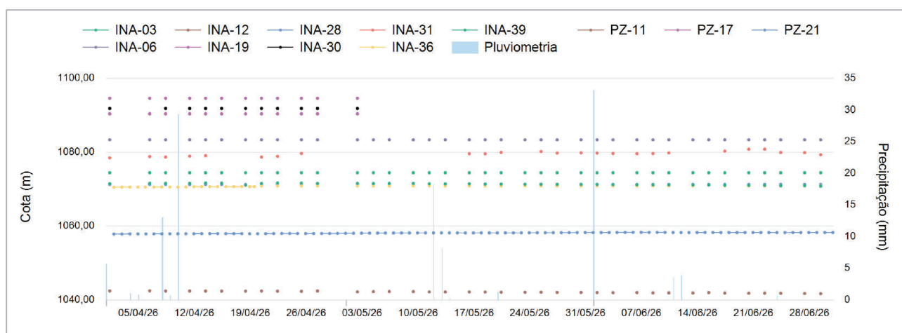
Figura 7.4 - Instrumentos Seção A-A.
