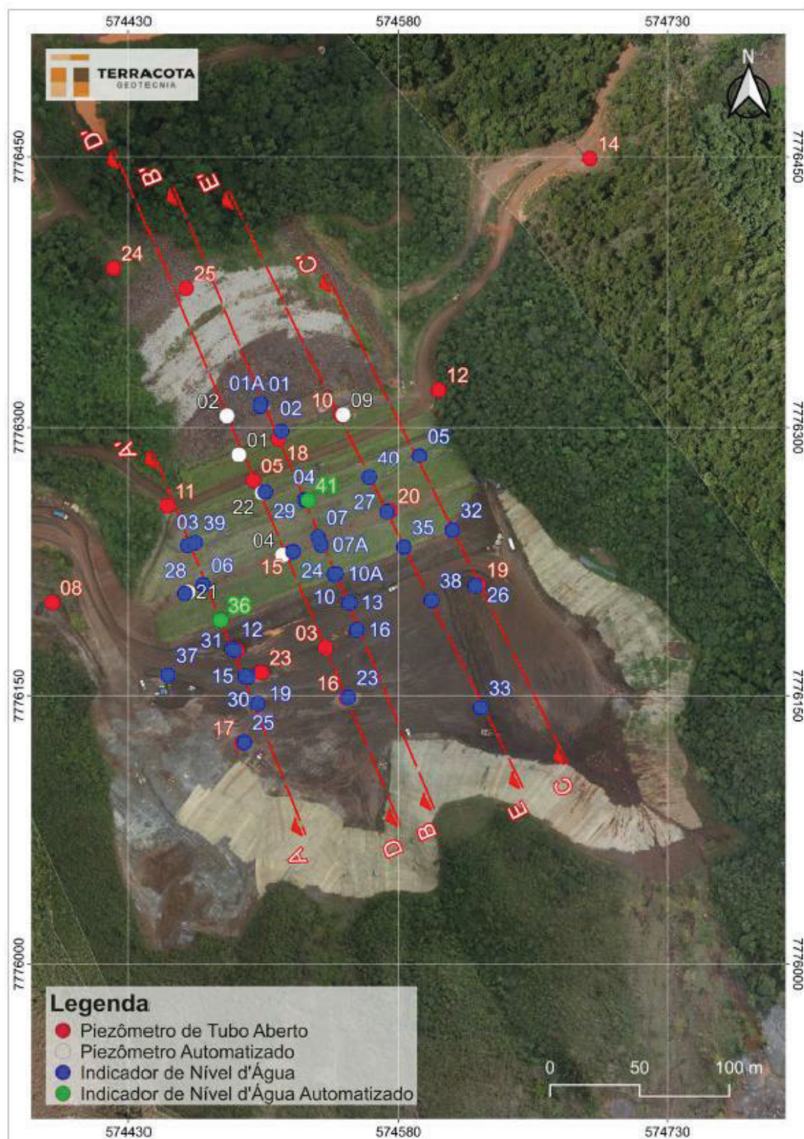
Figura 7.23 – Seções Instrumentadas Barragem B2 – Mina Tico-Tico – Planta (RISR – Março/26).
