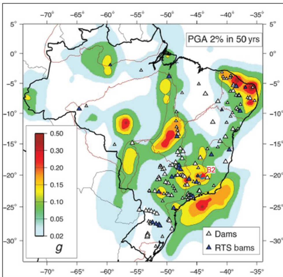
Figura 7.25 – Mapa de Ameaça Sísmica Brasileiro com probabilidade de excedência de 2% durante 50 anos (Assumpção Et al., 2018).
