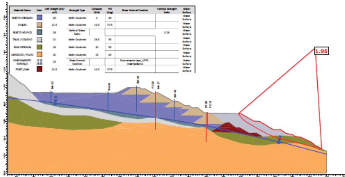
Figura 7.60 - Seção E-E' – Análise Não Drenada – Superfície de ruptura plano-circular otimizada - Freática atual (27/04/2026) – Razão de resistência não drenada de pico.
