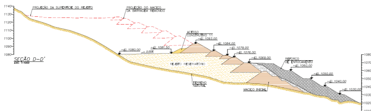
Figura 6.4 - Sequência Construtiva – Seção D-D' – Etapa 3 - Fase 7E - Final (IPE.OP.DE.8000.GT.20.729).
