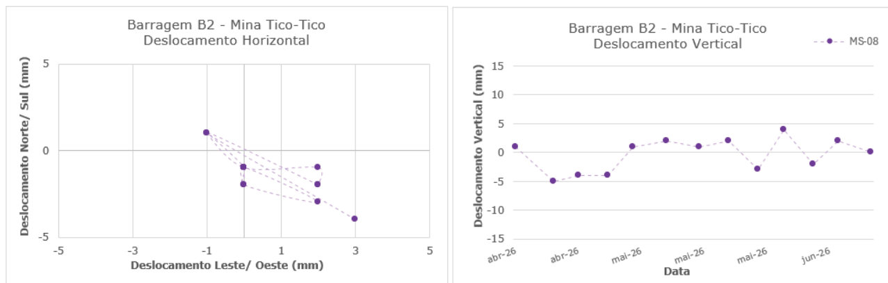
Figura 7.11 – Marco de controle de deformação – MS-08.
